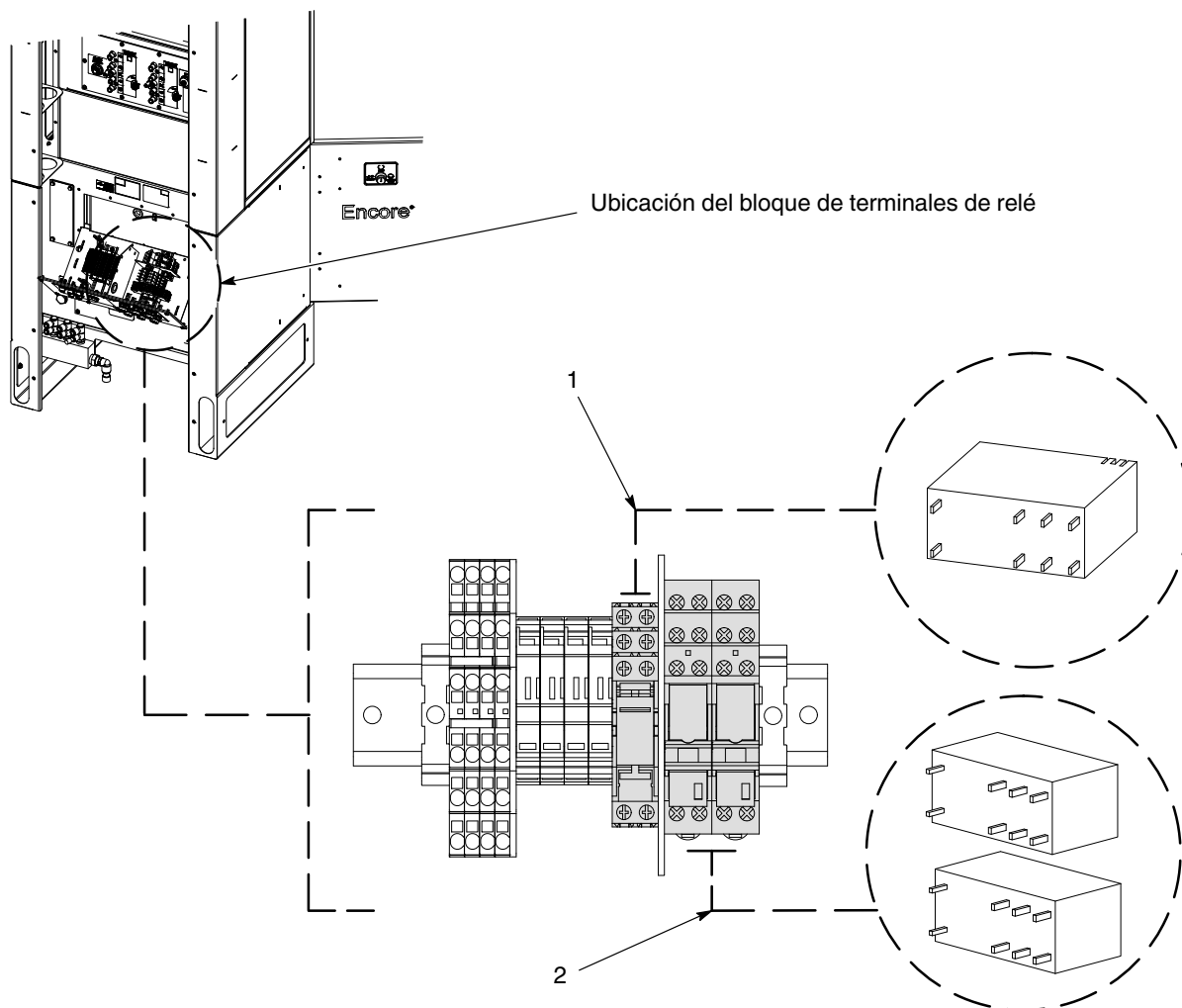
Figura 1 Ubicación del bloque de terminales
