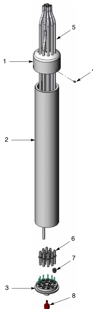
Ábra 2 Szórószár szerelvény javítása és pótalkatrészek
