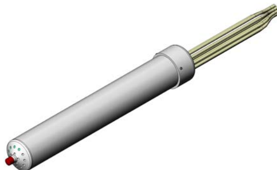
Ábra 1 Prodigy szórószár szerelvény
