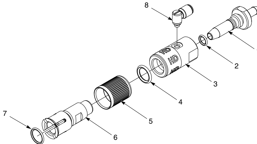
Ábra 1 Encore HD külső diffúzor
