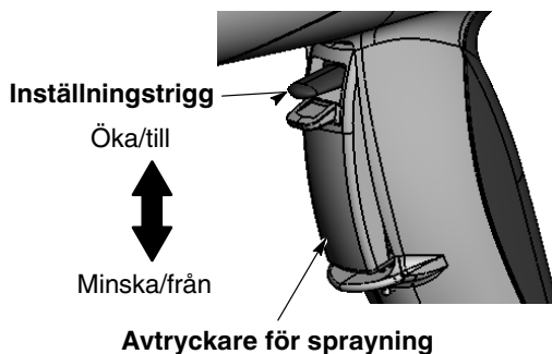
Bild 22 Pistolavtryckarens funktioner
