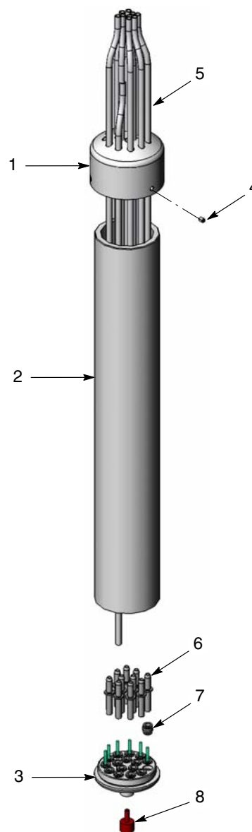
Slika 2 Popravilo in deli sklopa sulice
