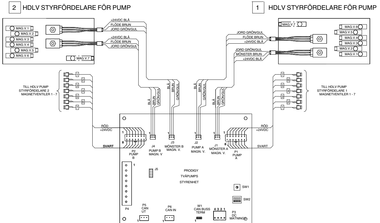
Bild 8 Kopplingschema för anslutningar mellan kretskort och pumppördelare
