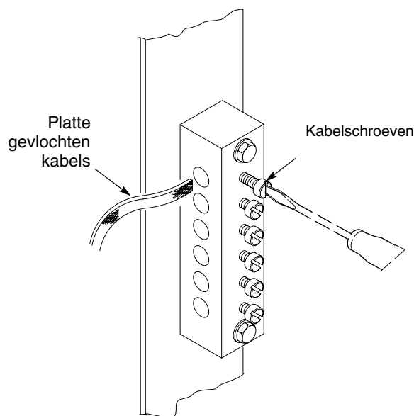
Afbeelding 2 Aansluiten van aardingskabels aan het blok
