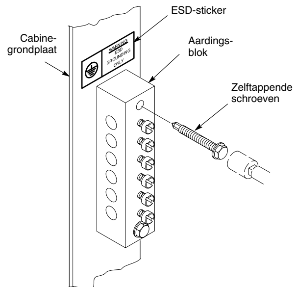
Afbeelding 1 Monteren van het aardingsblok
