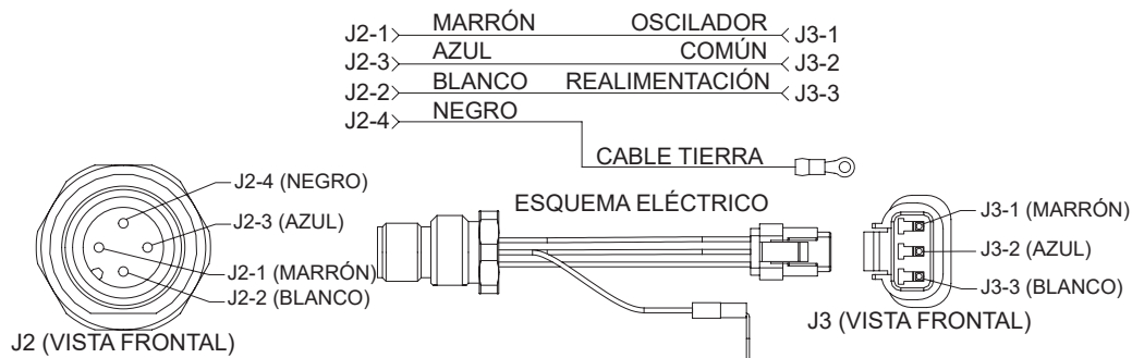
Figura 13 Cableado del receptáculo de la pistola
