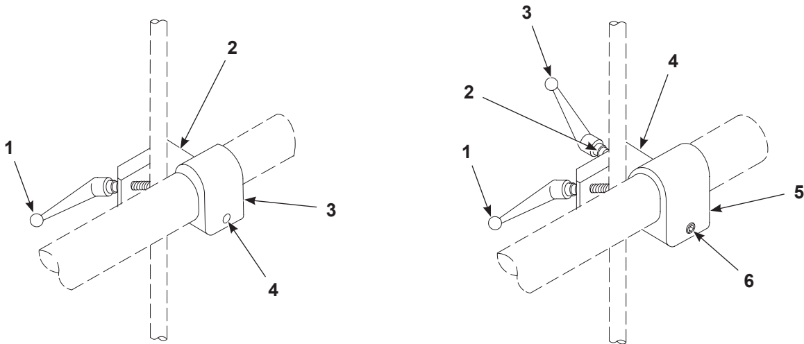
Figura 36 Montajes en barra de pistola para pistolas de montaje en tubo
