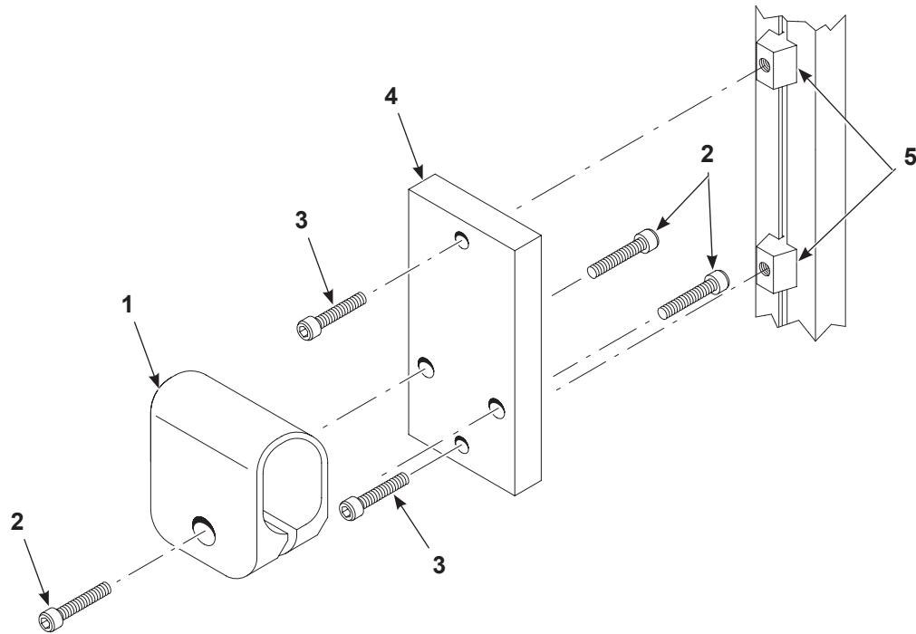
Figura 37 Conjunto de montaje de pistola de extrusión para pistolas de montaje en tubo
