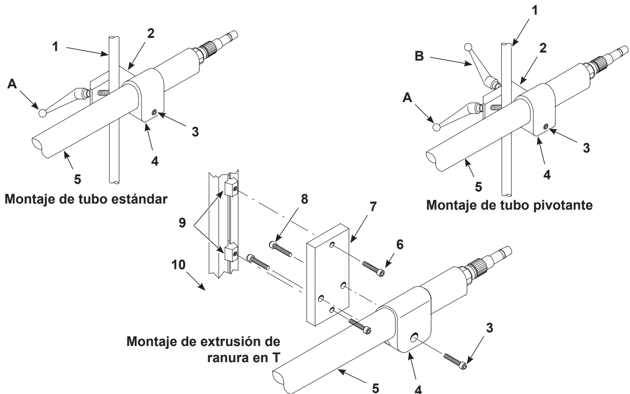
Figura 3 Conjuntos de montaje de la pistola de montaje en tubo
