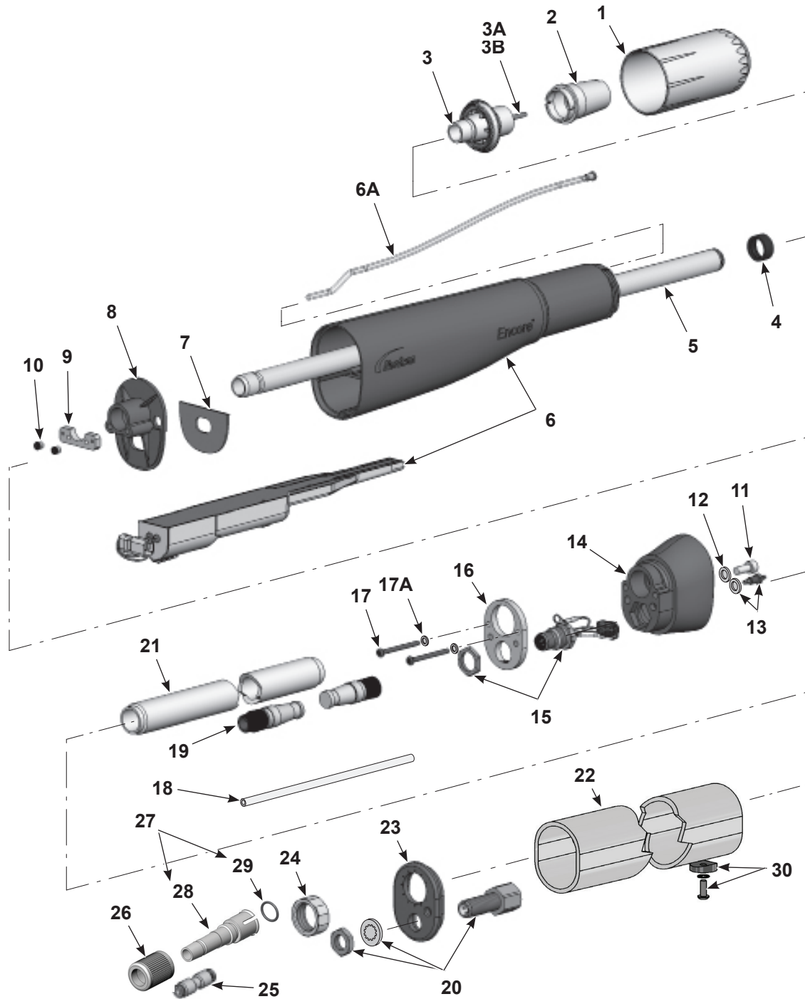
Figura 25 Piezas de la pistola de montaje en tubo
