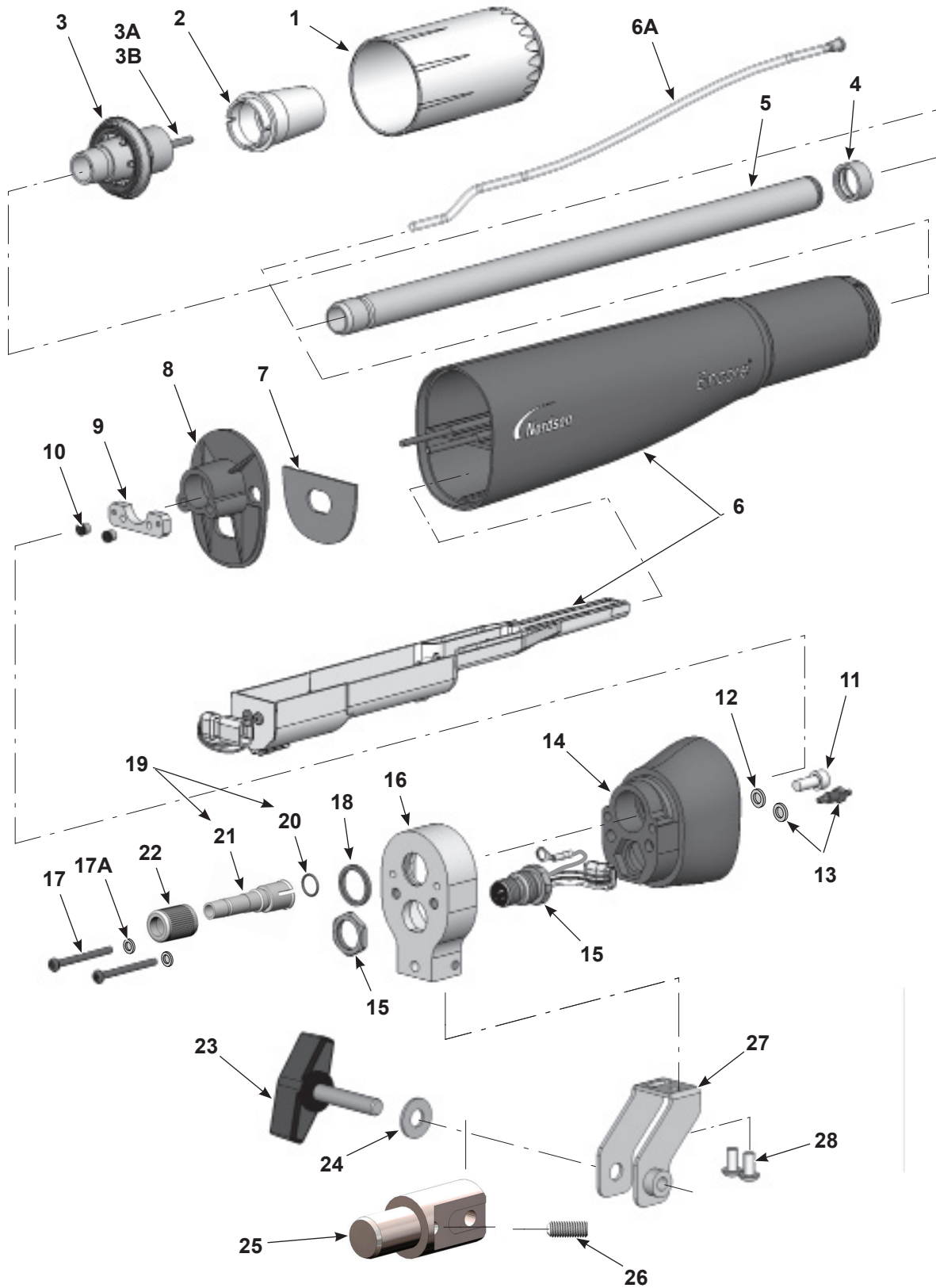
Figura 26 Piezas de la pistola de montaje en barra
