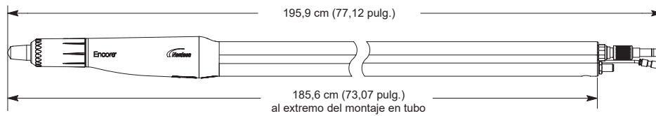
Figura 2 Dimensiones y pesos de las pistolas automáticas Encore
