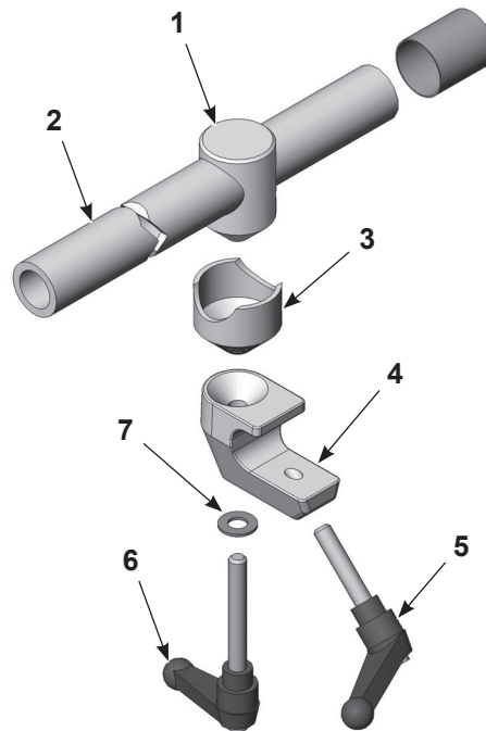
Figura 38 Barra de pistola para pistolas de montaje en barra
