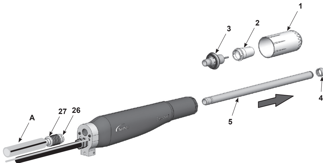
Figura 10 Mantenimiento - Pistola de montaje en barra mostrada sin montaje de pivote
