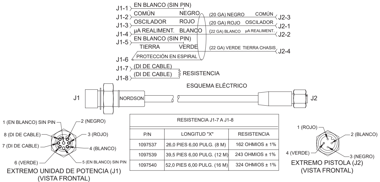
Figura 15 Cable de la pistola
