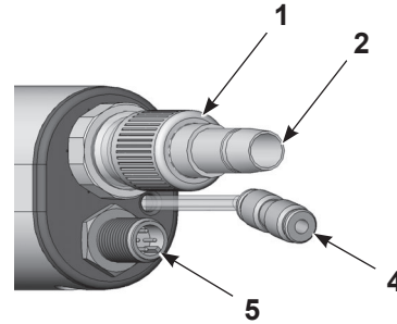
Pistola de montaje en tubo
