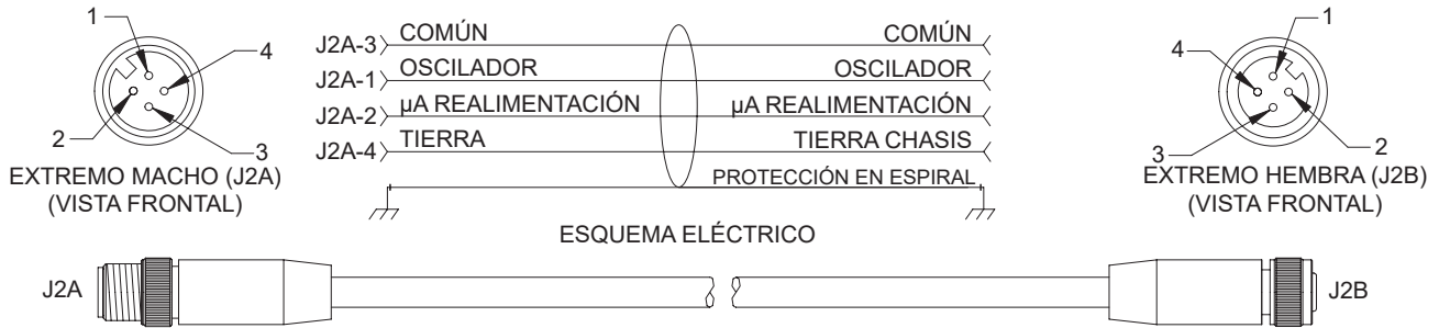
Figura 14 Cable alargador de pistola
