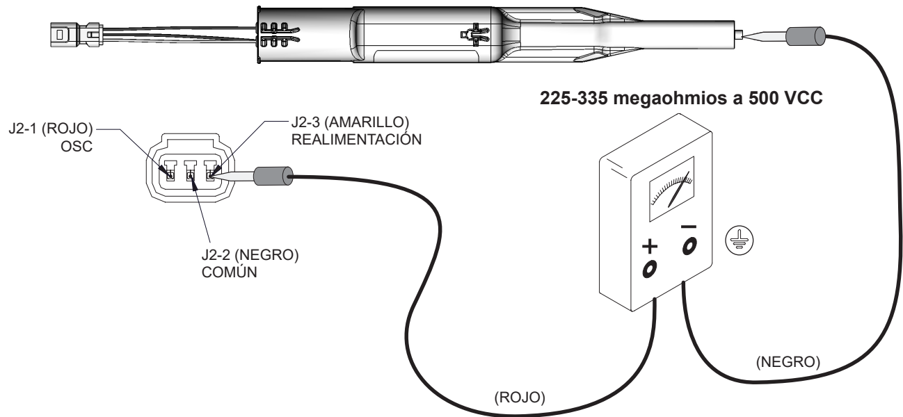
Figura 11 Prueba de resistencia del suministro de tensión (se muestra para un suministro de tensión negativo)
