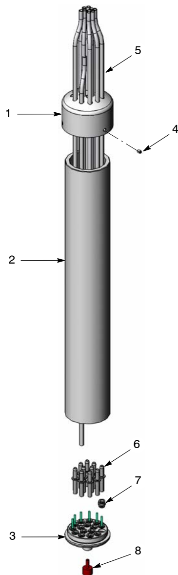
Paveikslėlis 2 Vamzdelių montažo remontas ir dalys
