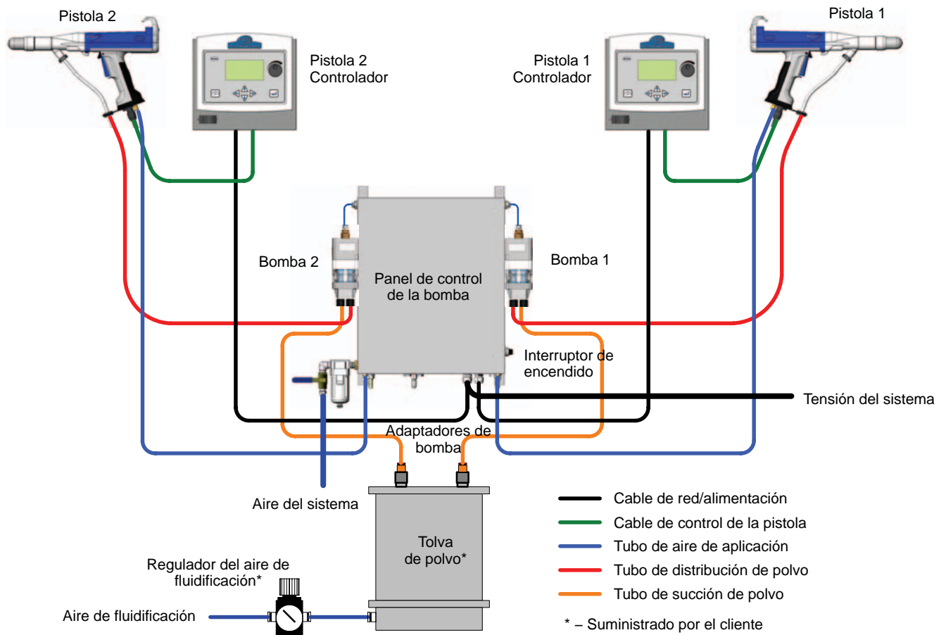
Figura 1 Diagrama del sistema (se muestra un sistema de dos pistolas)
