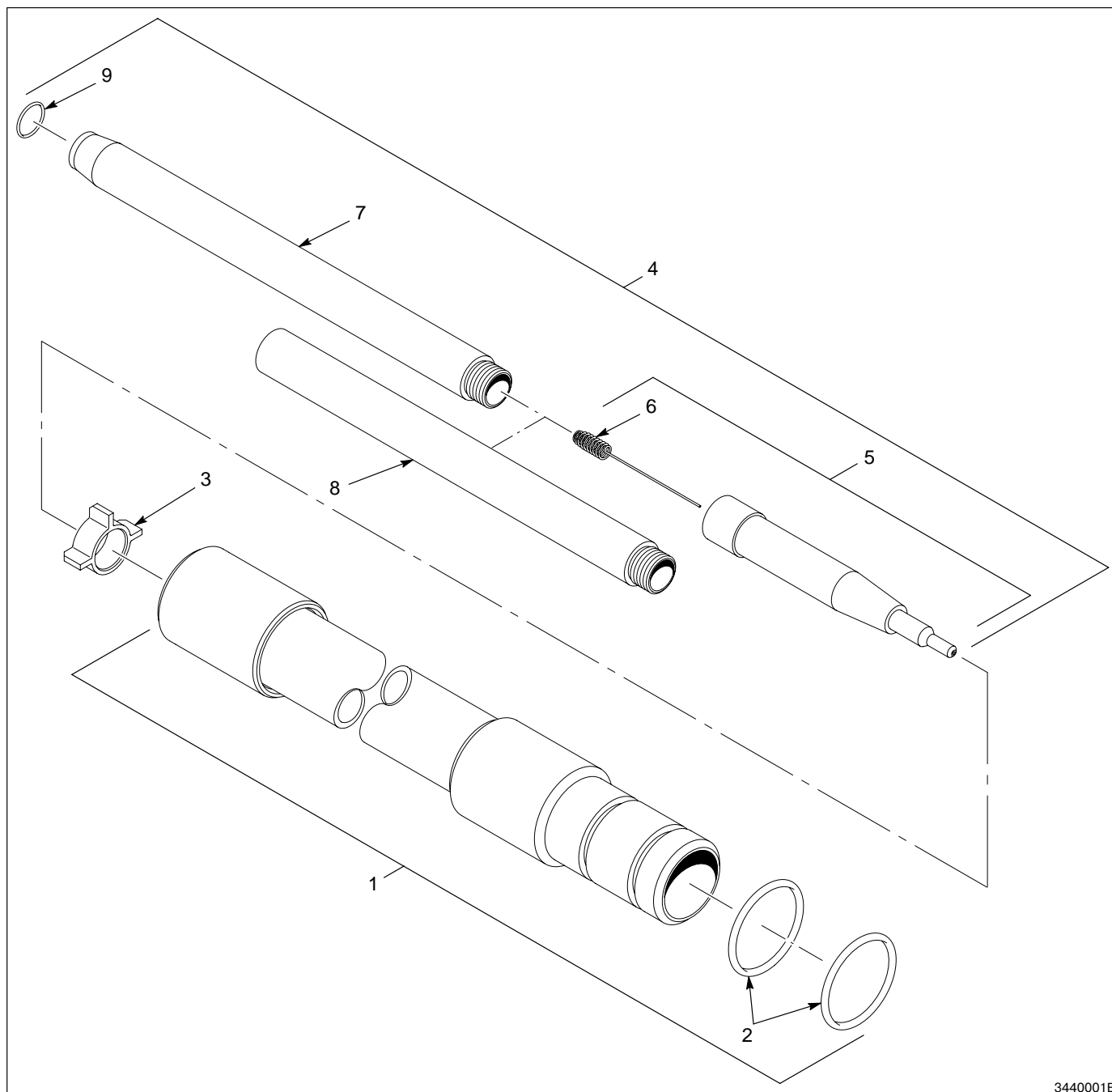
Рис. 1 Удлинитель ствола распылителя Sure Coat
