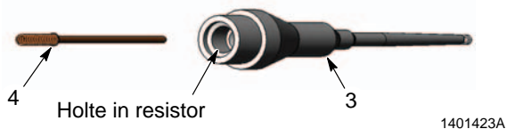
Afbeelding 6 Verwijderen van resistor uit resistorhouder
