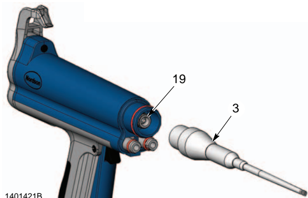
Afbeelding 4 Verwijderen van de resistorhouder
