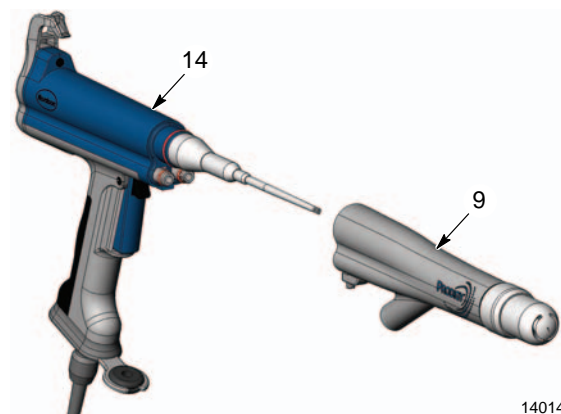
Afbeelding 3 Verwijderen van de adapter
