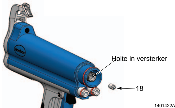
Afbeelding 5 Verwijderen van contactstuk
