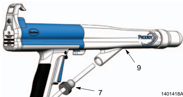
Afbeelding 1 Loshalen van de poederslang
