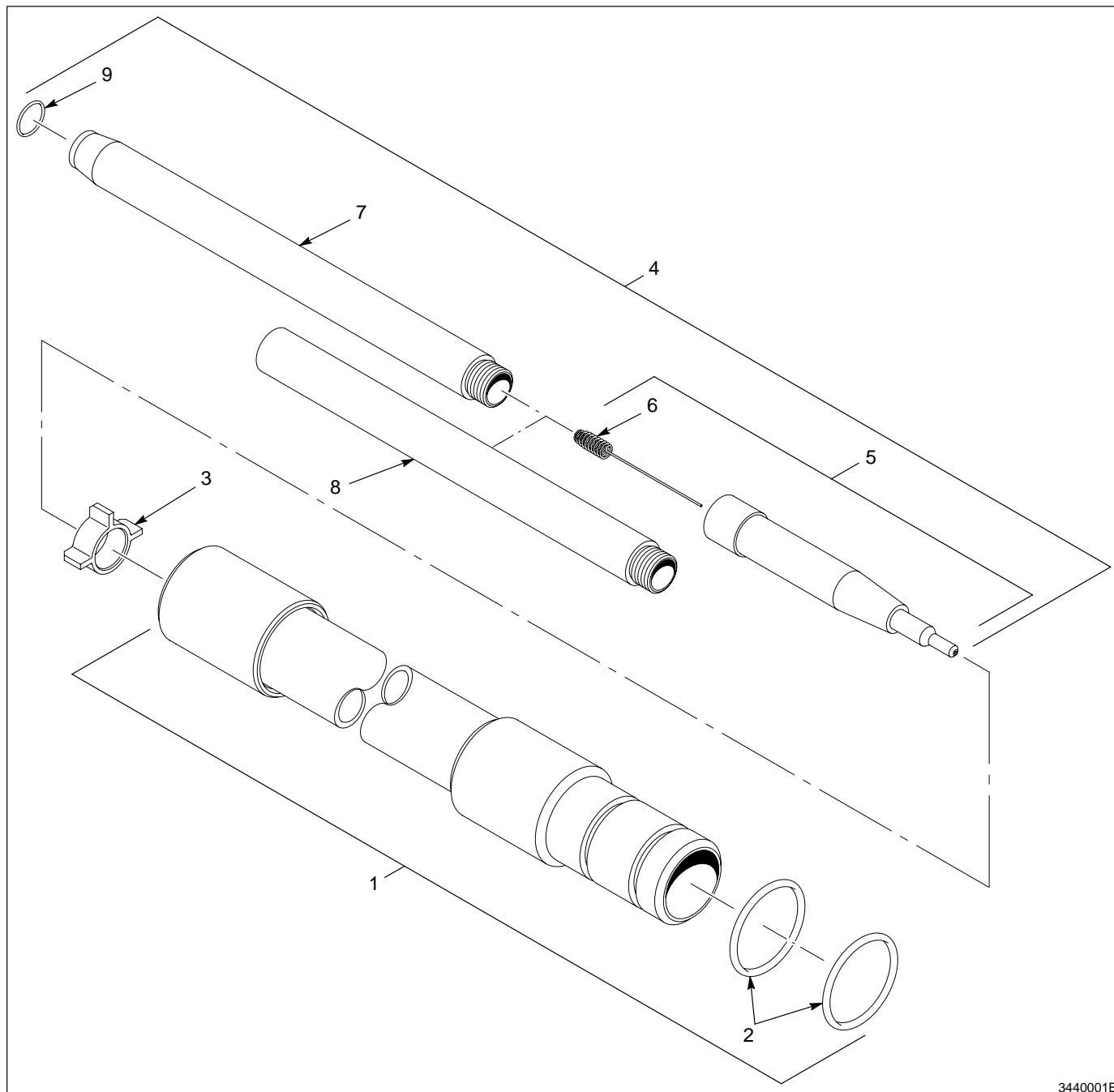
Fig. 1 Extensão para pistola Sure Coat
