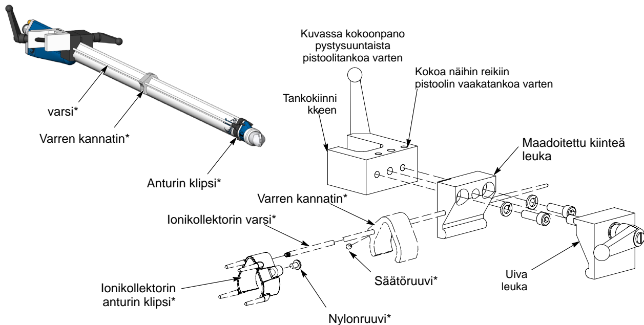
Kuva 1 Putkiinittainen pistoolikiinnike (*= ionikollektorin osat)
