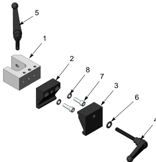
Kuva 2 Putkikiinnitteinen pistoolikiinnike (lisävaruste)
