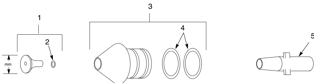
Kuva 5 Lyhyt kartiosuutin ja ilmansuuntaimet
