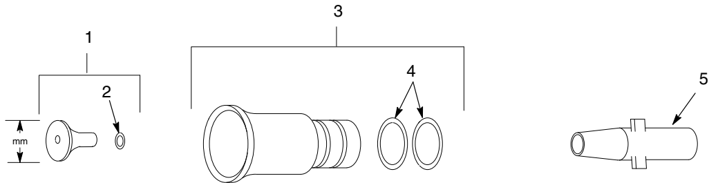
Kuva 4 45-mm kartiosuutin ja ilmansuuntain
