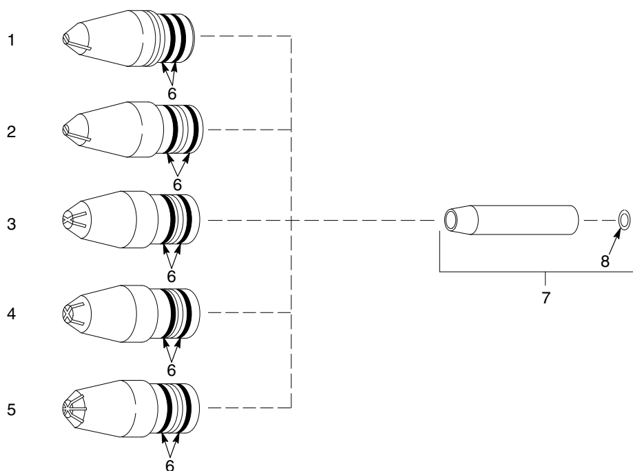
Kuva 2 Tasosuuttimen osat
