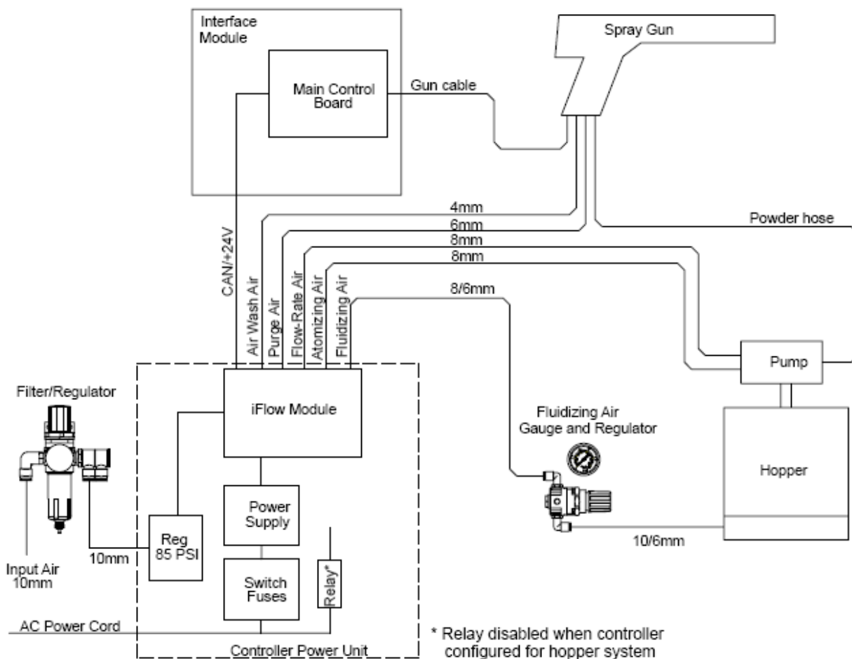
图 2-2 Encore 手动式粉末喷涂系统方框图
