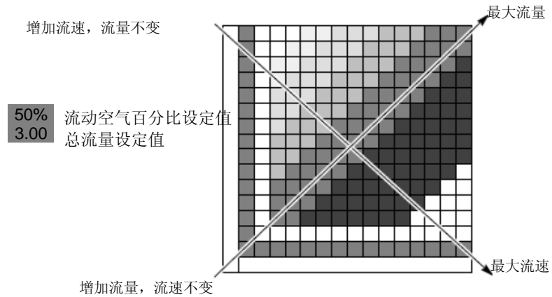
图 3-16 智能流量图表
