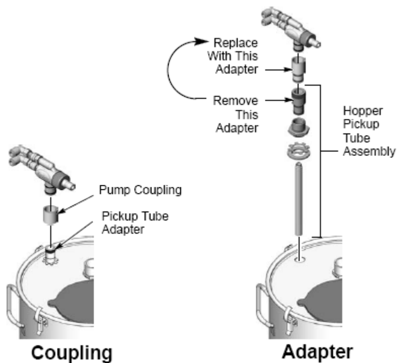
图 2-7 泵安装
