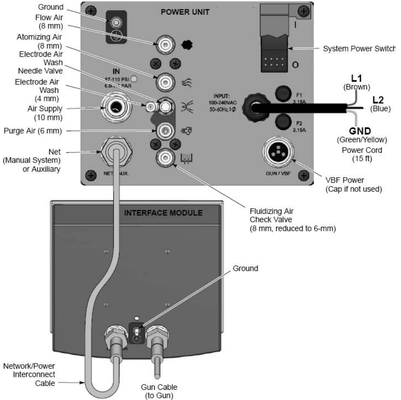
图 2-3 Encore 喷枪控制器连接
