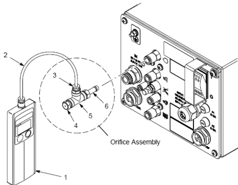
图 5-18 空气检定套件的使用
