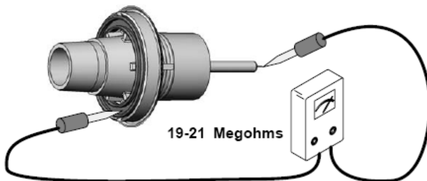
图 4-3 电极装置电阻测试
