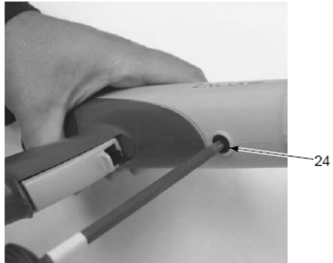
图 5-5 旋下枪身螺钉
