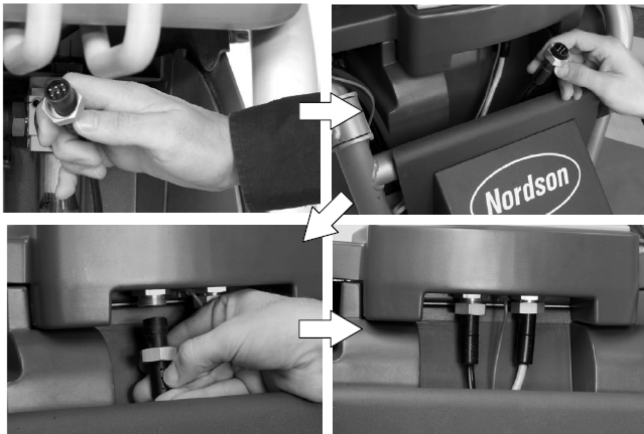
图 2-9 喷枪电缆连至控制器界面模块
