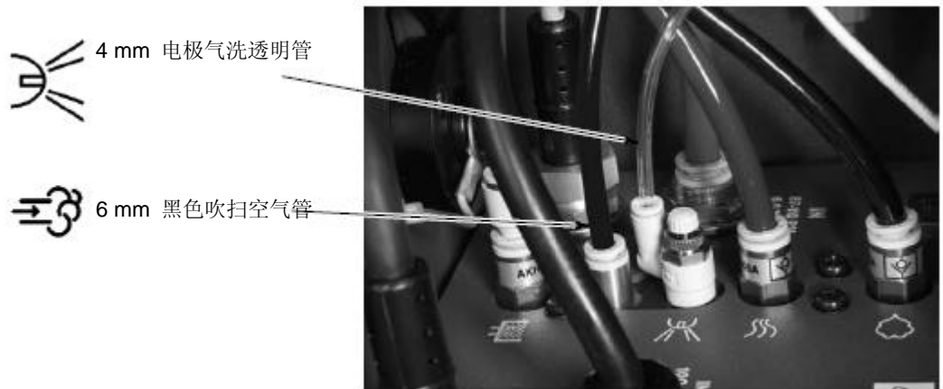
图 2-11 喷枪和吹扫空气管连接控制器
