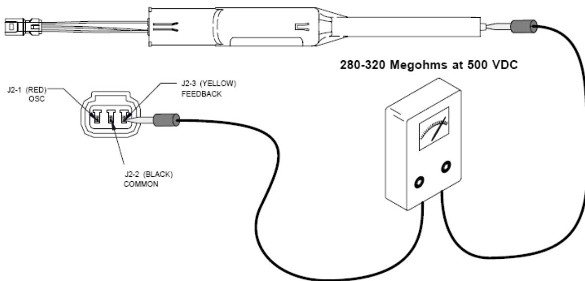
图 4-2 电源电阻测试
