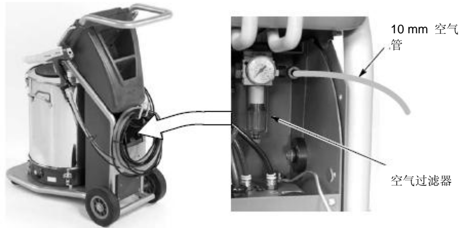
图 2-13 系统气源连接
