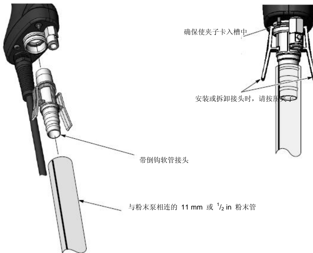
图 2-12 粉末管连接喷枪
