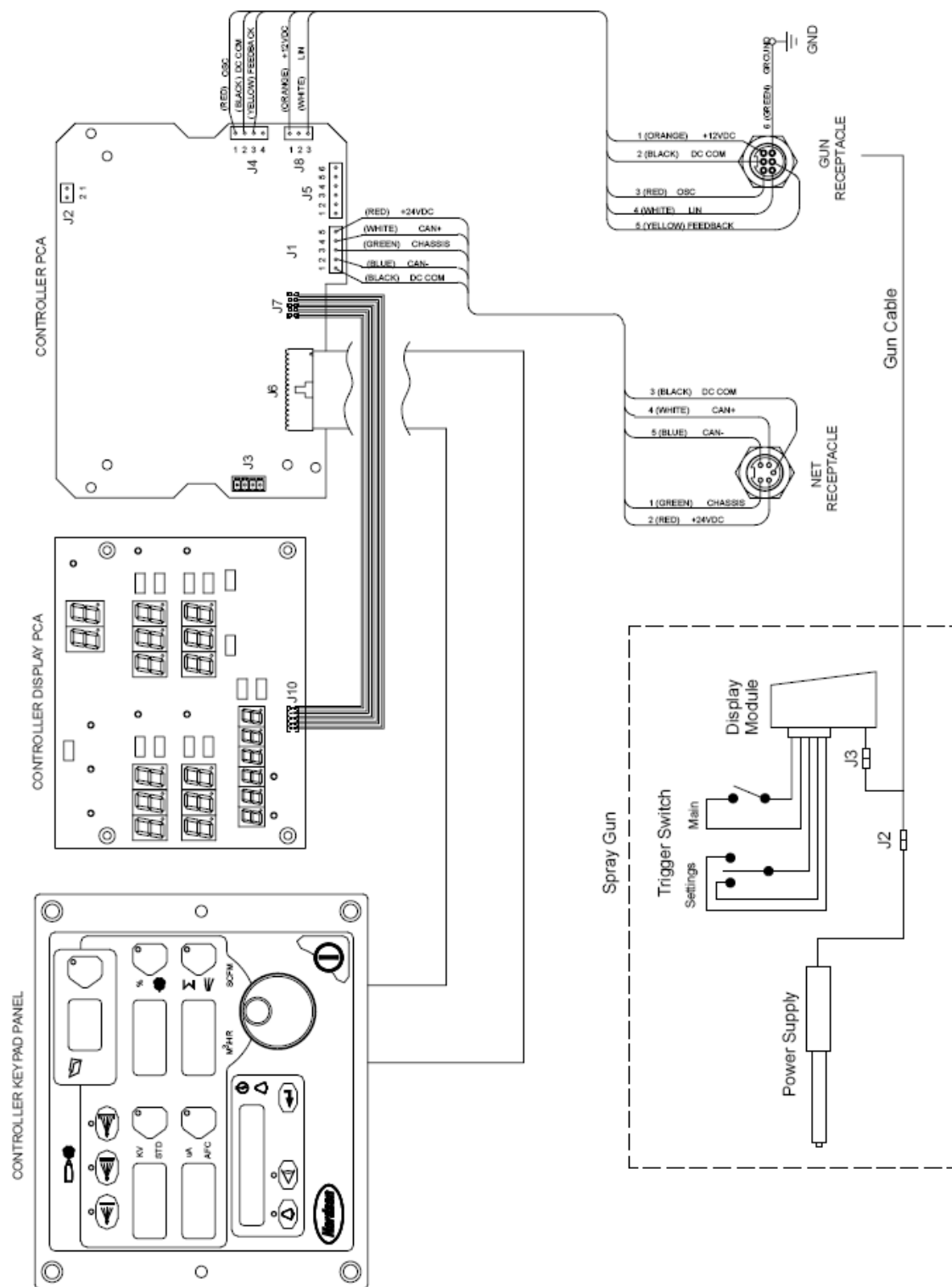
图 4-7 控制器界面布线图
