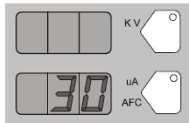
AFC 模式 — kV 设定
