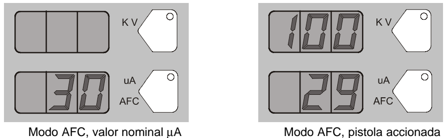
Fig. 3-14 Modo AFC, pantallas de los valores nominales y de la pistola accionada
