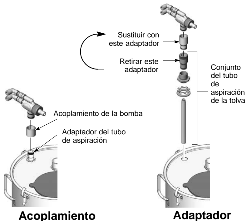
Fig. 2-7 Montaje de la bomba
