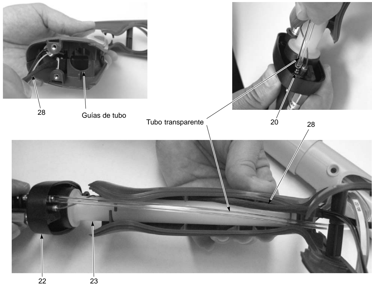
Fig. 5-11 Montaje de las partes de la empuñadura y la base
