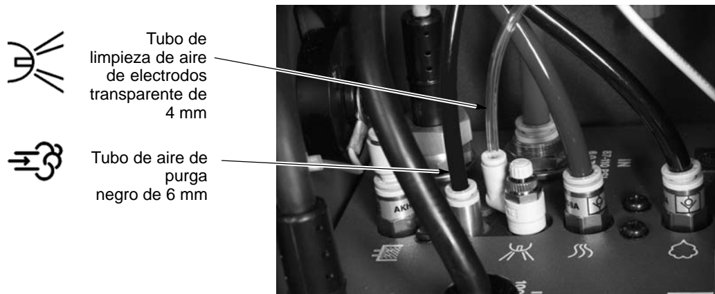
Fig. 2-11 Conexión de los tubos del aire de la pistola y del aire de purga al controlador
