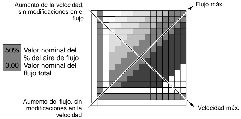
Fig. 3-16 Lectura de las tablas correspondientes al modo Smart Flow
