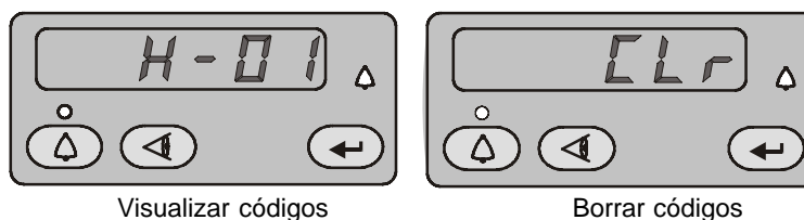
Fig. 3-8 Visualización y borrado de los códigos de ayuda
