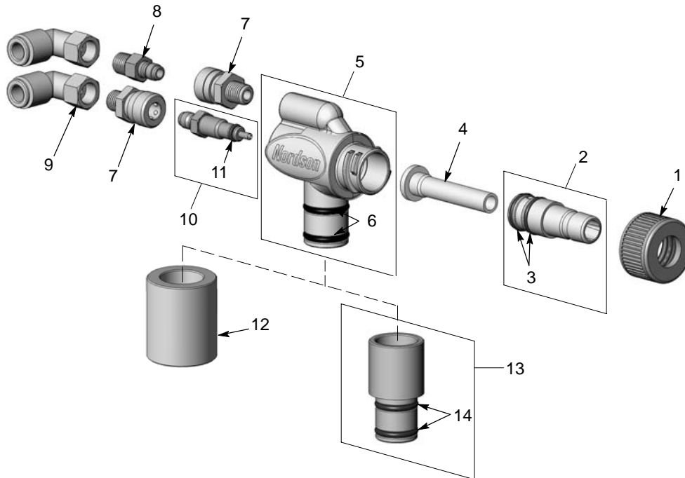
Fig. 6-8 Piezas de la bomba
