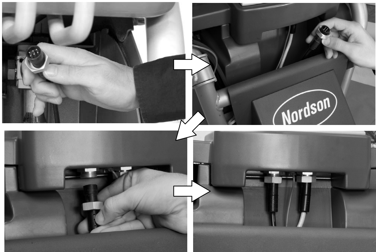
Fig. 2-9 Conexión del cable de la pistola al módulo de la interfaz del controlador.
