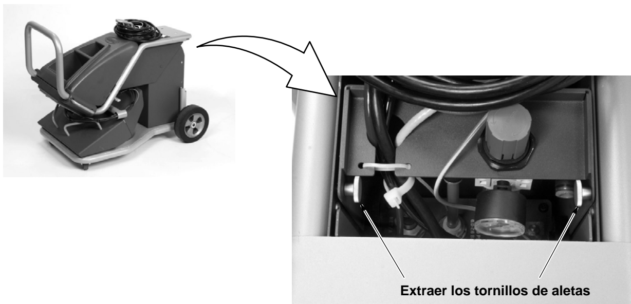
Fig. 2-4 Preparación para desplegar el mango de la carretilla (se muestra el sistema VBF)
