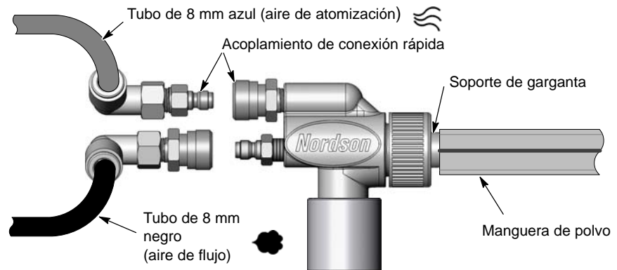
Fig. 2-8 Montaje de la bomba
