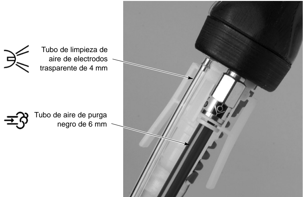
Fig. 2-10 Conexión del tubo de polvo y del tubo de aire a la pistola de aplicación
