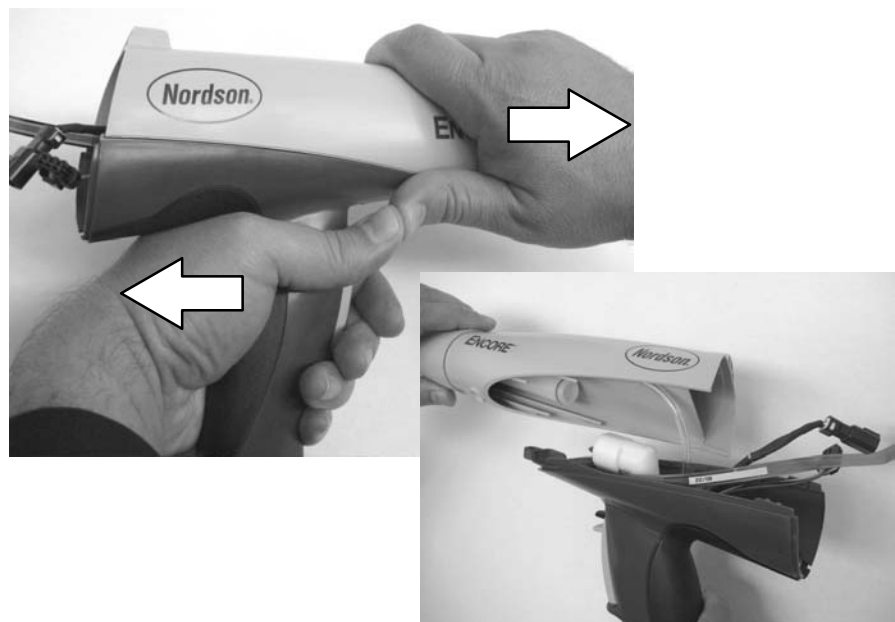
Fig. 5-6 Separación de la empuñadura y el cuerpo de la pistola
