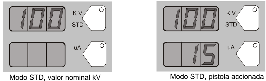
Fig. 3-13 Modo STD, pantallas de los valores nominales y de la pistola accionada
