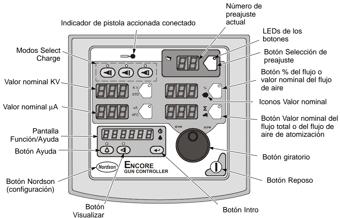
Fig. 3-6 Interfaz del controlador
