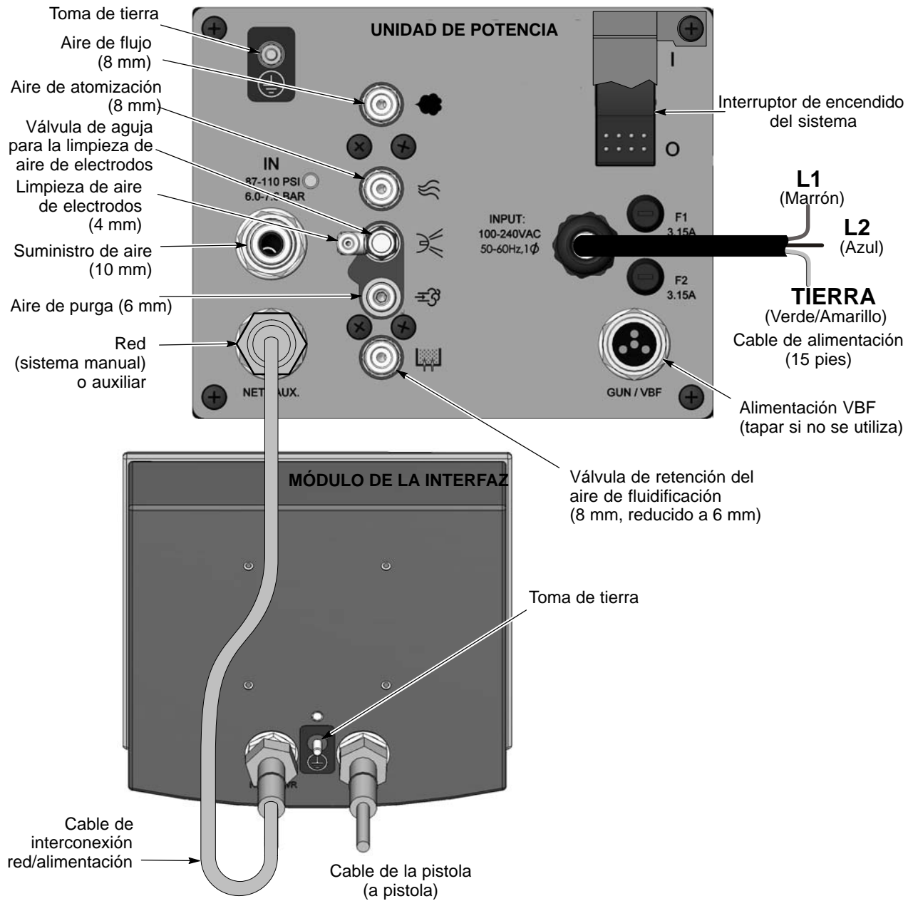
Fig. 2-3 Conexiones del controlador de pistolas Encore
