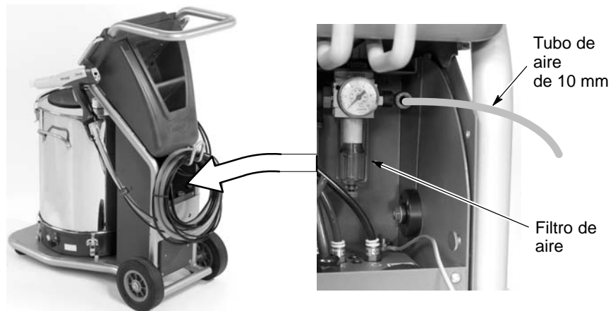
Fig. 2-13 Conexión del suministro de aire del sistema
