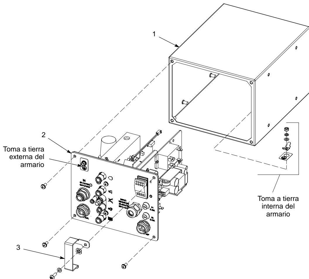
Fig. 5-16 Extracción del subpanel
