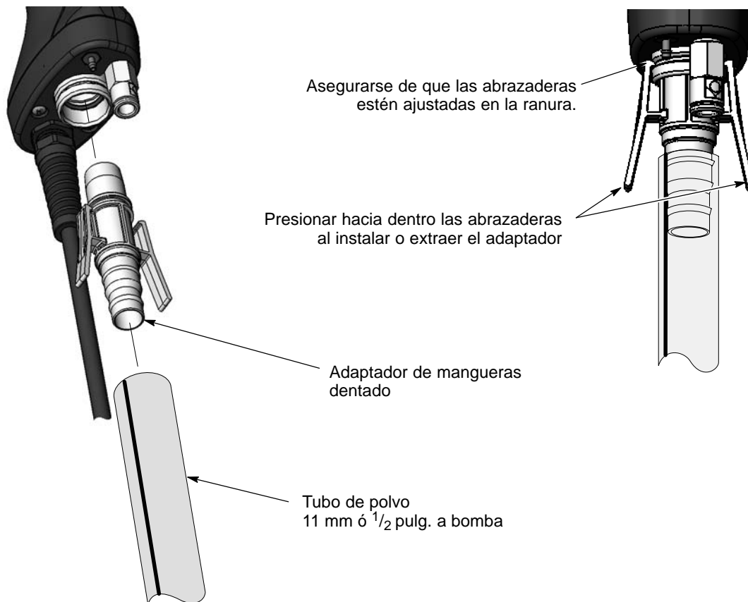
Fig. 2-12 Conexión del tubo de polvo a la pistola de aplicación
