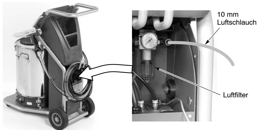
Abb. 2-11 Pneumatischer Systemanschluss
