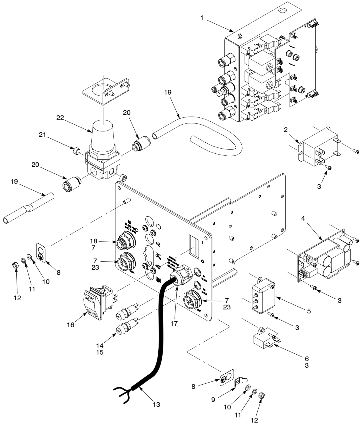
Abb. 6-6 Spannungsversorgungsmodul
