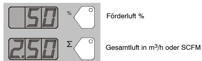
Abb. 3-18 Verfahren Smart Flow – Förderluft % oder Gesamtluft \Sigma
