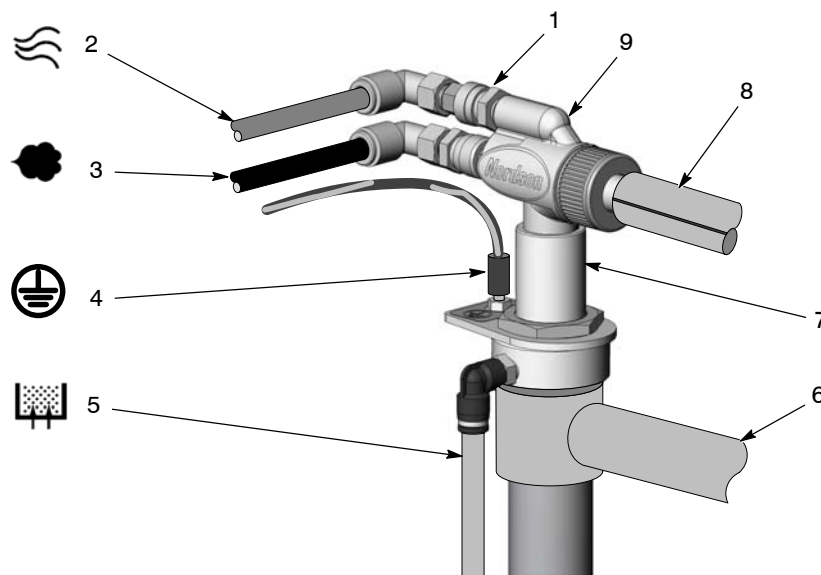
Abb. 2-6 Entnahmerohr und Pumpe installieren
