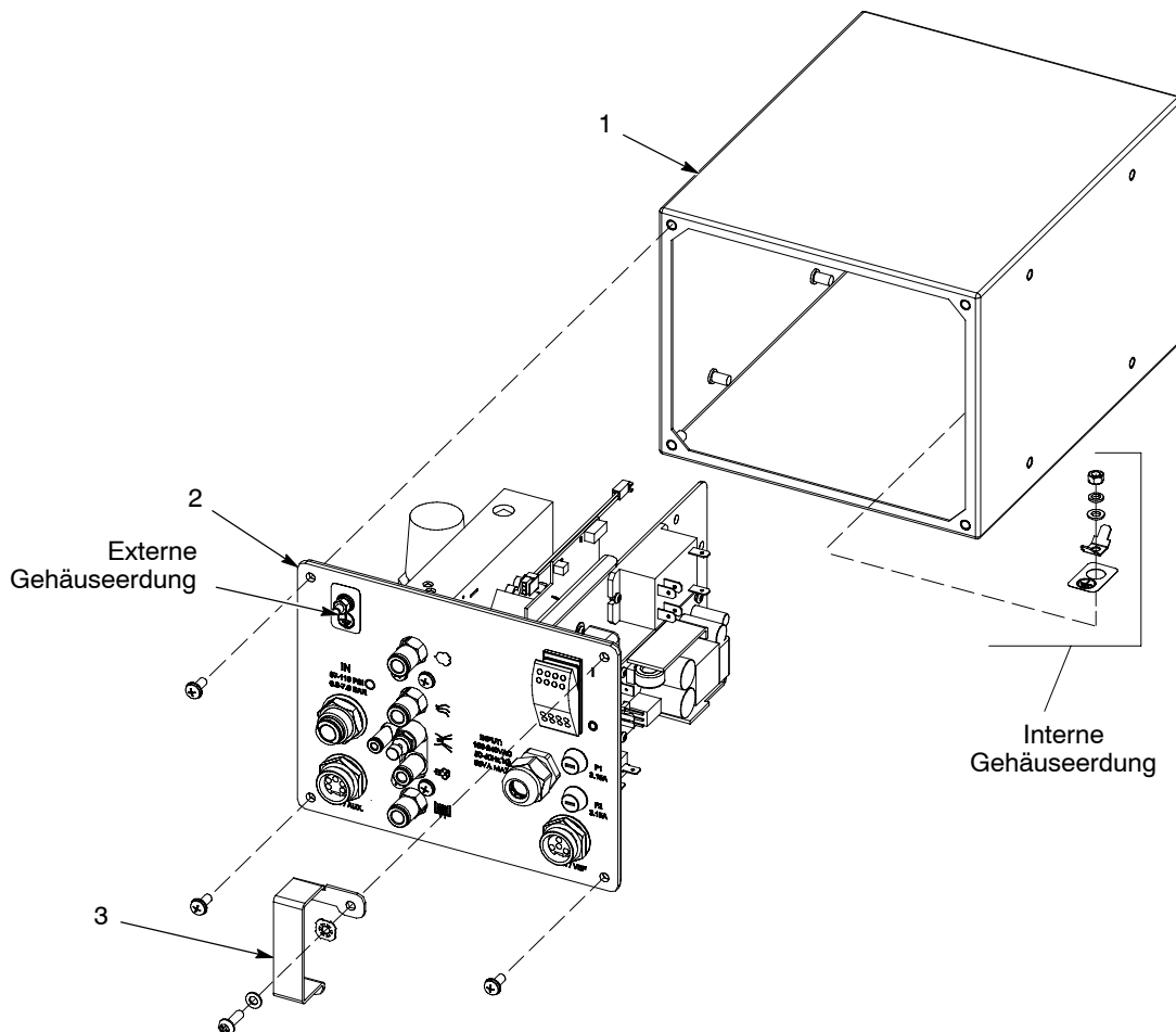
Abb. 5-16 Unterkonsole abnehmen
