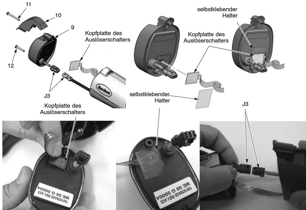
Abb. 5-1 Anzeigemodul ersetzen
