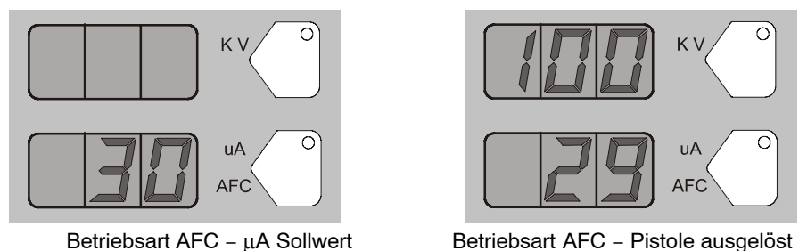
Abb. 3-15 Betriebsart AFC – Sollwerte und Anzeigen bei ausgelöster Pistole
