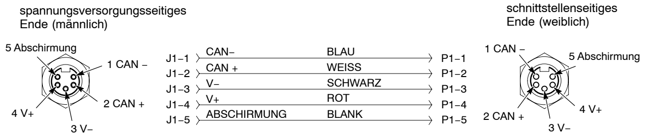
Abb. 4-5 Verbindungskabel der Steuerung; Verkabelung
