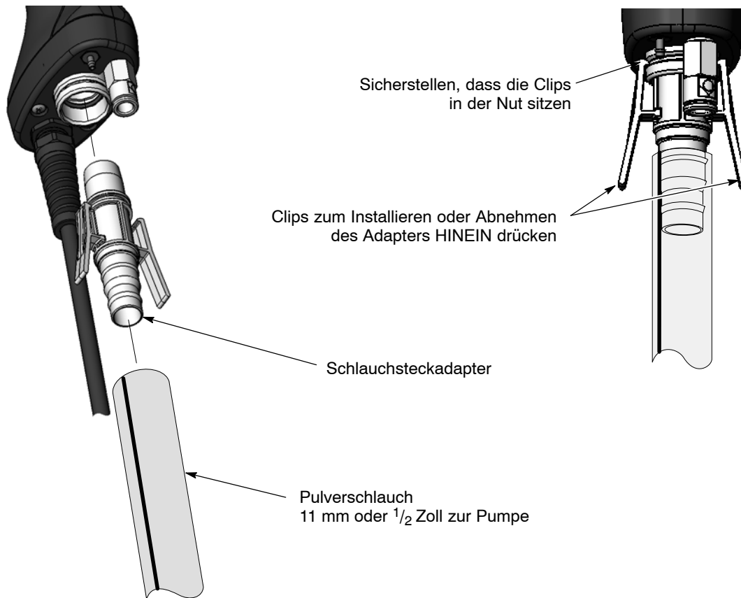
Abb. 2-10 Pulverschlauch an die Sprühpistole anschließen
