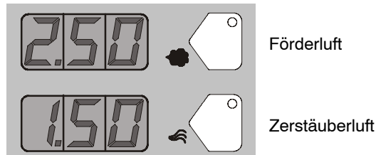
Abb. 3-19 Verfahren Classic – Sollwerte für Förderluft oder Zerstäuberluft
