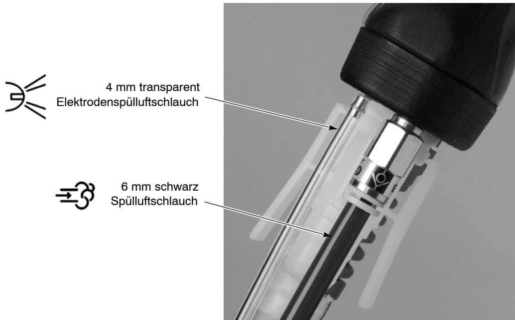
Abb. 2-8 Pulver- und Luftschläuche an die Sprühpistole anschließen
