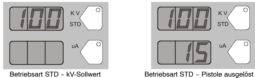
Abb. 3-14 Betriebsart STD – Sollwerte und Anzeigen bei ausgelöster Pistole
