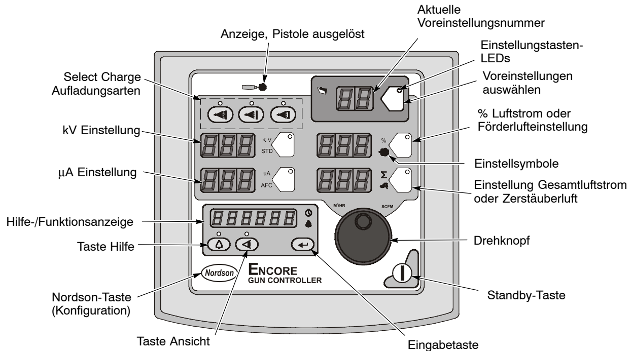
Abb. 3-7 Steuerungs-Schnittstelle
