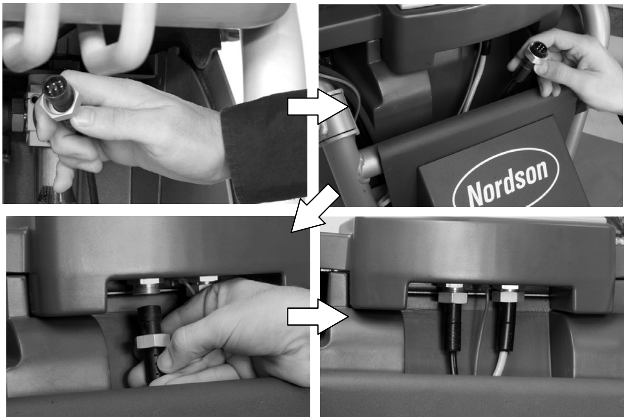
Abb. 2-7 Pistolenkabel an das Schnittstellenmodul der Steuerung anschließen
