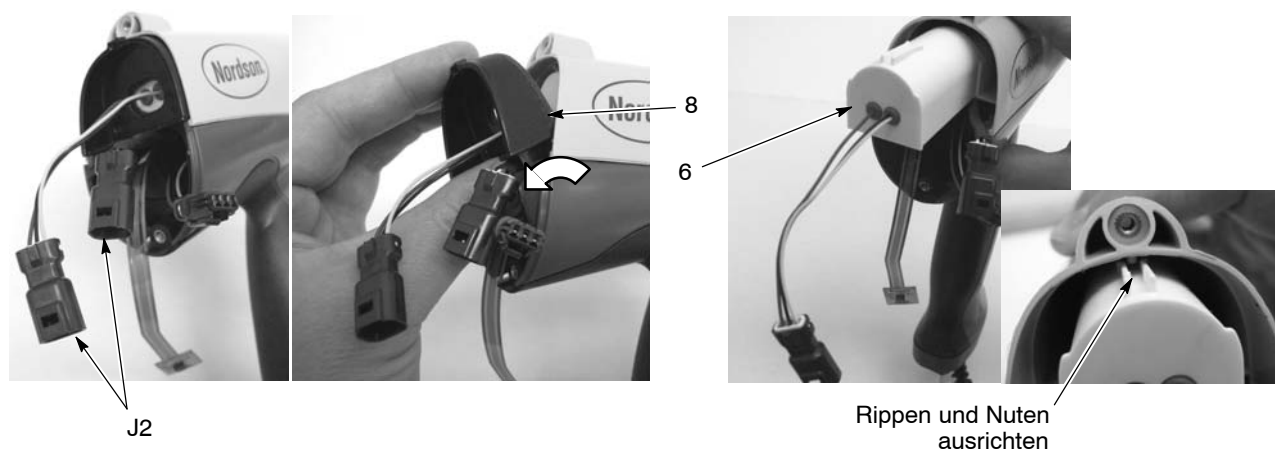
Abb. 5-2 Spannungsversorgung ersetzen
