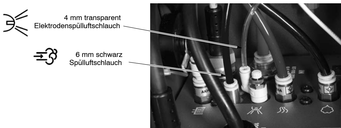
Abb. 2-9 Pistolen- und Spülluftschlauch an die Steuerung anschließen
