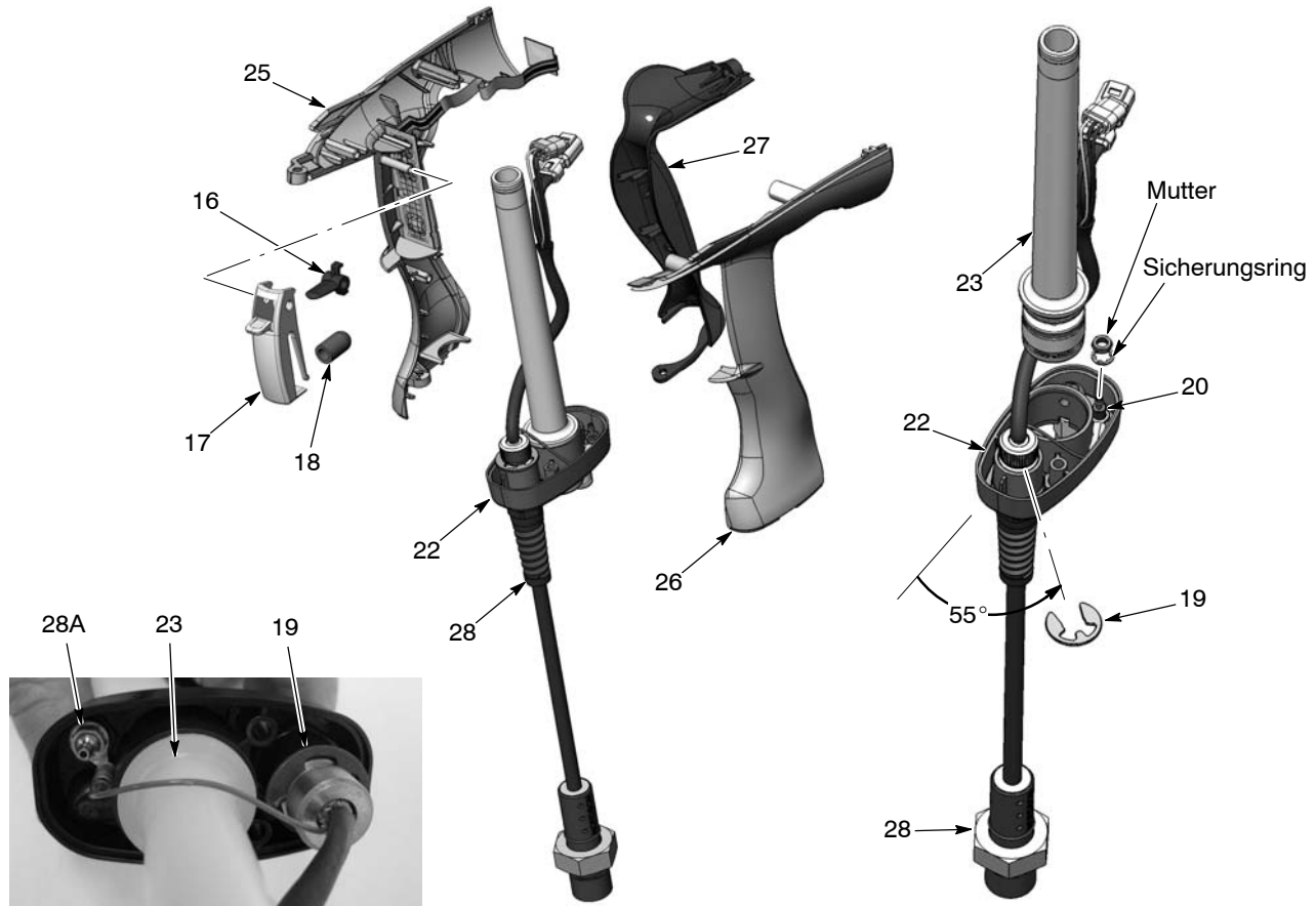
Abb. 5-9 Pistole fertig zerlegen
