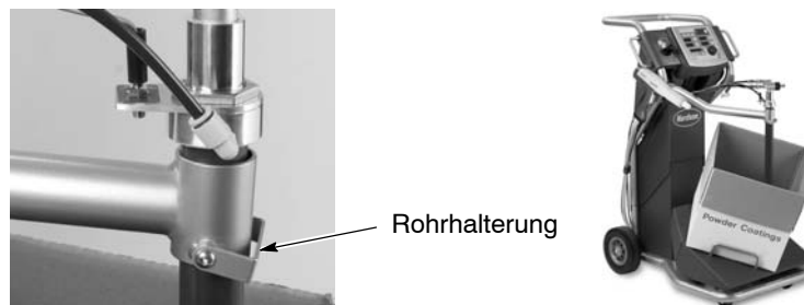
Abb. 3-3 Pulverkarton installieren
