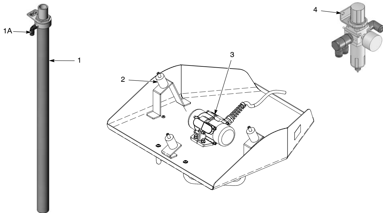
Abb. 6-8 Verschiedene Systemersatzteile
