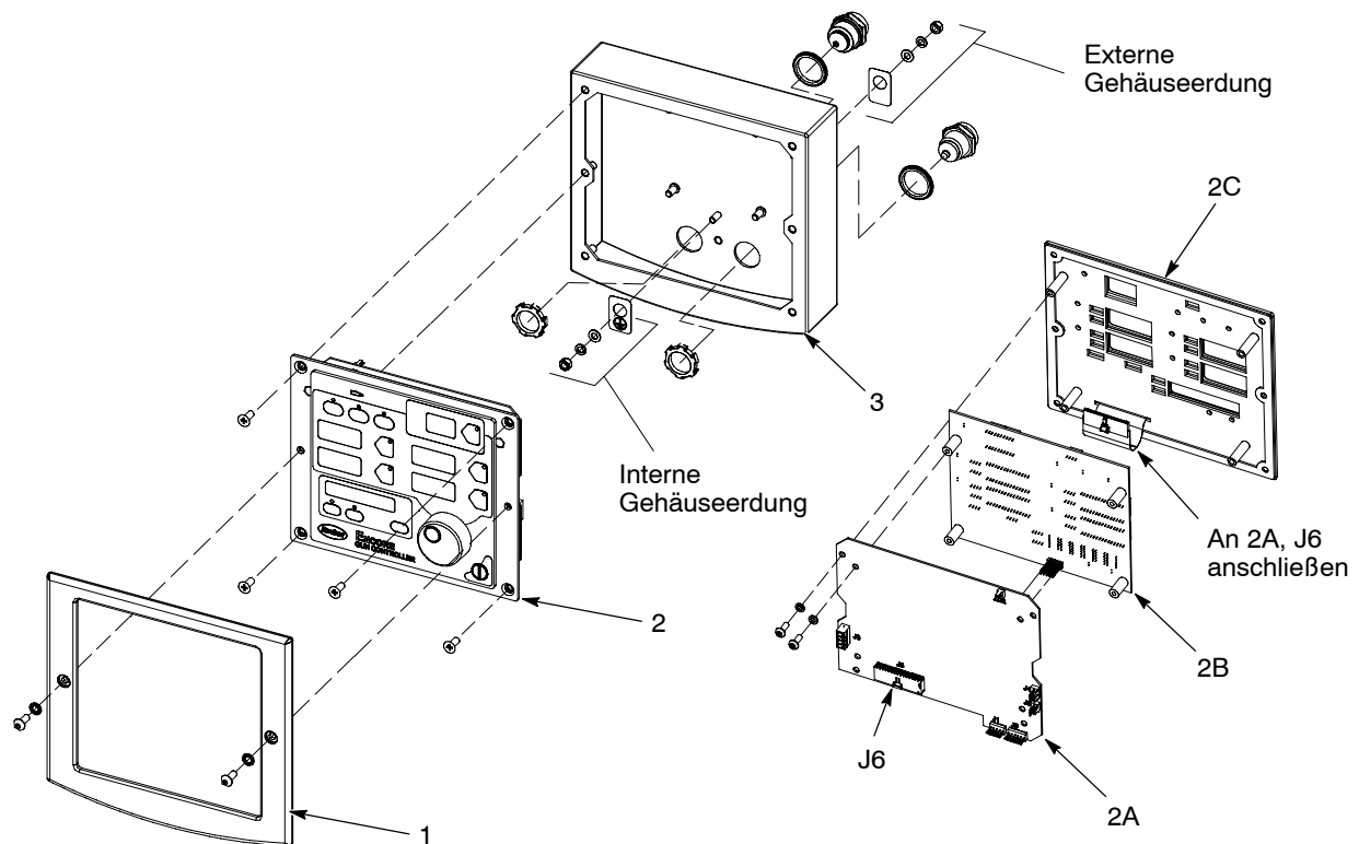
Abb. 5-15 Schnittstellenmodulbaugruppe
