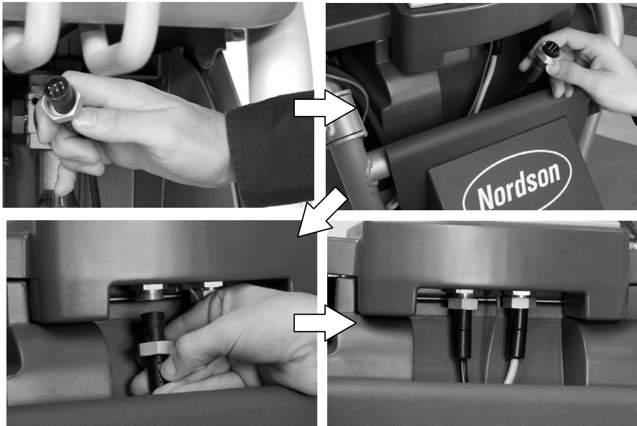
Afb. 2-9 Pistoolkabel aansluiten op de besturinginterfacemodule
