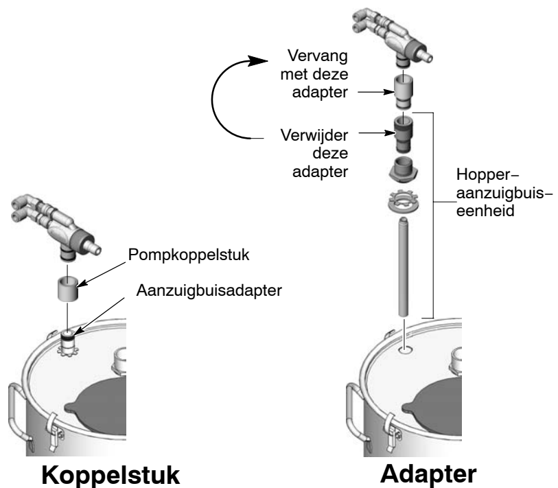
Afb. 2-7 Montage van pomp
