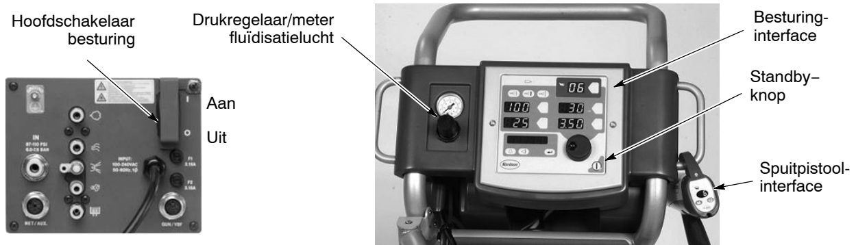
Afb. 3-1 Systeemschakelaars
