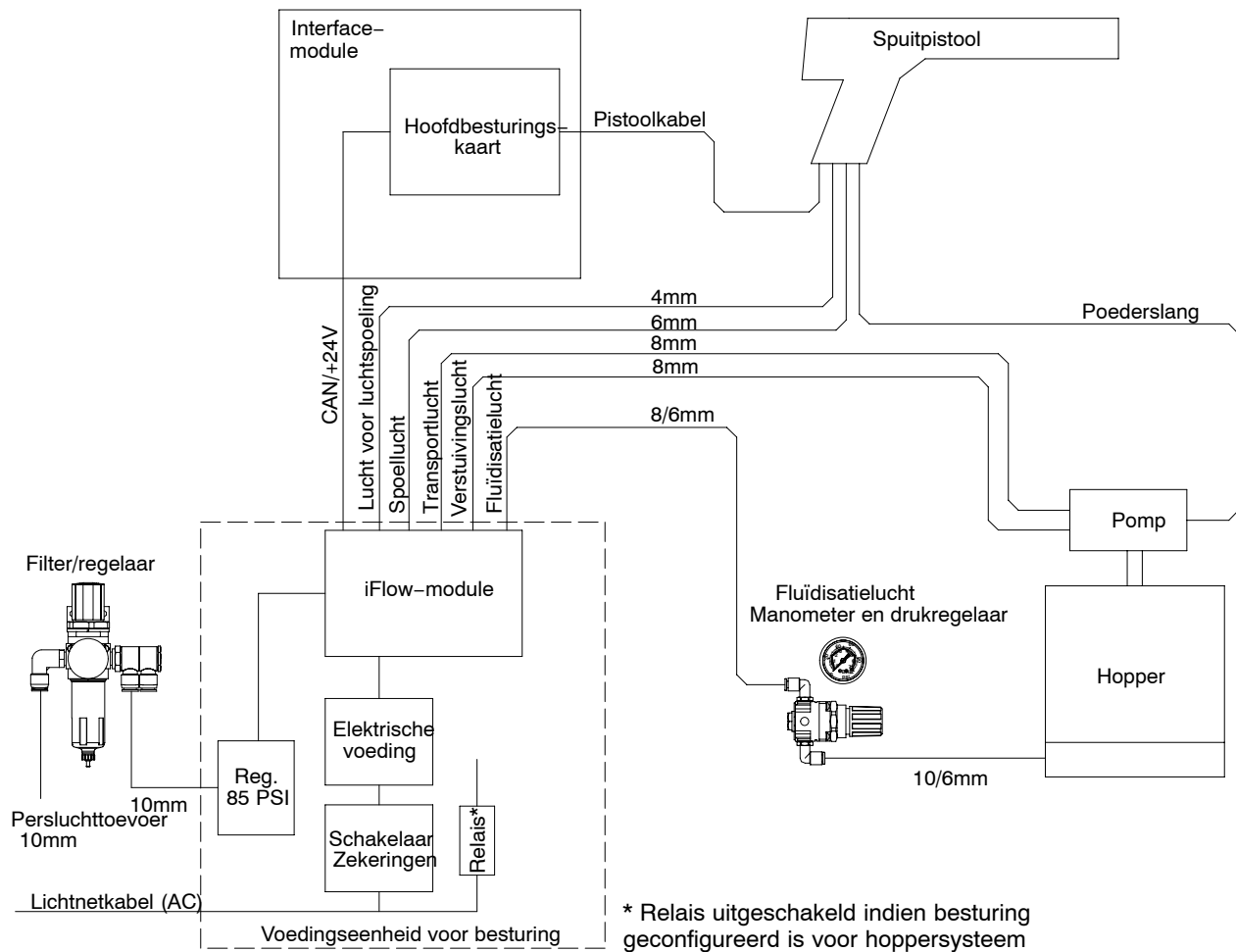
Afb. 2-2 Blokschema handbediend Encore-poederspuitsysteem
