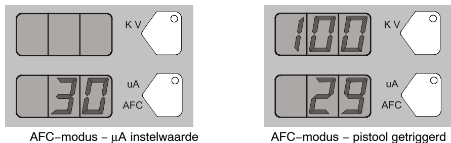
Afb. 3-14 AFC-modus – displays voor instelwaarde en voor getriggerd pistool
