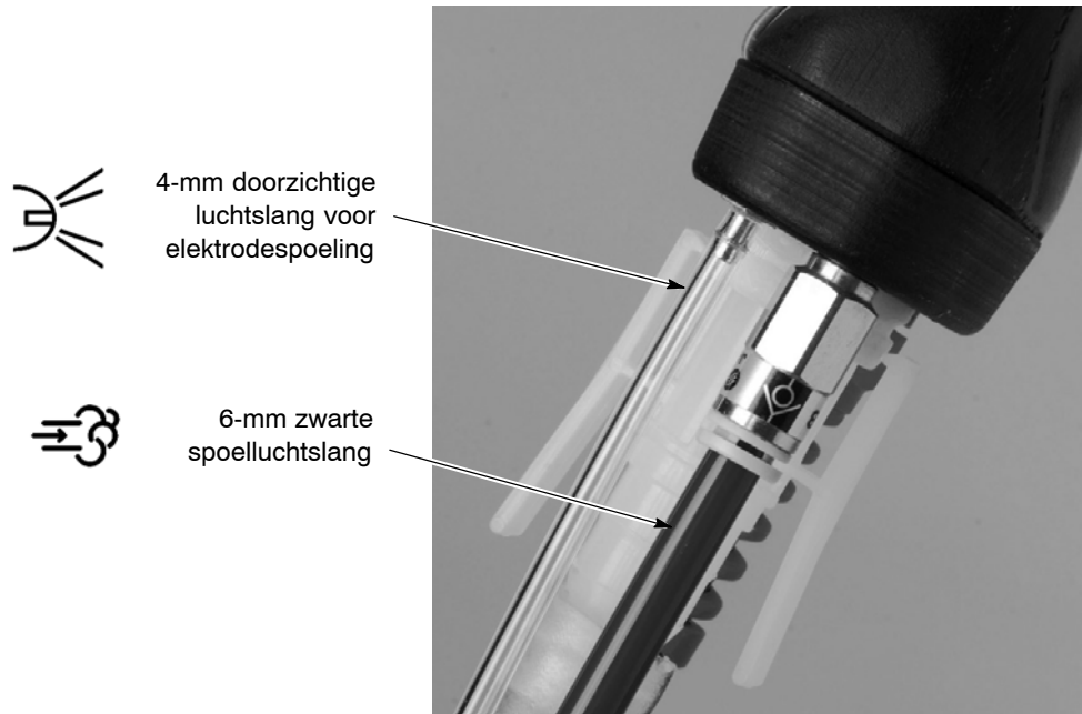
Afb. 2-10 Aansluiten van poeder- en pistoolluchtlangen aan spuitpistool
