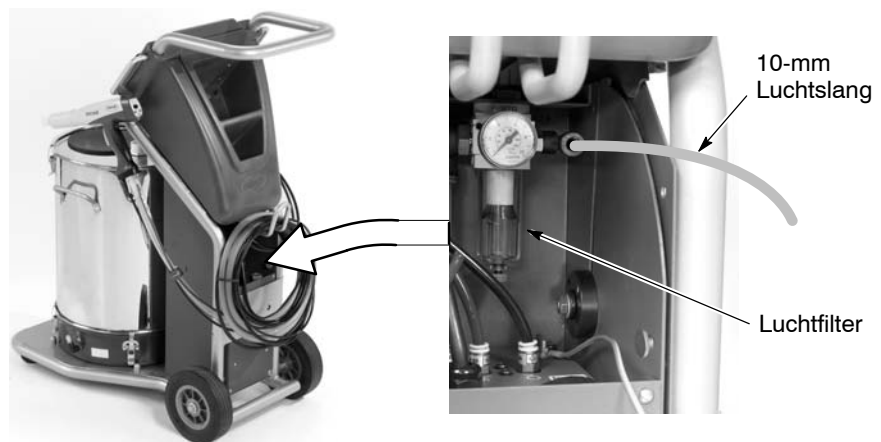
Afb. 2-13 Aansluiting voor persluchttoevoer
