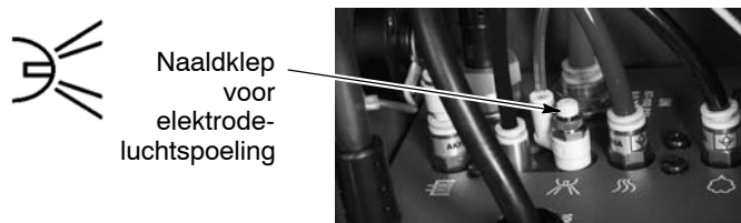
Afb. 3-3 Locatie van naaldklep voor elektrodeluchtspoeling
