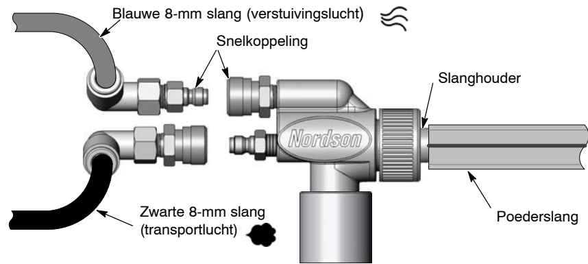
Afb. 2-8 Montage van pomp
