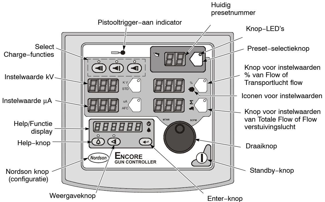
Afb. 3-6 Besturinginterface
