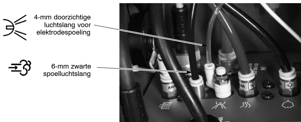
Afb. 2-11 Aansluiten van pistoollucht- en spoelluchtlangen aan de besturing
