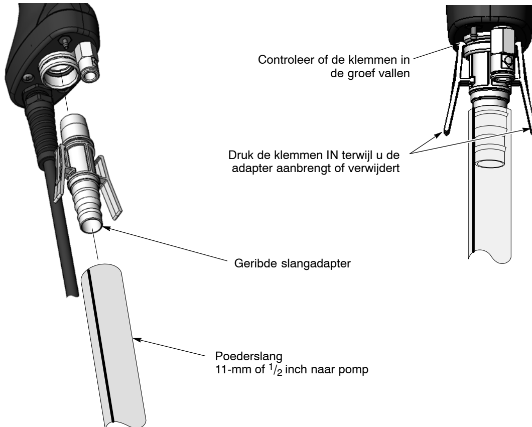
Afb. 2-12 Aansluiten van poederslang aan spuitpistool
