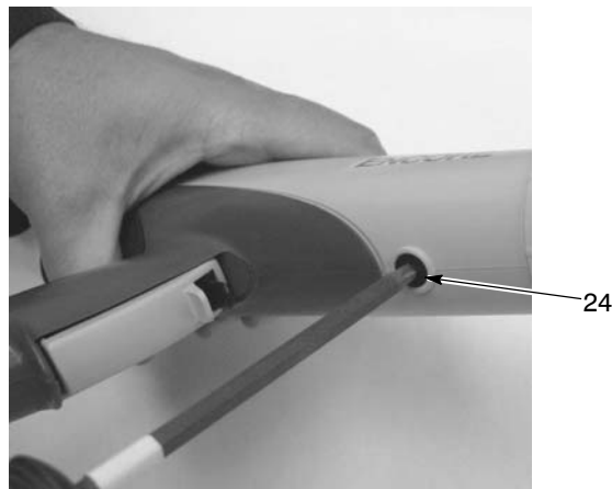
Afb. 5-5 Schroef in pistoolhuis verwijderen
