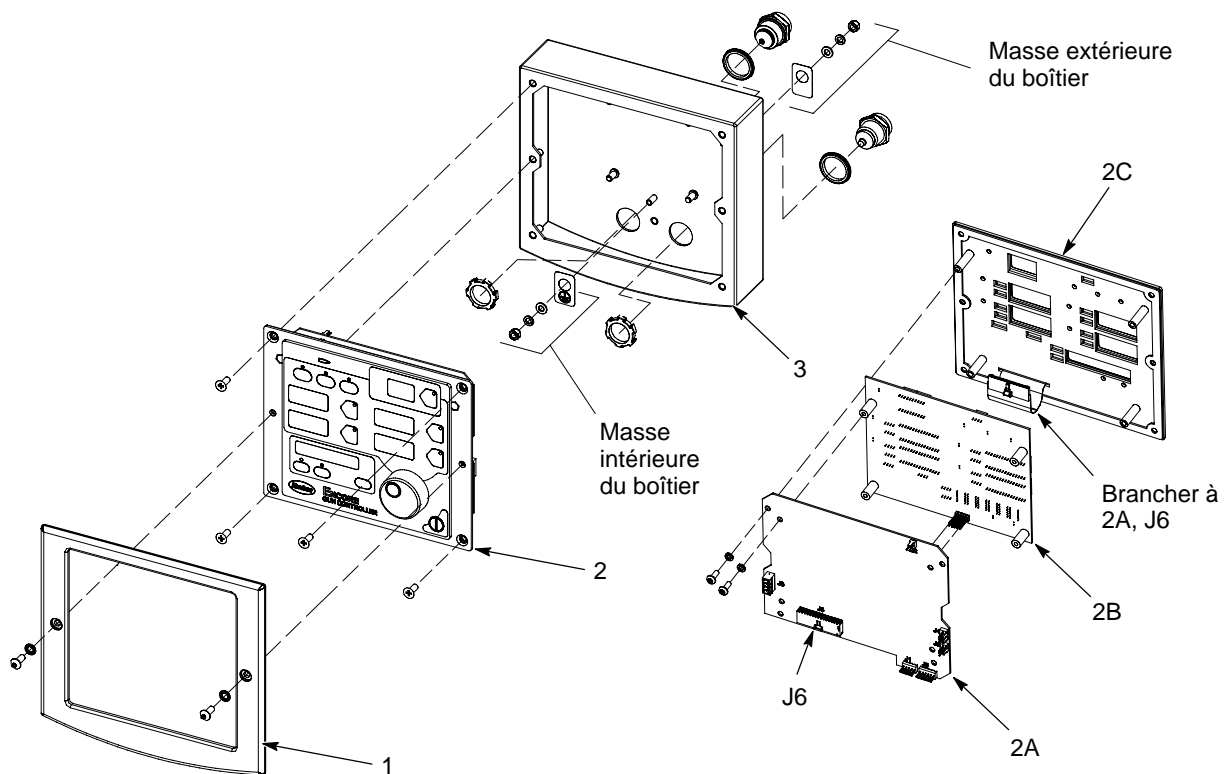
Fig. 5-15 Ensemble module d'interface
