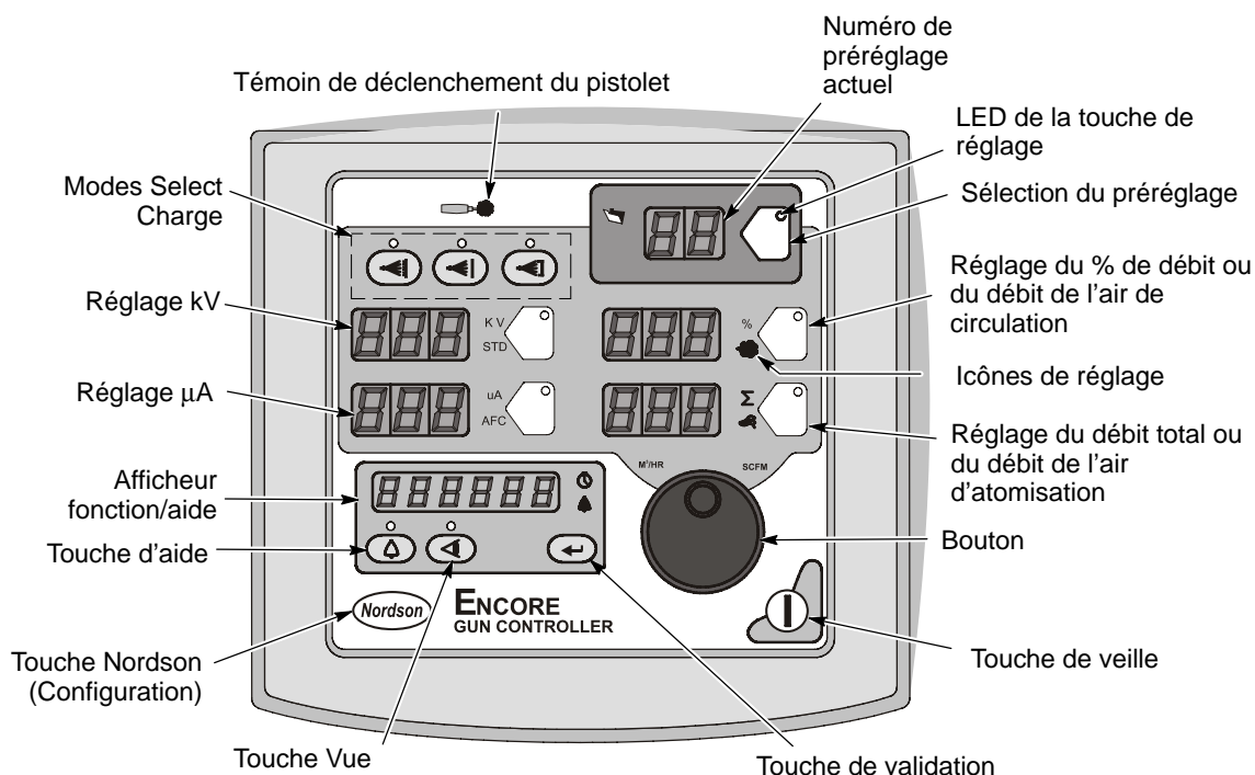
Fig. 3-7 Interface du contrôleur
