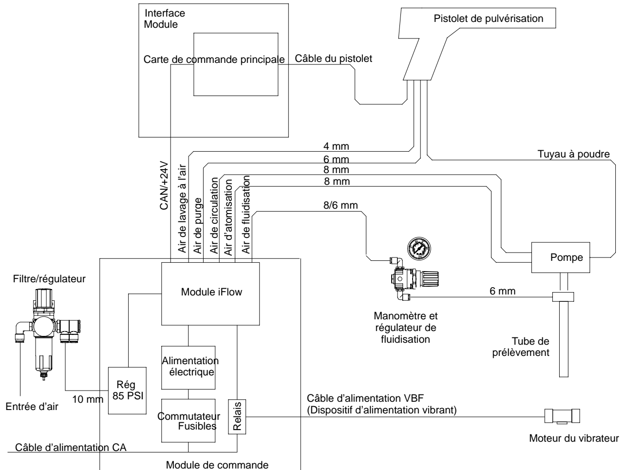
Fig. 2-2 Synoptique du système de poudrage manuel Encore
