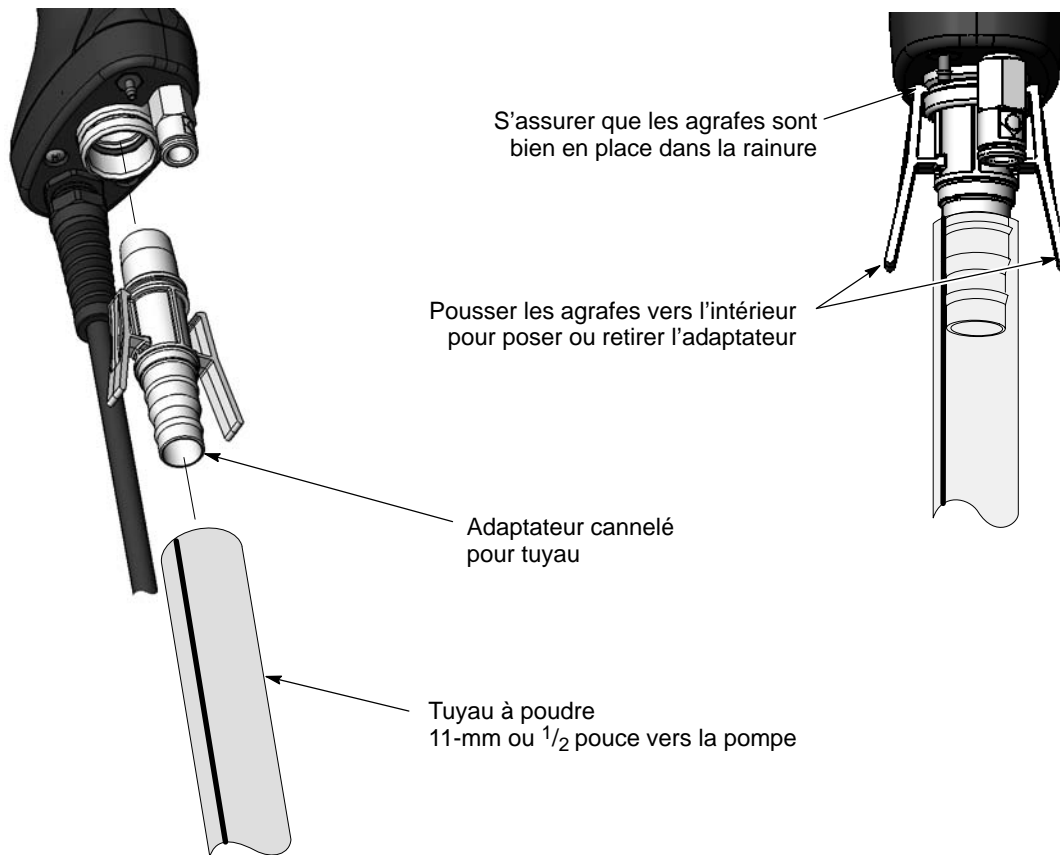
Fig. 2-10 Raccordement du tuyau à poudre au pistolet de pulvérisation
