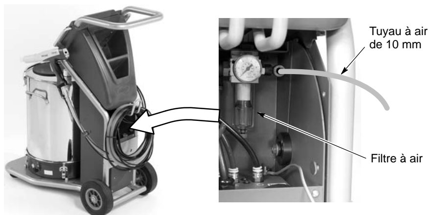
Fig. 2-11 Branchement de l'alimentation pneumatique du système
