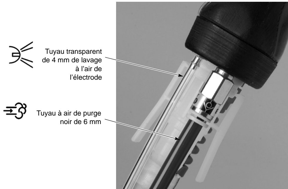
Fig. 2-8 Raccordement des tuyaux à poudre et à air au pistolet de pulvérisation
