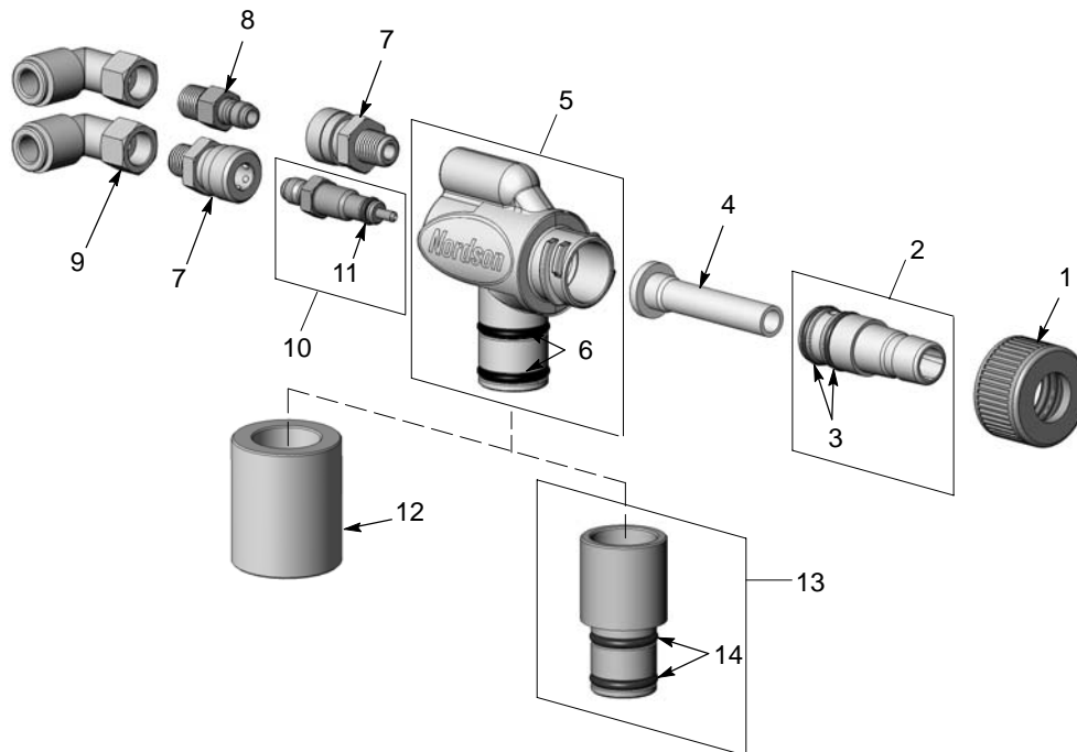
Fig. 6-9 Pièces de la pompe
