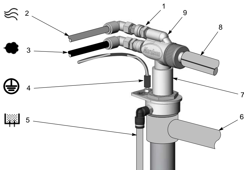
Fig. 2-6 Installation du tube de prélèvement et de la pompe
