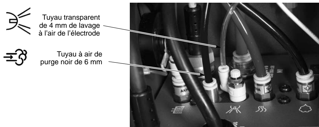
Fig. 2-9 Raccordement des tuyaux à air de pistolet et de purge au contrôleur
