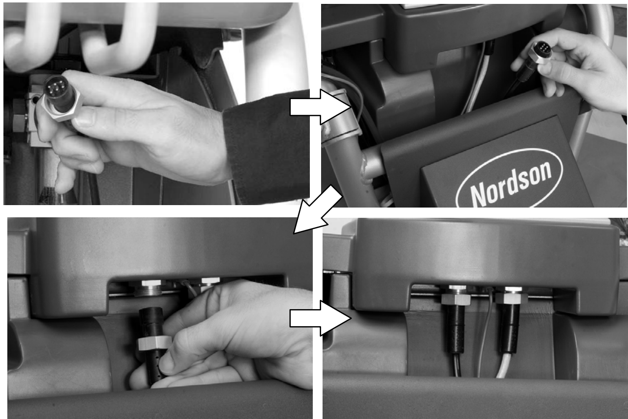
Fig. 2-7 Branchement du câble de pistolet au module d'interface du contrôleur
