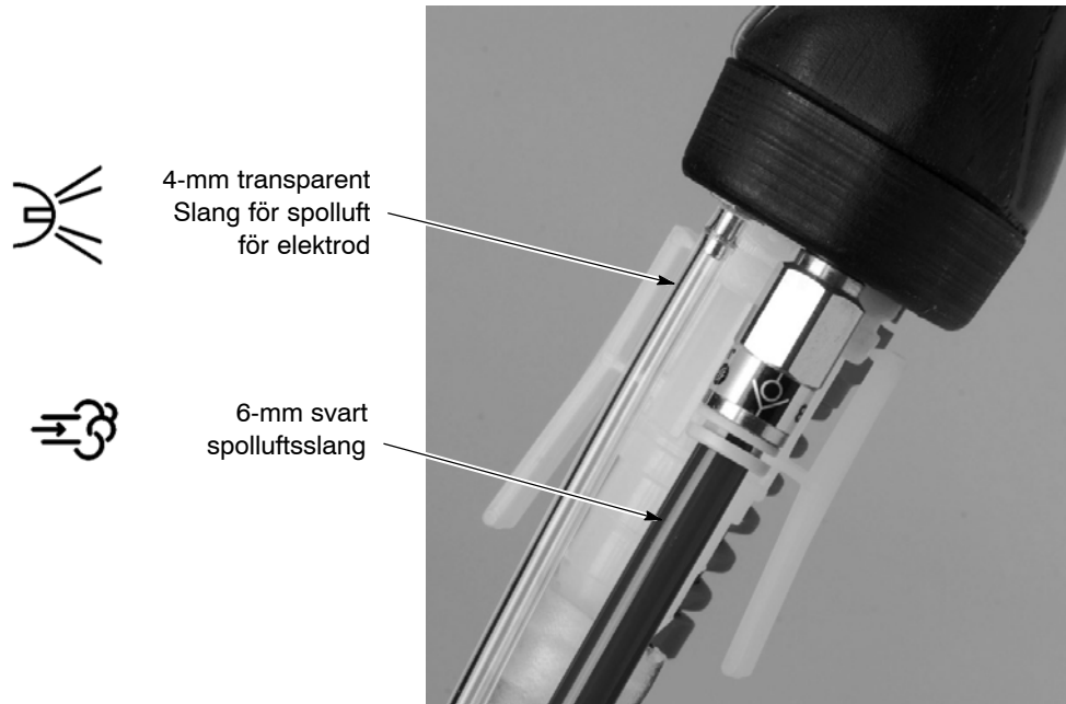
Bild 2-10 Anslutning av pulver- och luftslangar till spraypistolen
