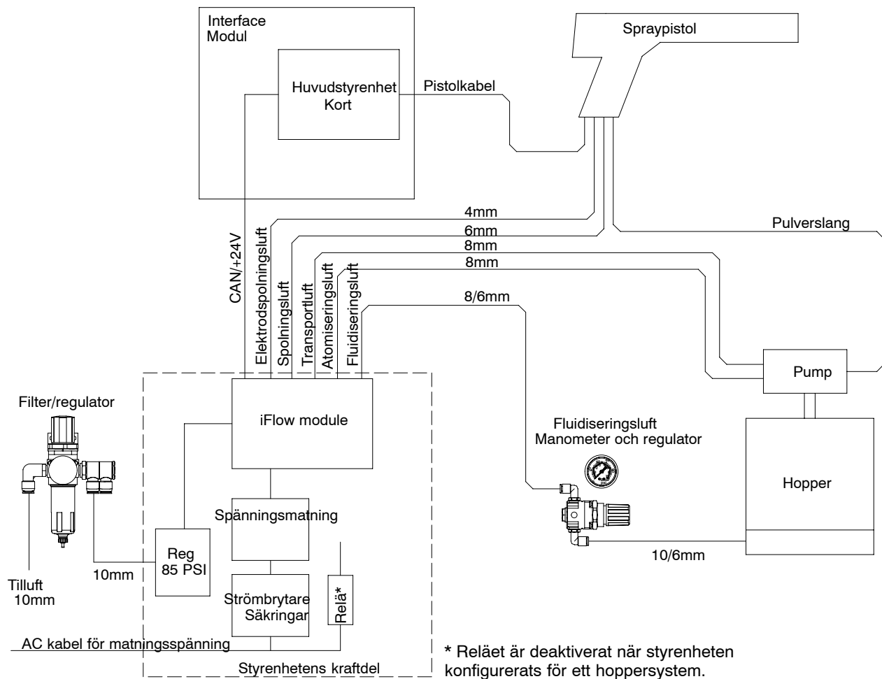
Bild 2-2 Blockschema för Encore manuellt pulverbeläggningssystem
