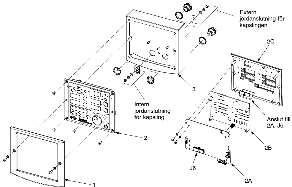
Bild 5-15 Interfacemodulsdelen
