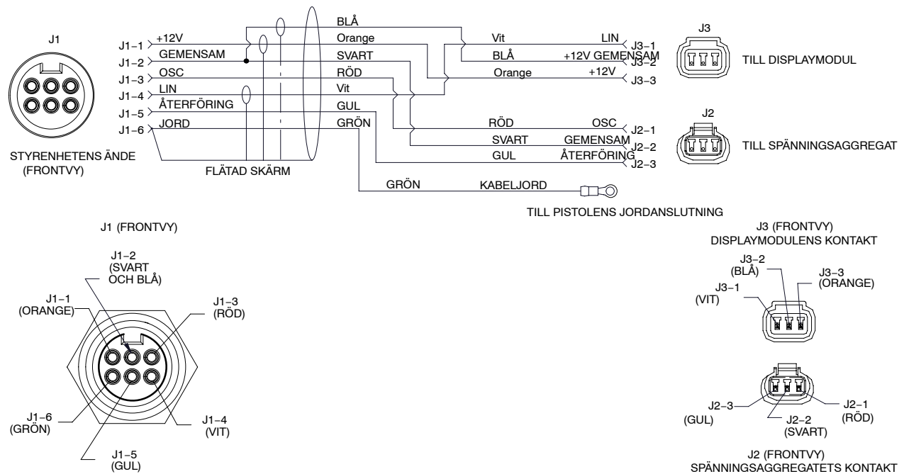
Bild 4-4 Pistolkabelanslutningar
