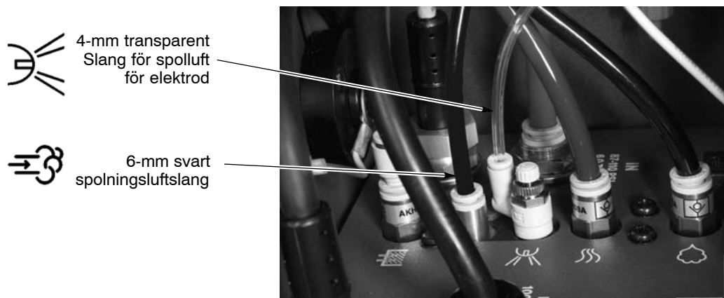
Bild 2-11 Anslutning av pistollufts- och spolningsluftslangar till styrenheten
