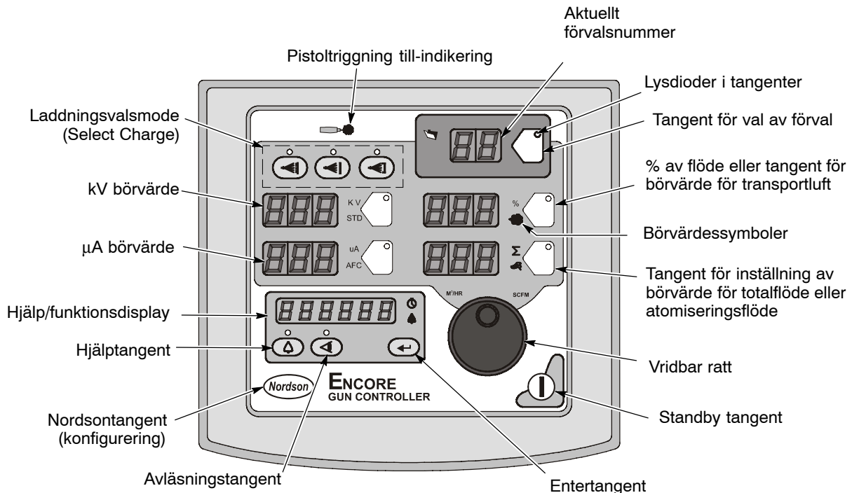
Bild 3-6 Styrenhetens interface
