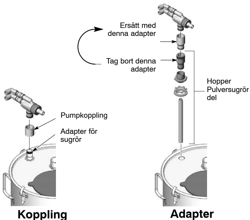
Bild 2-7 Pumpmontage
