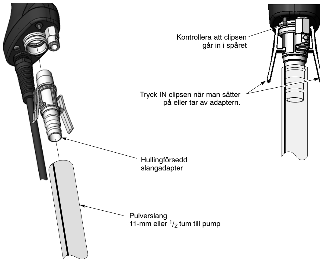
Bild 2-12 Anslutning av pulverslang till spraypistolen
