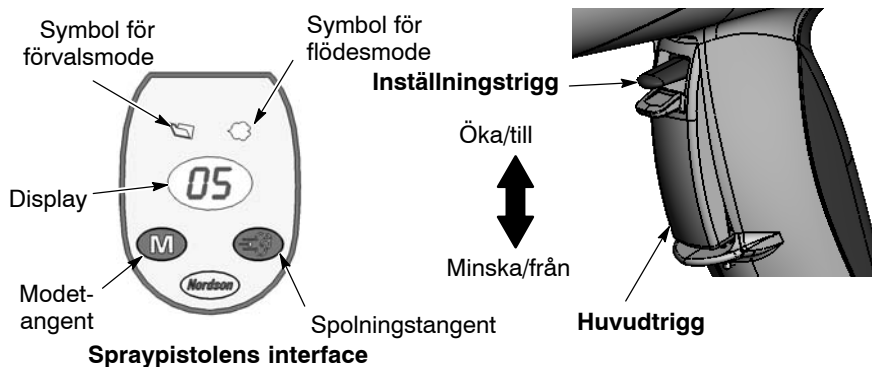
Bild 3-2 Pistolens inställningsorgan
