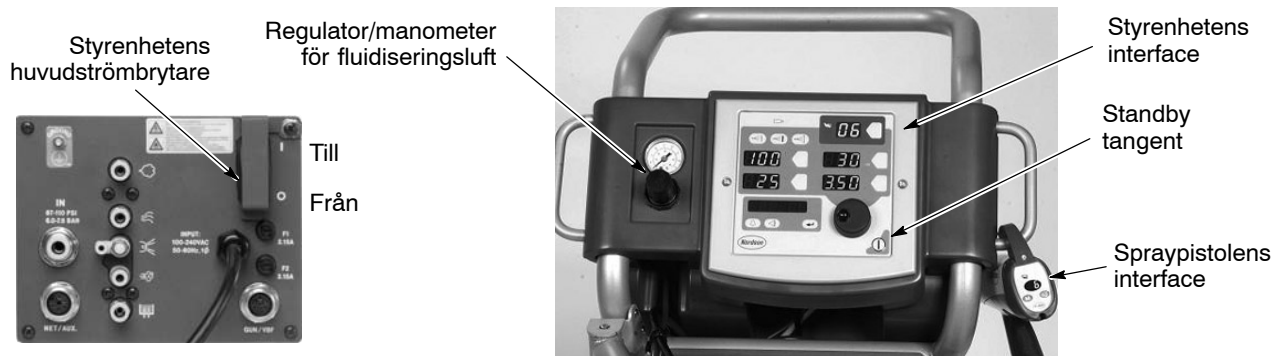
Bild 3-1 Systemets inställningsorgan
