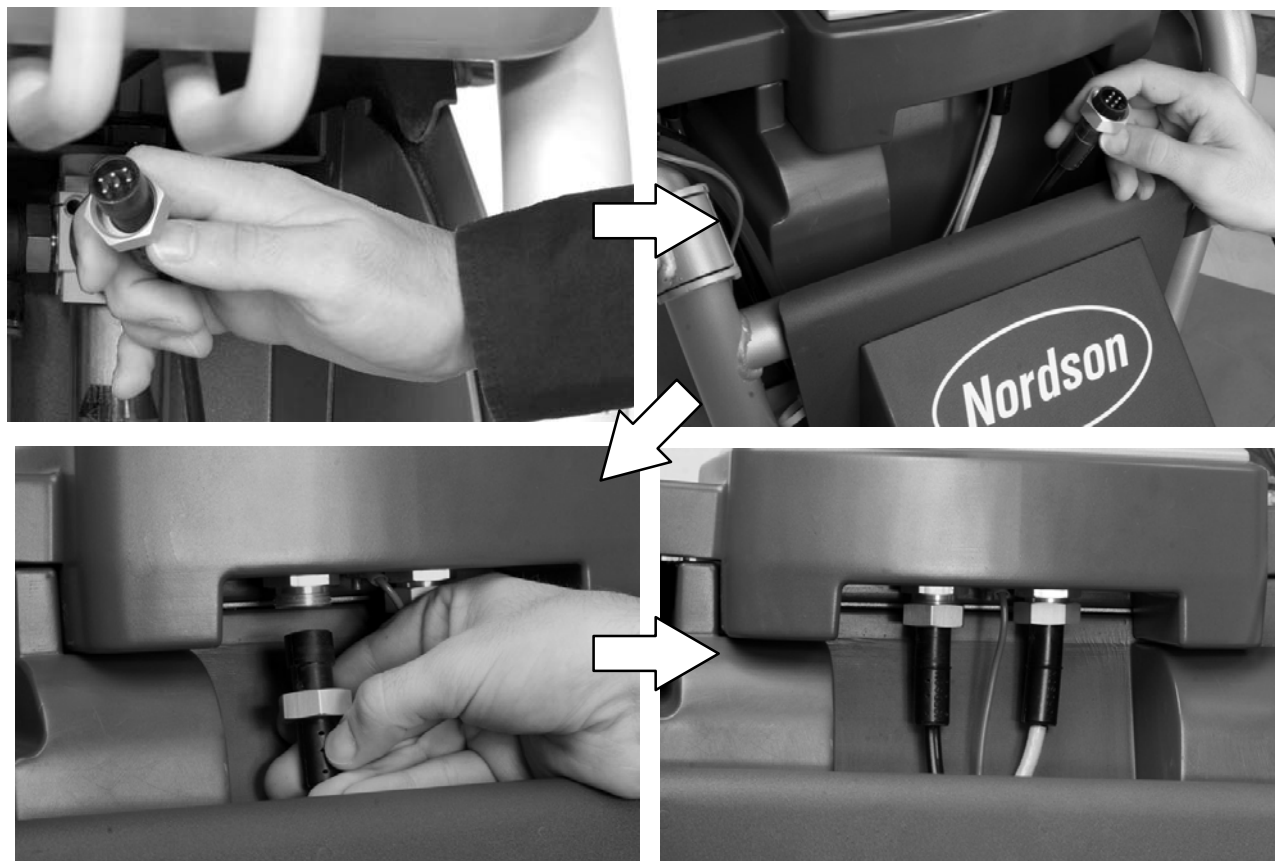
Bild 2-9 Anslutning av pistolkabeln till styrenhetens interfacemodul
