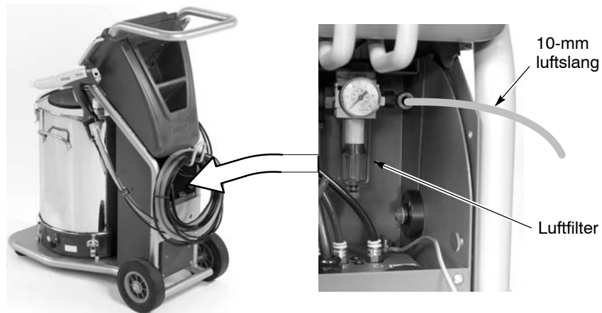
Bild 2-13 Luftförsörjning av systemet
