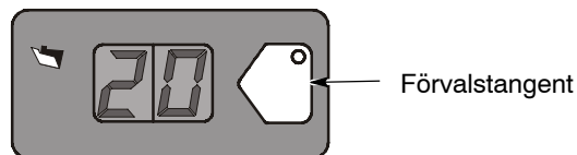
Bild 3-10 Välj förval
