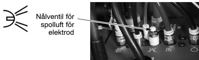
Bild 3-3 Placering av nålventil för spolluft för elektrod
