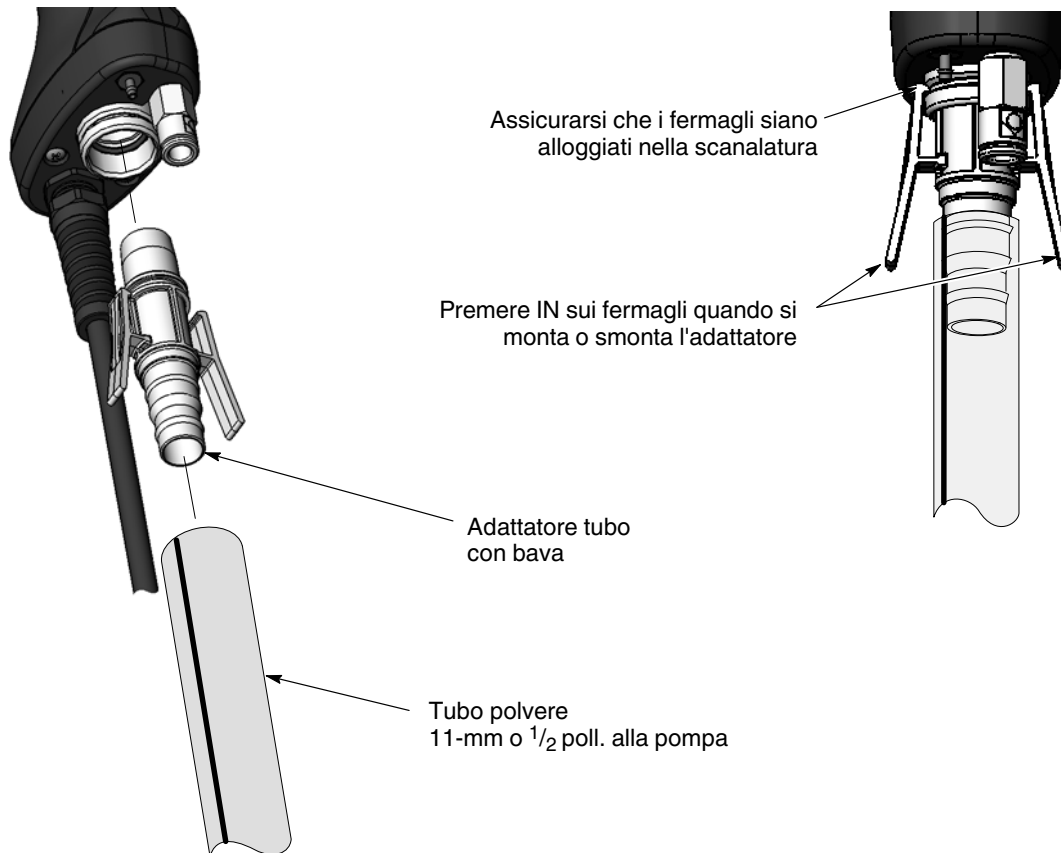
Fig. 2-10 Collegamento dei tubo della polvere alla pistola di spruzzo
