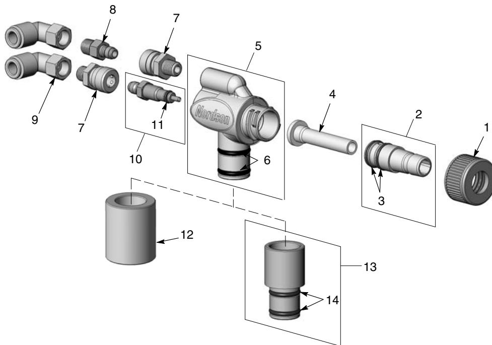
Fig. 6-9 Pezzi della pompa
