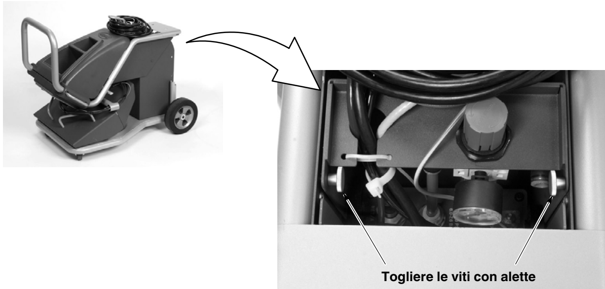
Fig. 2-4 Preparazione all'apertura della maniglia del carrello
