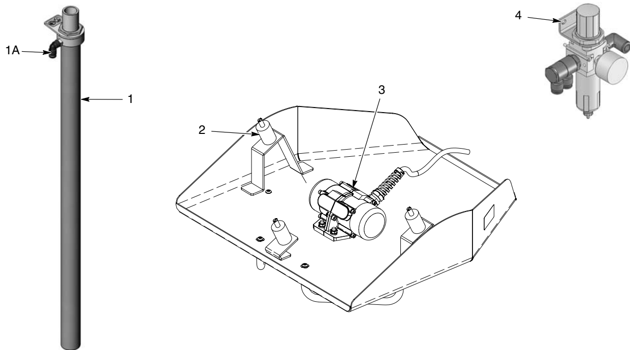
Fig. 6-8 Diversi pezzi del sistema
