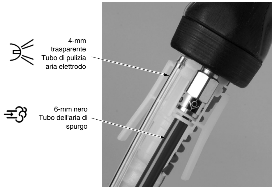
Fig. 2-8 Collegare i tubi della polvere e dell'aria alla pistola di spruzzo
