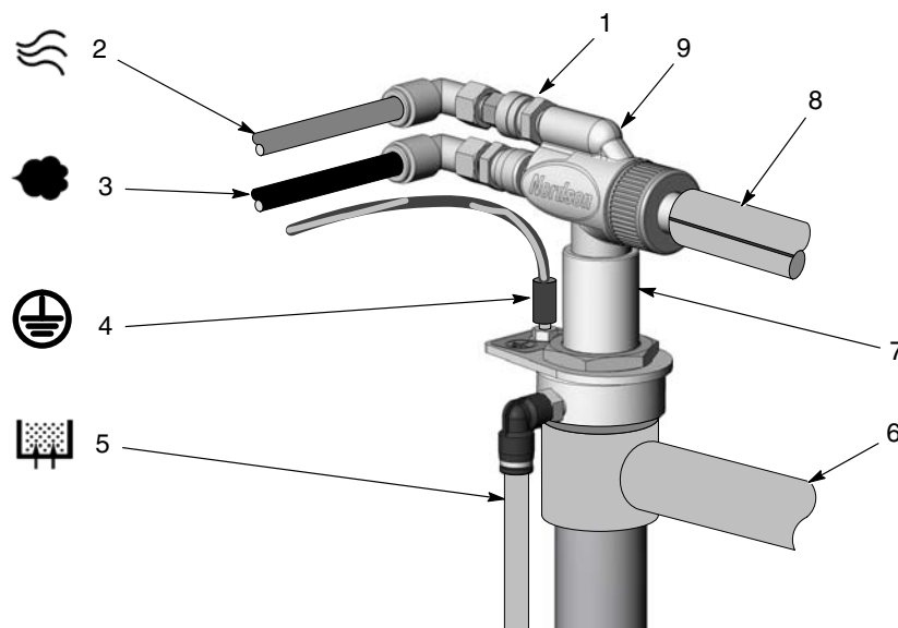
Fig. 2-6 Installazione del tubo di raccolta e della pompa
