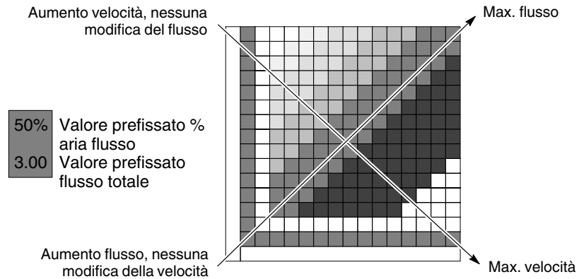
Fig. 3-17 Lettura delle tabelle di flusso intelligente
