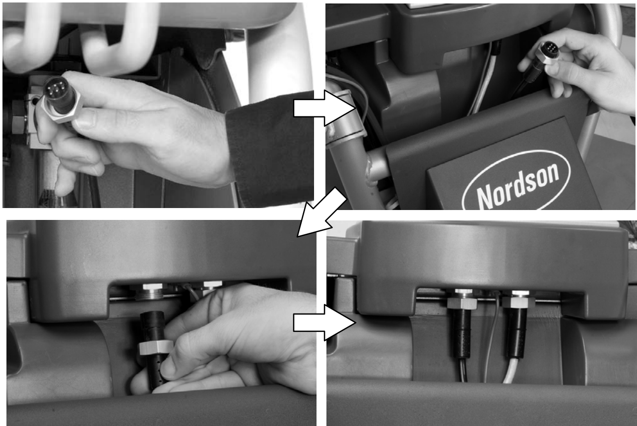
Fig. 2-7 Collegamento del cavo della pistola al modulo interfaccia controller
