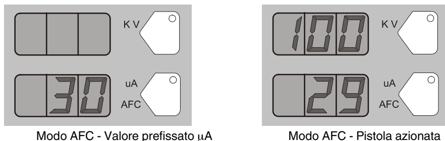
Fig. 3-15 Modo AFC - Visualizzazioni di valore prefissato e pistola azionata
