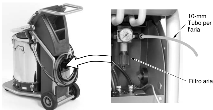
Fig. 2-11 Collegamento del rifornimento di aria al sistema
