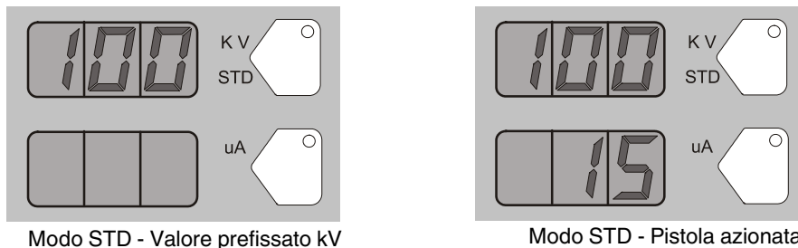
Fig. 3-14 Modo STD - Visualizzazioni di valore prefissato e pistola azionata
