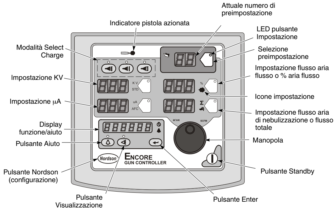
Fig. 3-7 Interfaccia del controller
