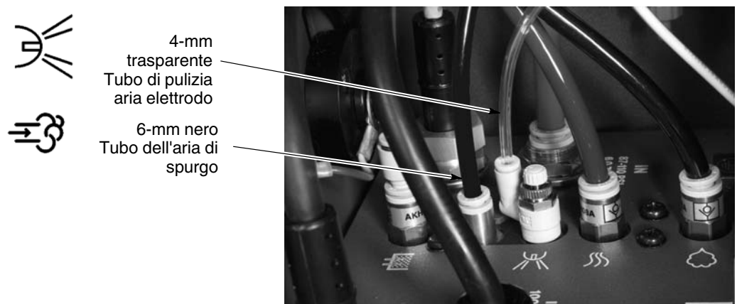
Fig. 2-9 Collegamento dei tubi dell'aria di spurgo e della pistola al controller
