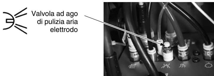
Fig. 3-4 Controllo dell'aria fluidizzante del sistema mobile
