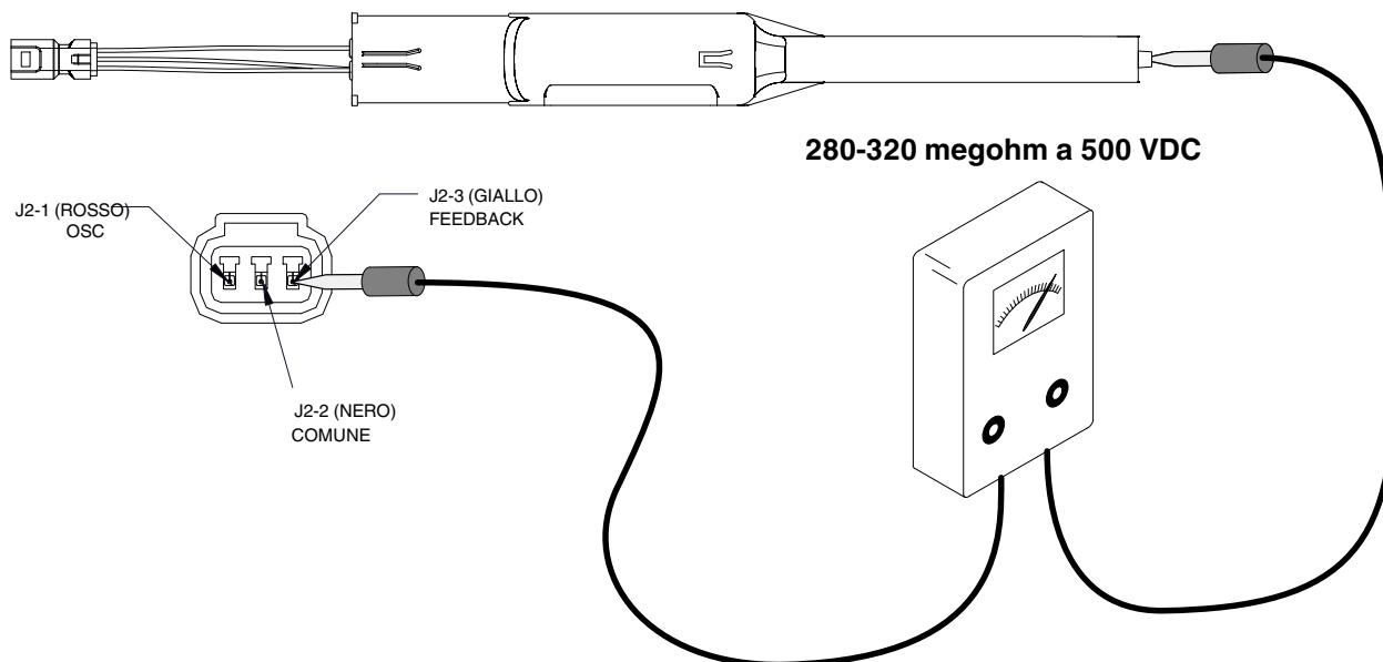
Fig. 4-2 Test di resistenza dell'alimentatore
