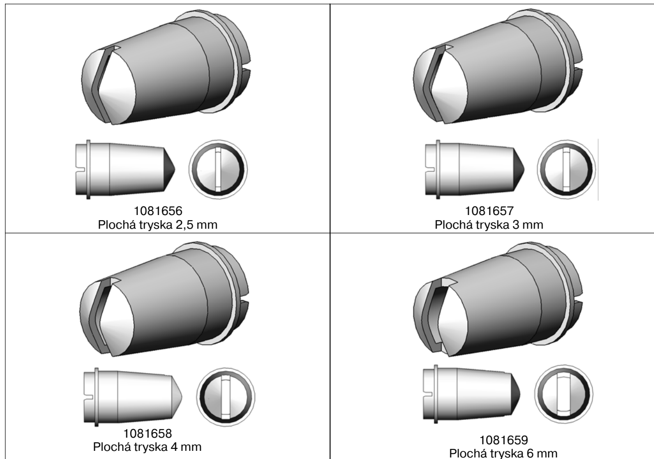
Obr. 6-2 Ploché trysky
