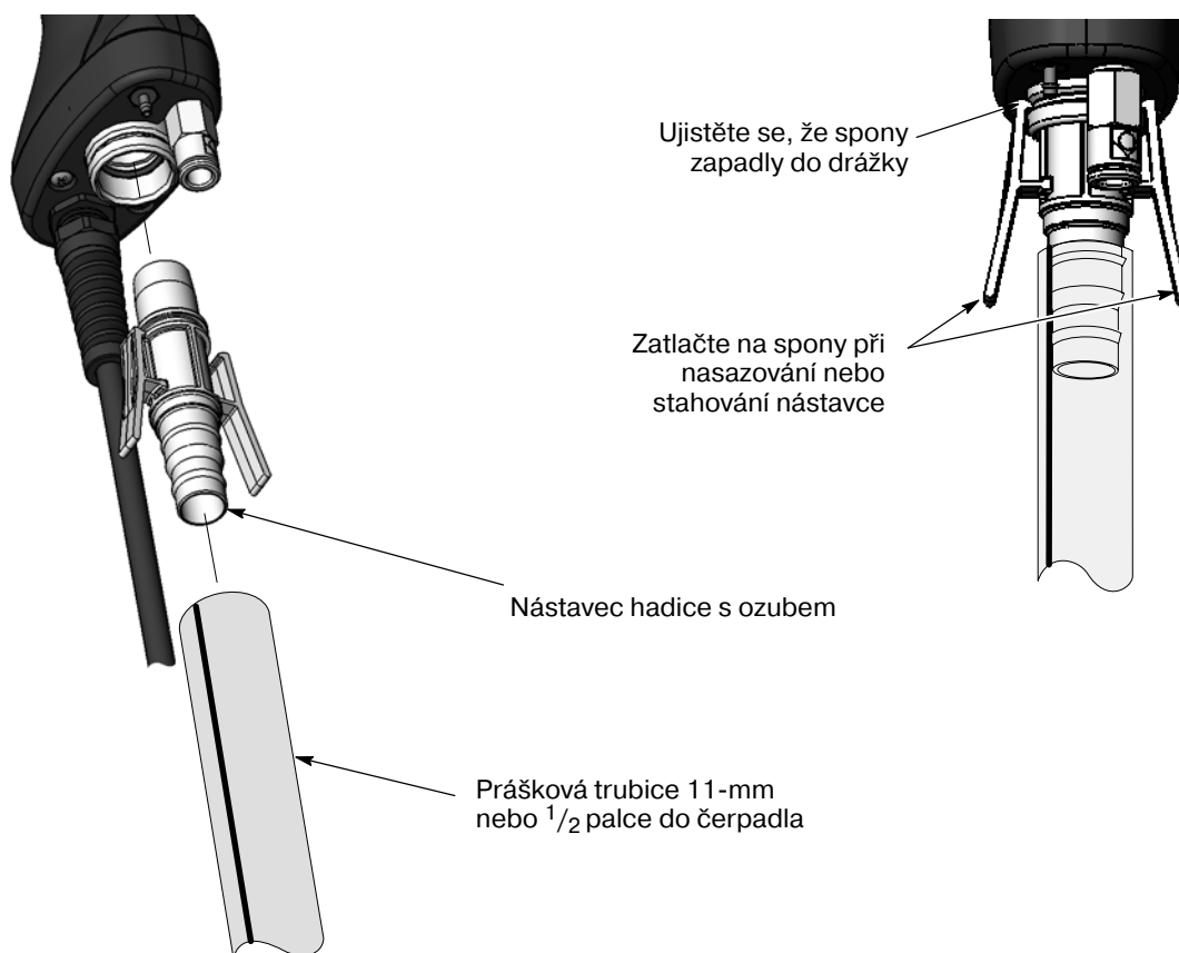
Obr. 2-10 Připojení práškové trubice ke stříkací pistoli
