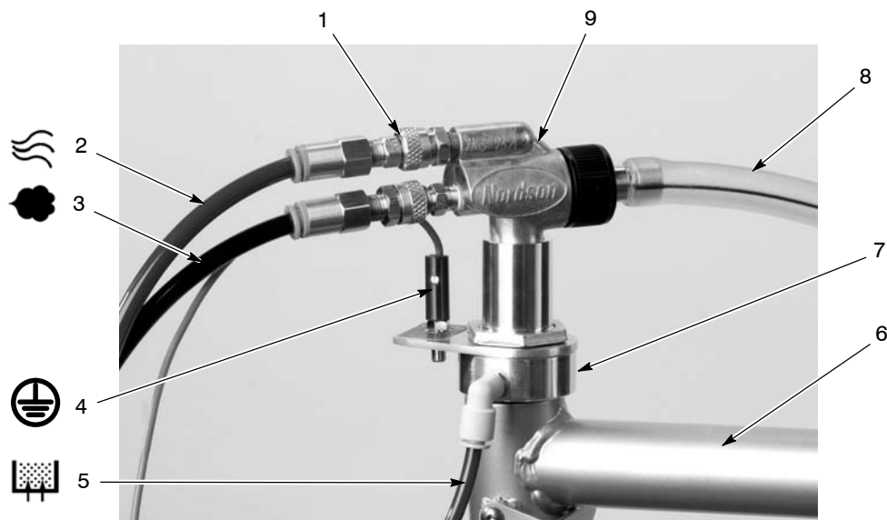
Obr. 2-6 Instalace sběrné trubice a čerpadla
