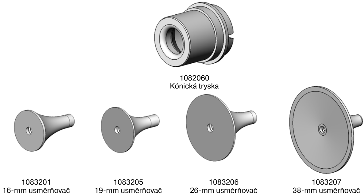
Obr. 6-3 Kónická tryska a usměrňovače
