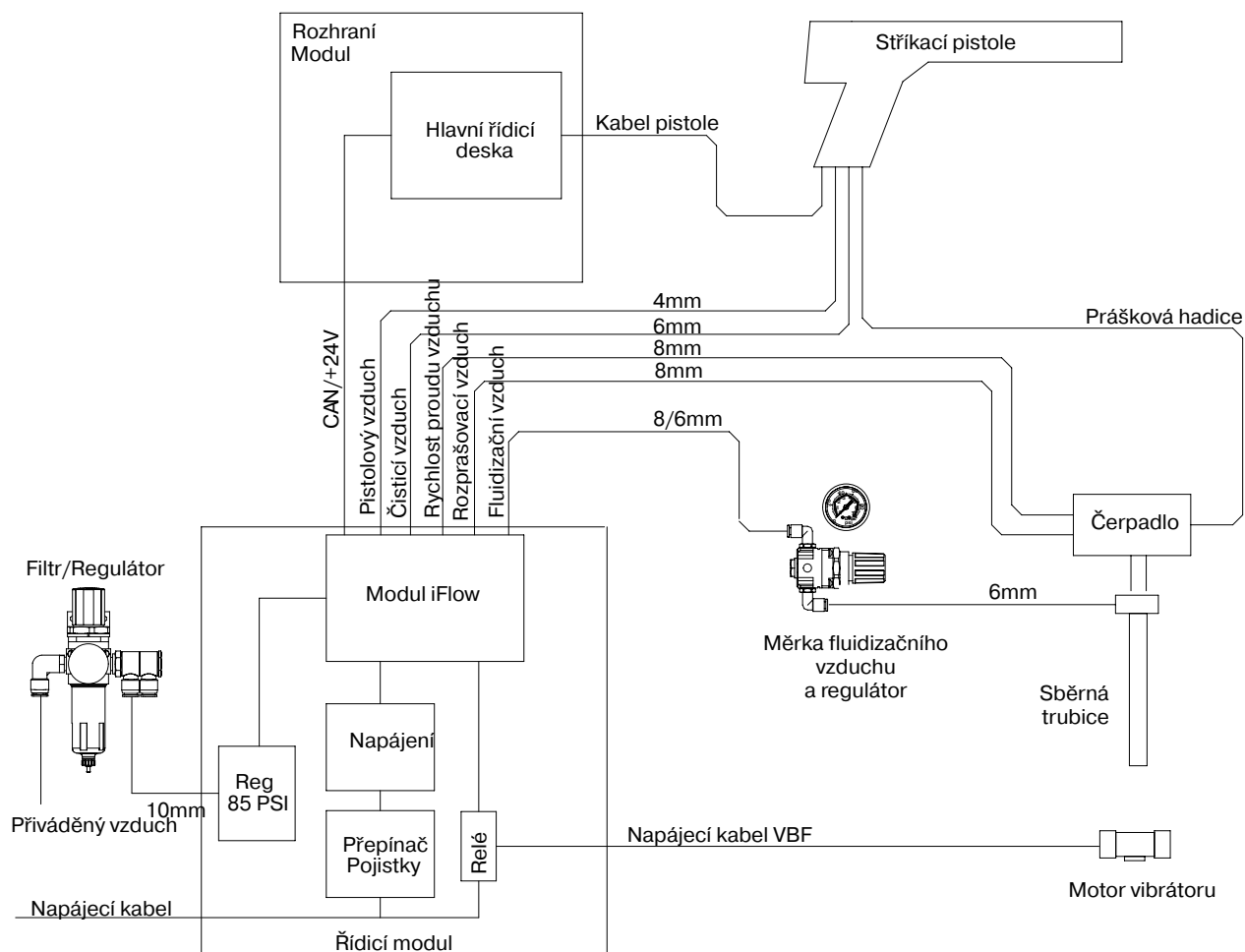
Obr. 2-2 Blokové schéma ručního práškového stříkáčního systému Encore
