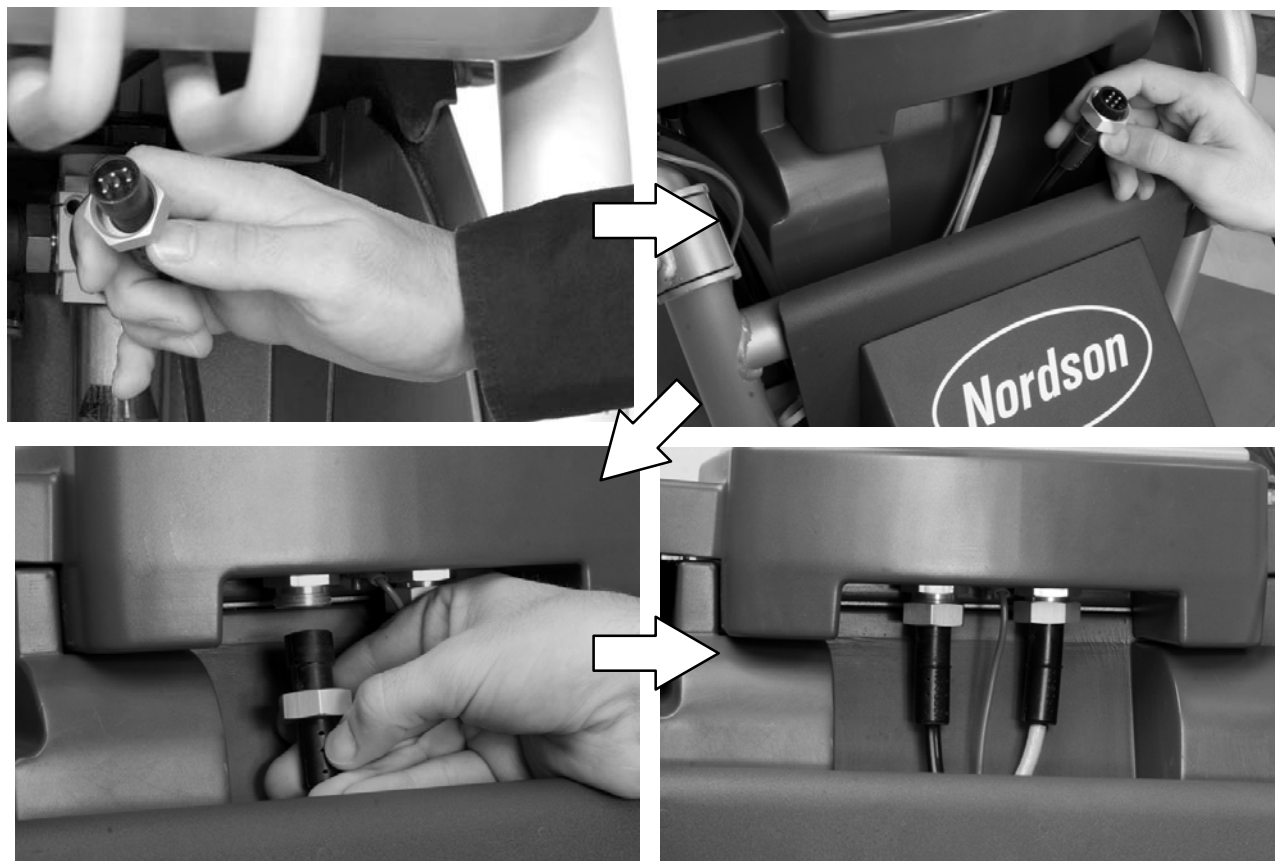
Obr. 2-7 Připojení kabelu pistole na modul rozhraní řídicí jednotky
