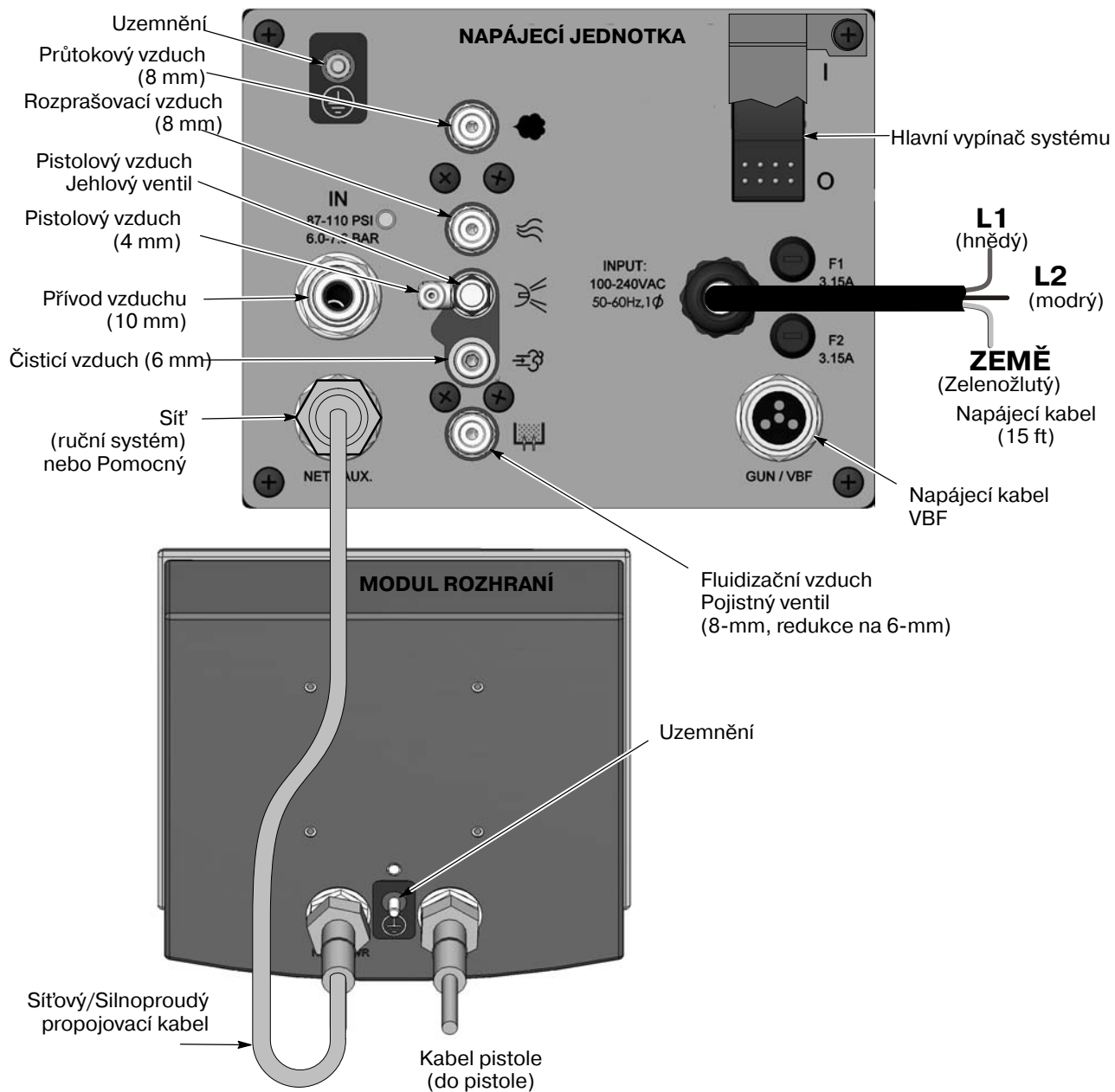
Obr. 2-3 Připojení řídicí jednotky pistole Encore
