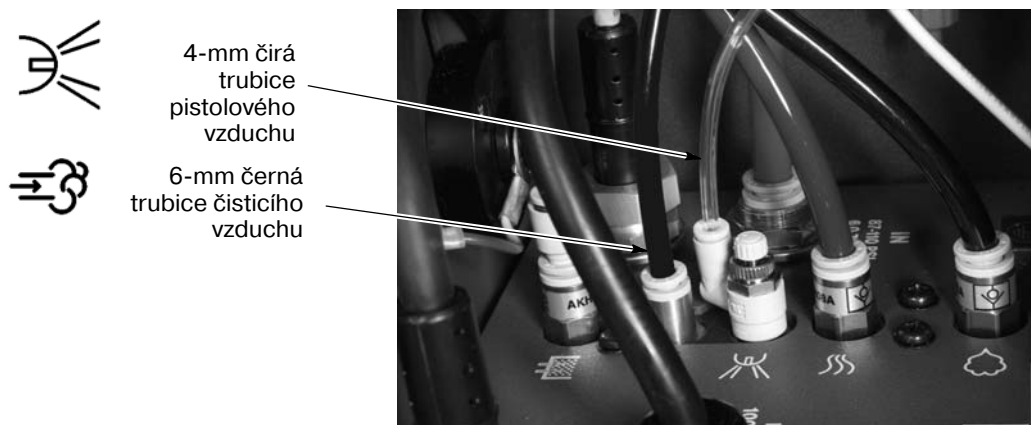
Obr. 2-9 Připojení trubice pistolového vzduchu a čistícího vzduchu k řídicí jednotce
