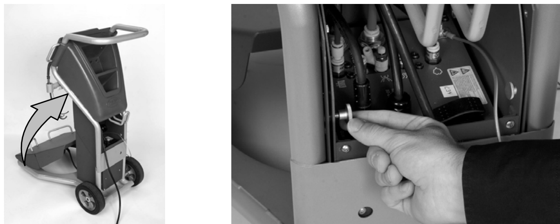
Obr. 2-5 Rozložení madla vozíku a jeho zajištění na místě
