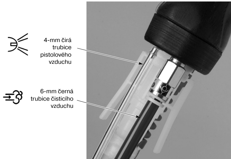
Obr. 2-8 Připojení práškové trubice a trubic pro přívod vzduchu ke stříkací pistoli
