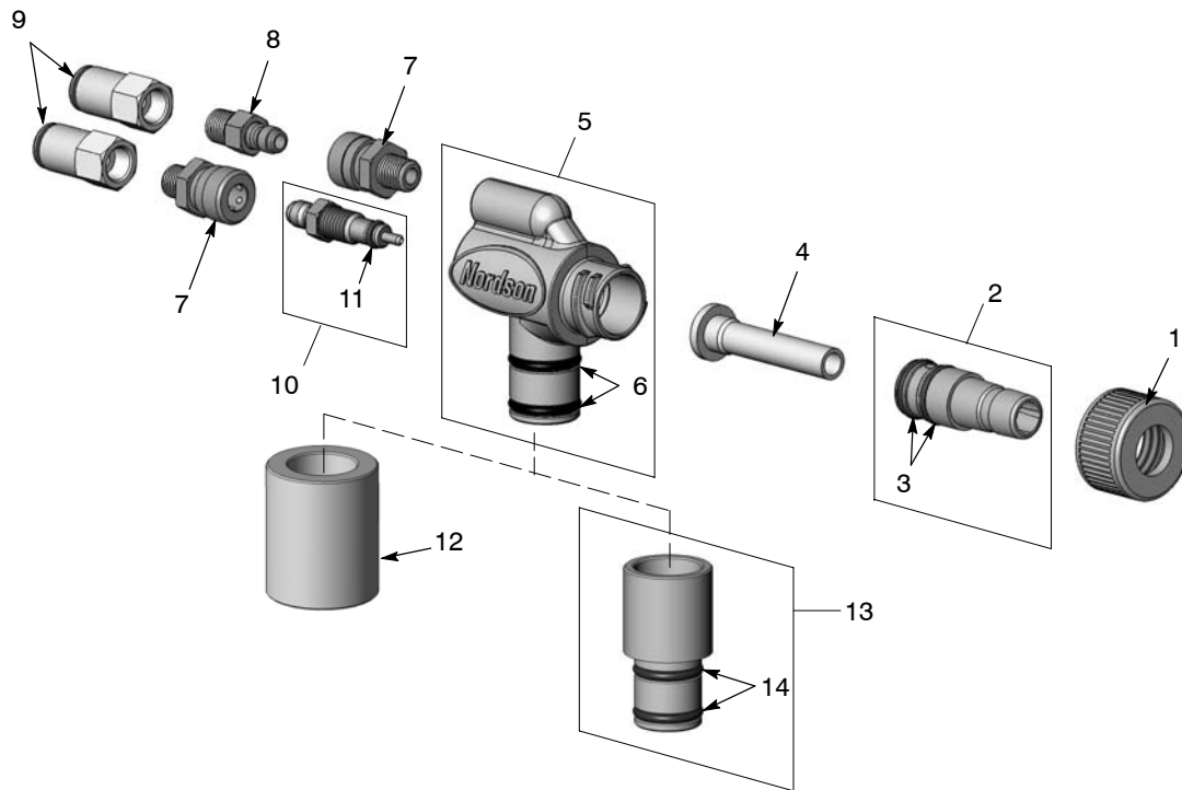
Obr. 6-9 Části čerpadla
