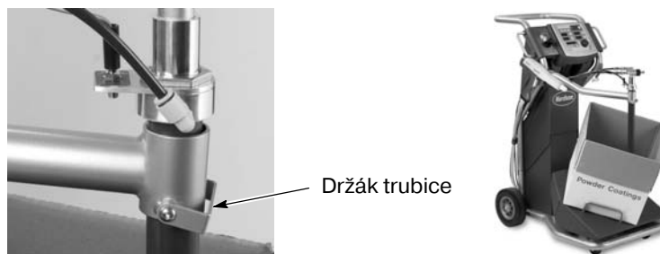
Obr. 3-3 Instalace krabice s práškem
