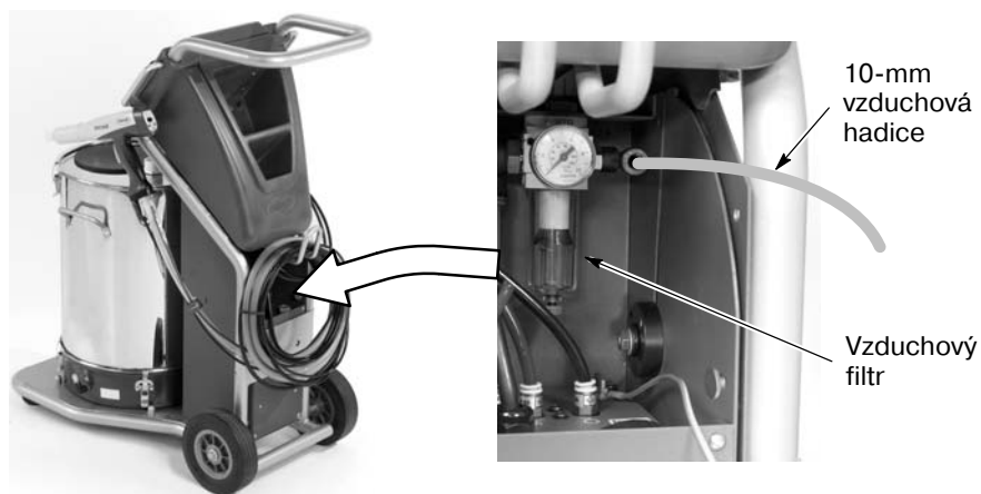
Obr. 2-11 Připojení přívodu vzduchu do systému
