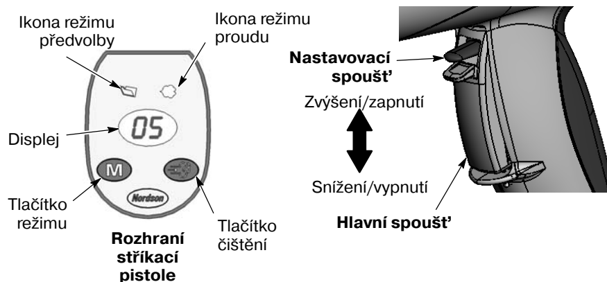
Obr. 3-2 Ovládací prvky pistole
