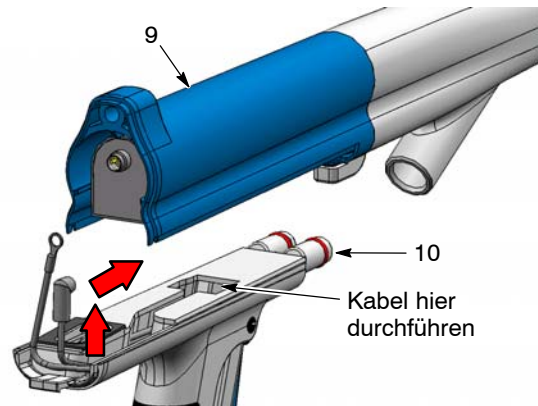
Abb. 4 Gehäuse vom Griff trennen und Kabel abnehmen
