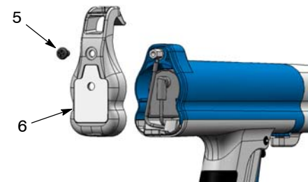
Abb. 2 Abschlusskappe abnehmen
