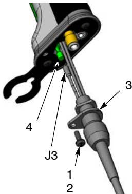
Abb. 1 Pistolenkabel von Griff und Auslöserschalter abnehmen
