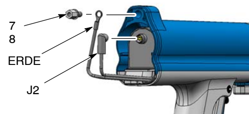
Abb. 3 Spannungsvervielfacherstecker und Erdungsleiter abnehmen
