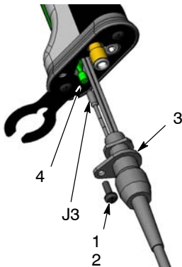
Bild 1 Urkoppling av pistolkabel från handtaget och triggkontakten
