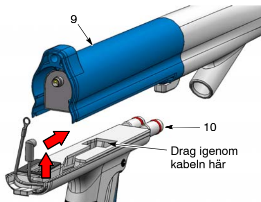
Bild 4 Delning av pistolkropp och handtag och demontering av kabel
