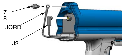
Bild 3 Demontering av multiplikatorkontakt och jordkabel
