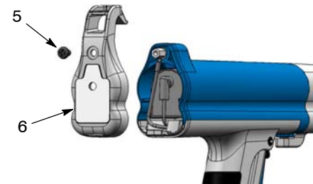
Bild 2 Demontering av lock över pistolände.
