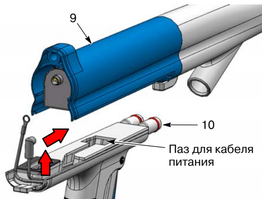
Рис. 4 Отсоединение корпуса от рукоятки распылителя и извлечение кабеля
