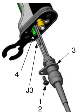
Рис. 1 Отсоединение кабеля распылителя от рукоятки и выключателя спускового крючка
