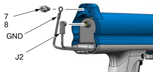
Рис. 3 Отсоединение разъема умножителя и провода заземления
