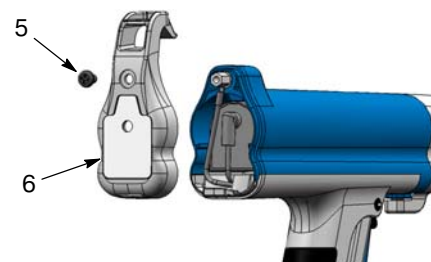
Рис. 2 Снятие крышки
