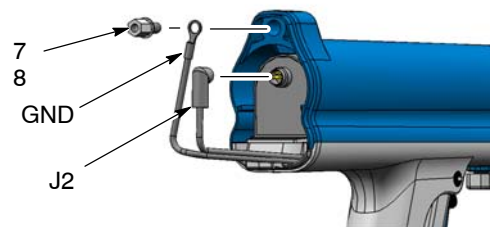
Slika 3 Odstranjevanje priključka množilnika in ozemljitvene žice
