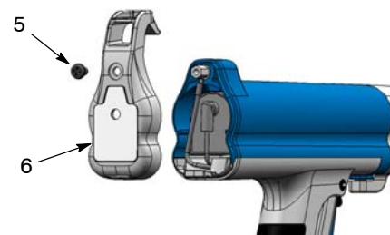
Slika 2 Odstranjevanje končnega pokrova
