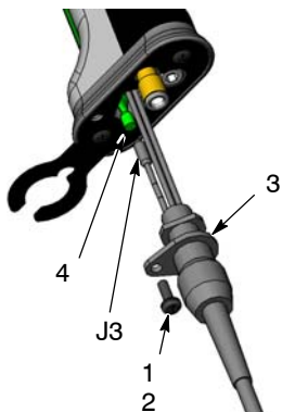
Slika 1 Odklapljanje kabla pištole iz ročaja in stikala sprožilca
