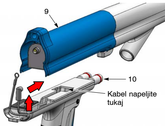
Slika 4 Ločevanje telesa z ročaja in odstranjevanje kabla
