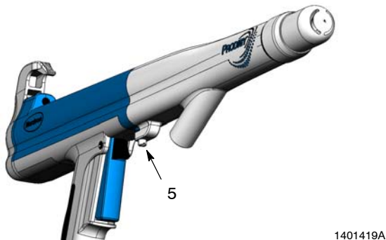
Slika 2 Odvijanje nastavljalnega vijaka prilagodilnika
