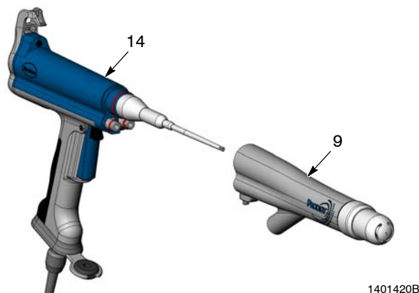
Slika 3 Odstranjevanje prilagodilnika
