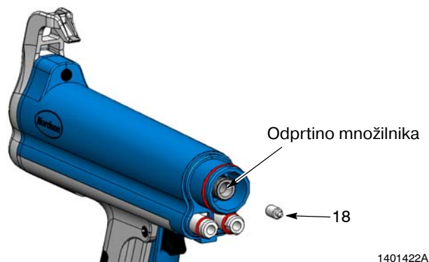
Slika 5 Odstranjevanje kontaktne podložke
