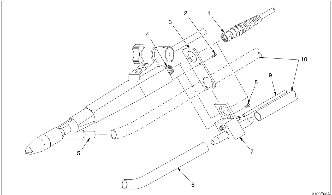
Afb. 2 Installeren van een diffusor
