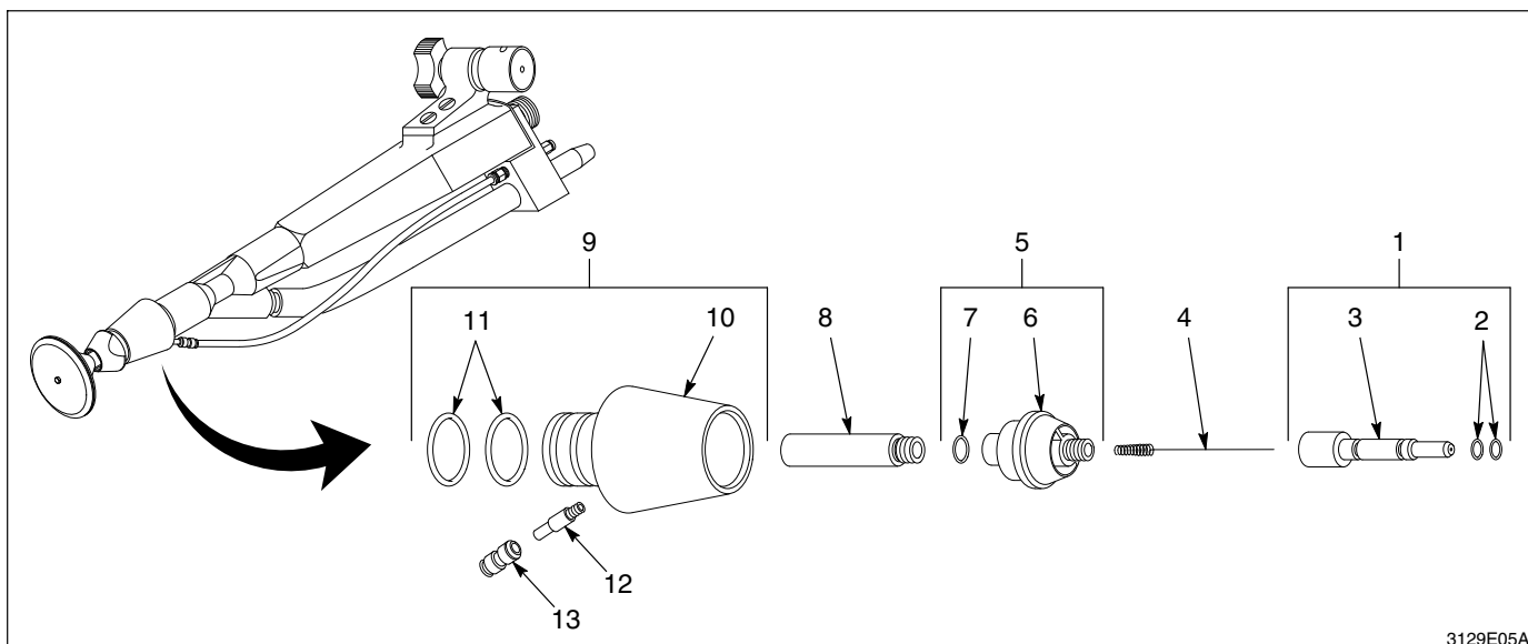
Afb. 6 Grote conische patroonspuitmondextensie
