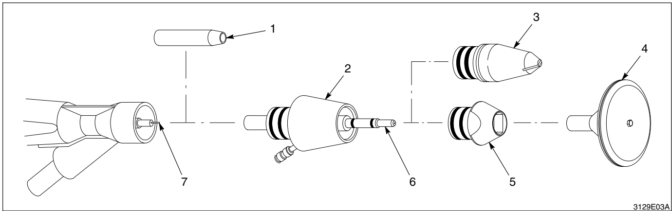
Afb. 3 Installeren van een grote conische patroonspuitmondextensie
