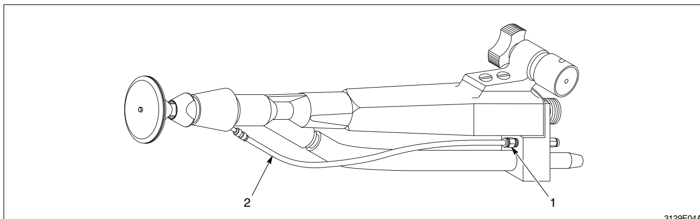
Afb. 4 Aansluiten van de luchtslang
