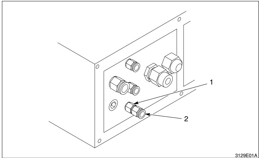
Afb. 1 Installeren van de luchtweerstand en de slangkoppeling
