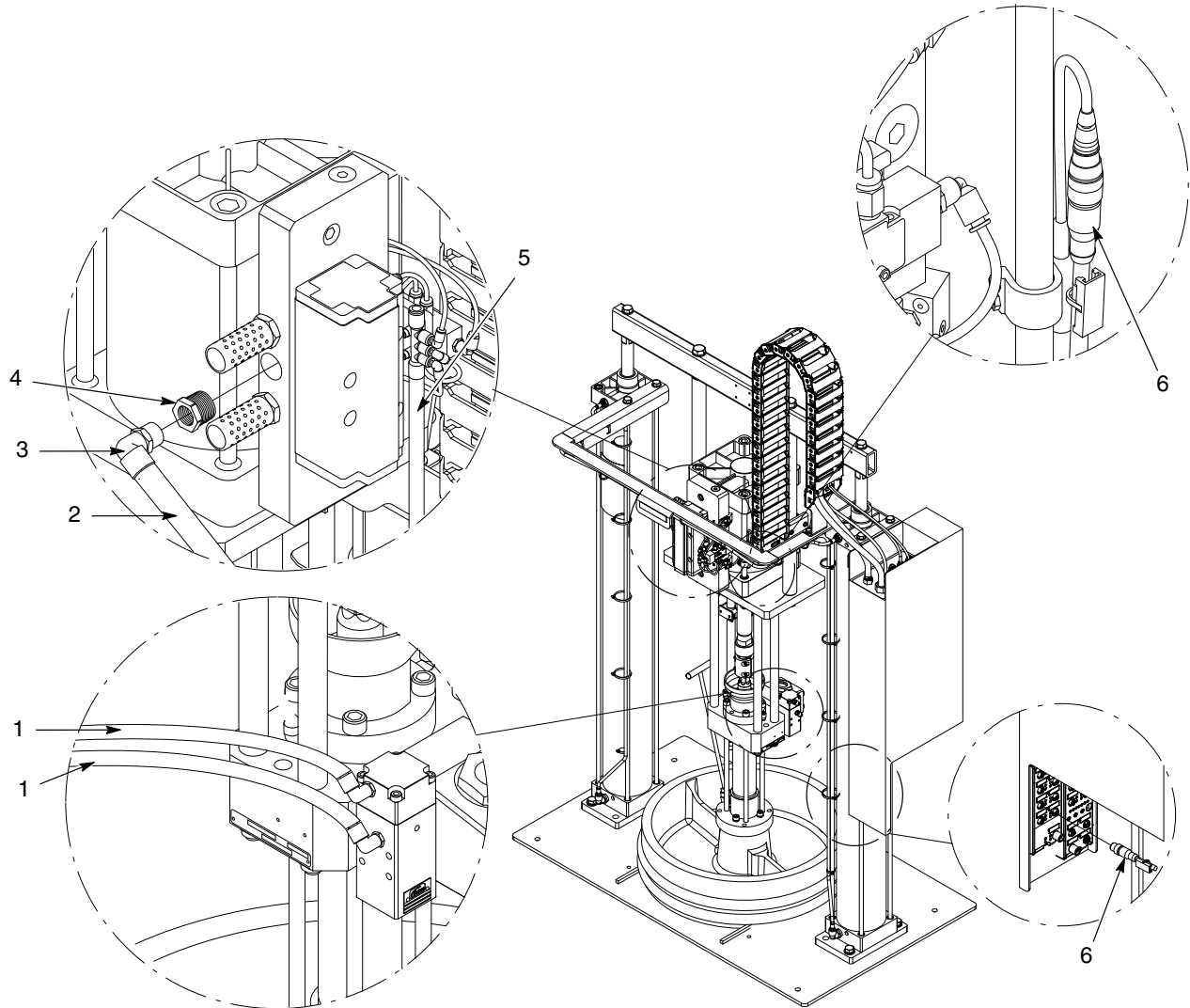
Obr. 15 Modul hadice s malým/veľkým rámom so vzduchovým motorom SD3, MT, 24 V DC (2 z 2)
