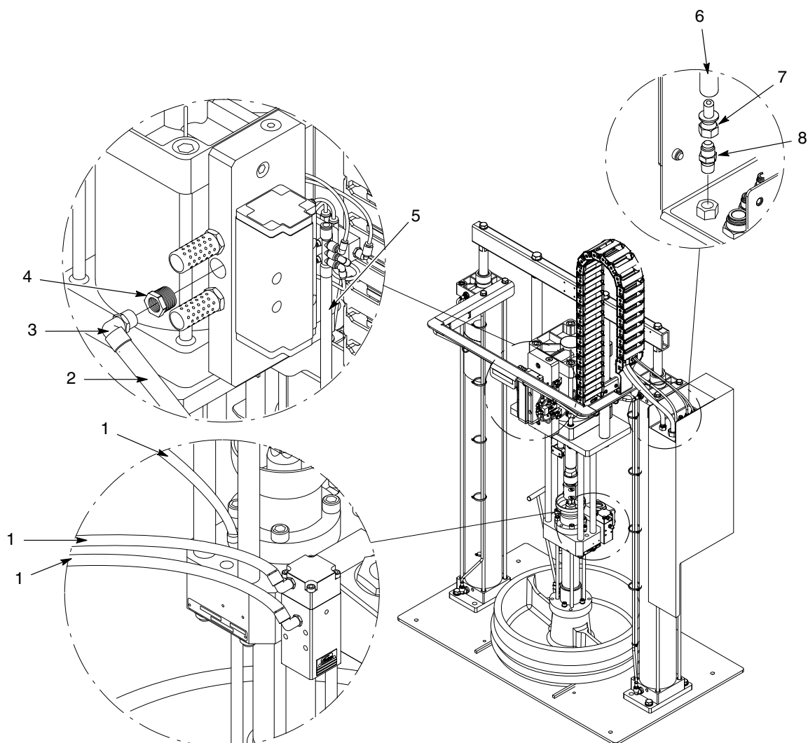
Obr. 9 Modul hadice s malým/veľkým rámom so vzduchovým motorom SD3, 24 V DC (2 z 3)
