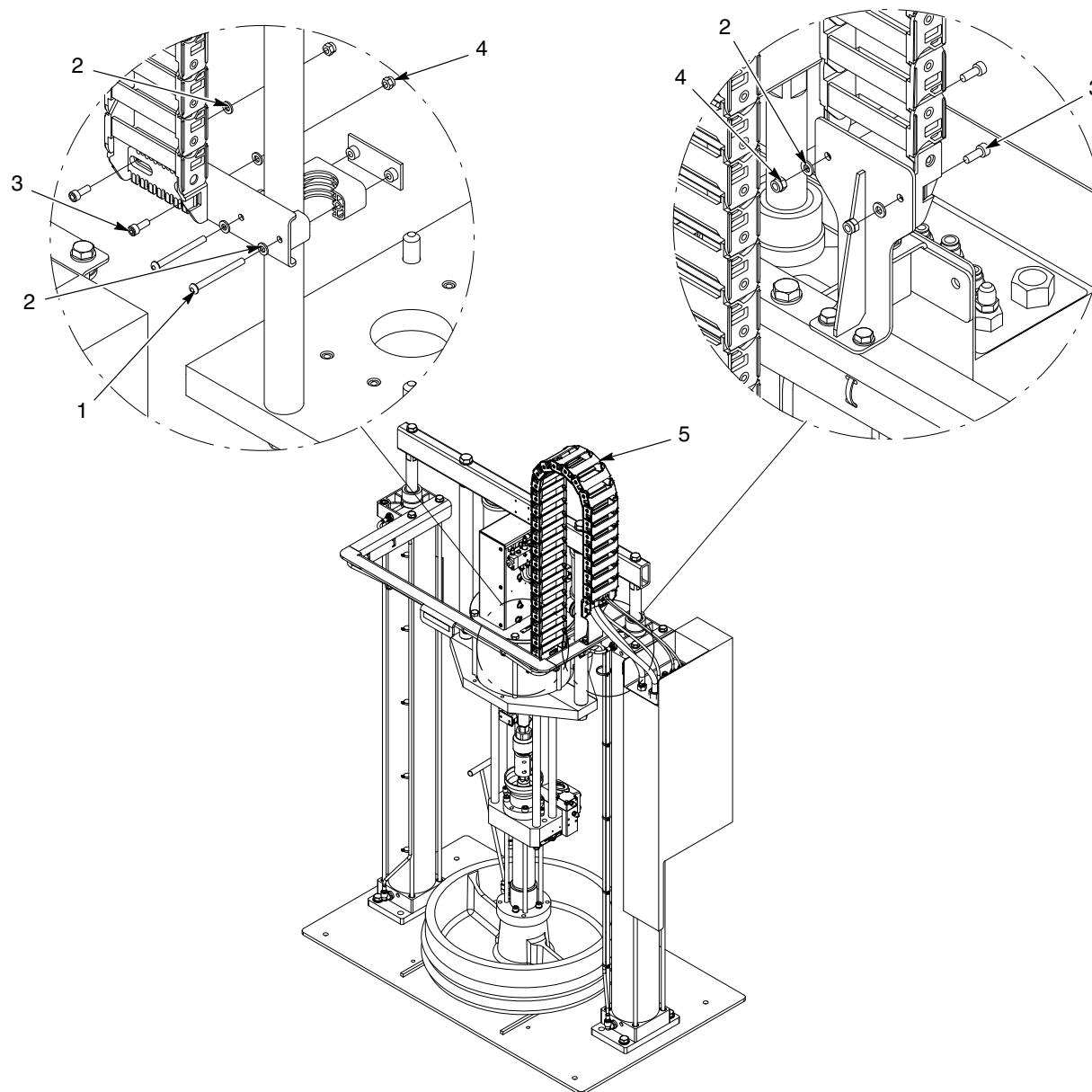
Obr. 11 Modul hadice s malým/velkým rámom so vzduchovým motorom SD2, 24 V DC (1 z 3)
