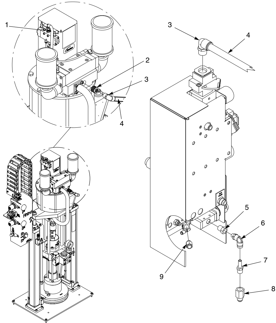
Obr. 21 Modul hadice s rámom DP so vzduchovým motorom SD2, pneumatický (2 z 2)
