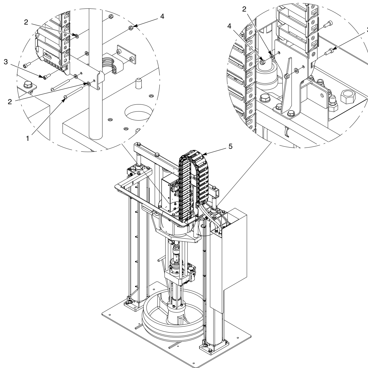
Obr. 16 Modul hadice s malým/velkým rámom so vzduchovým motorom SD2, MT, 24 V DC (1 z 2)
