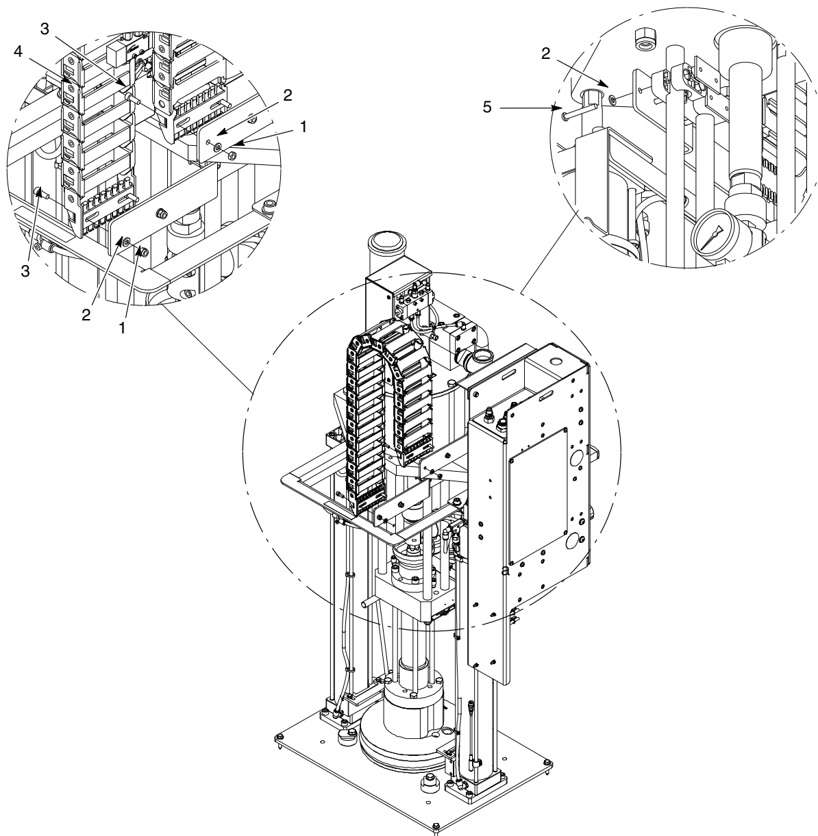
Obr. 7 Modul hadice s rámom DP so vzduchovým motorom SD2, 24 V DC (2 z 2)
