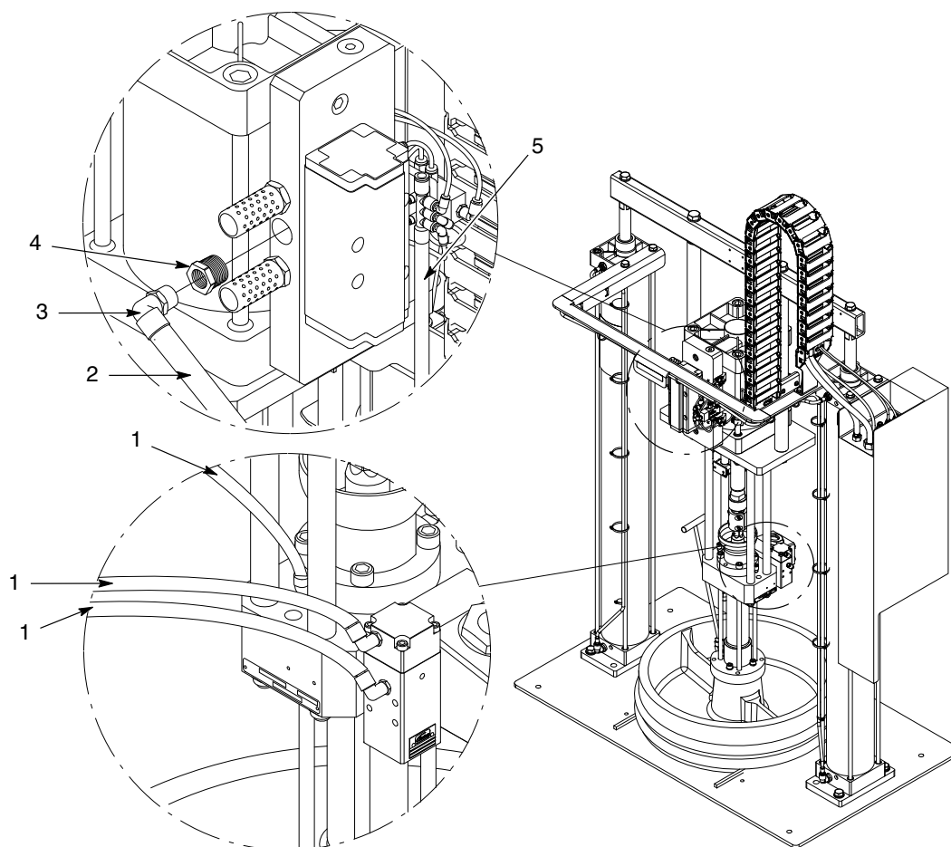
Obr. 12 Modul hadice s malým/veľkým rámom so vzduchovým motorom SD2, 24 V DC (2 z 3)
