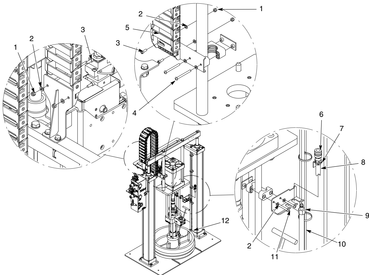
Obr. 24 Modul hadice s malým/velkým rámom so vzduchovým motorom SD2, 5-gal. A 55-gal., pneumatický (1 z 2)
