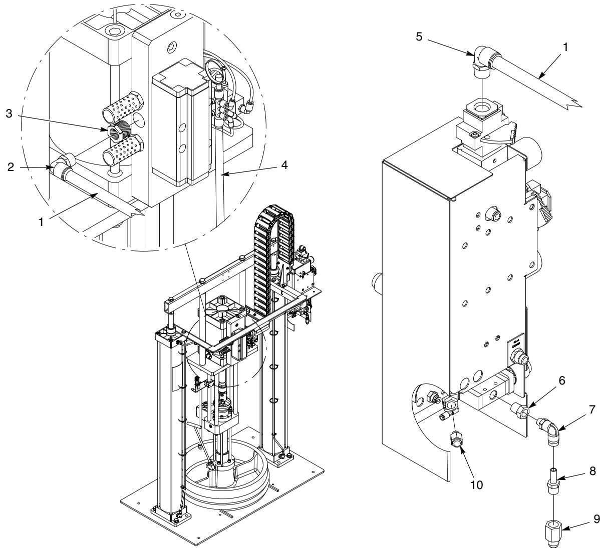
Obr. 23 Modul hadice s malým/veľkým rámom so vzduchovým motorom SD3, 55-gal., pneumatický (2 z 2)
