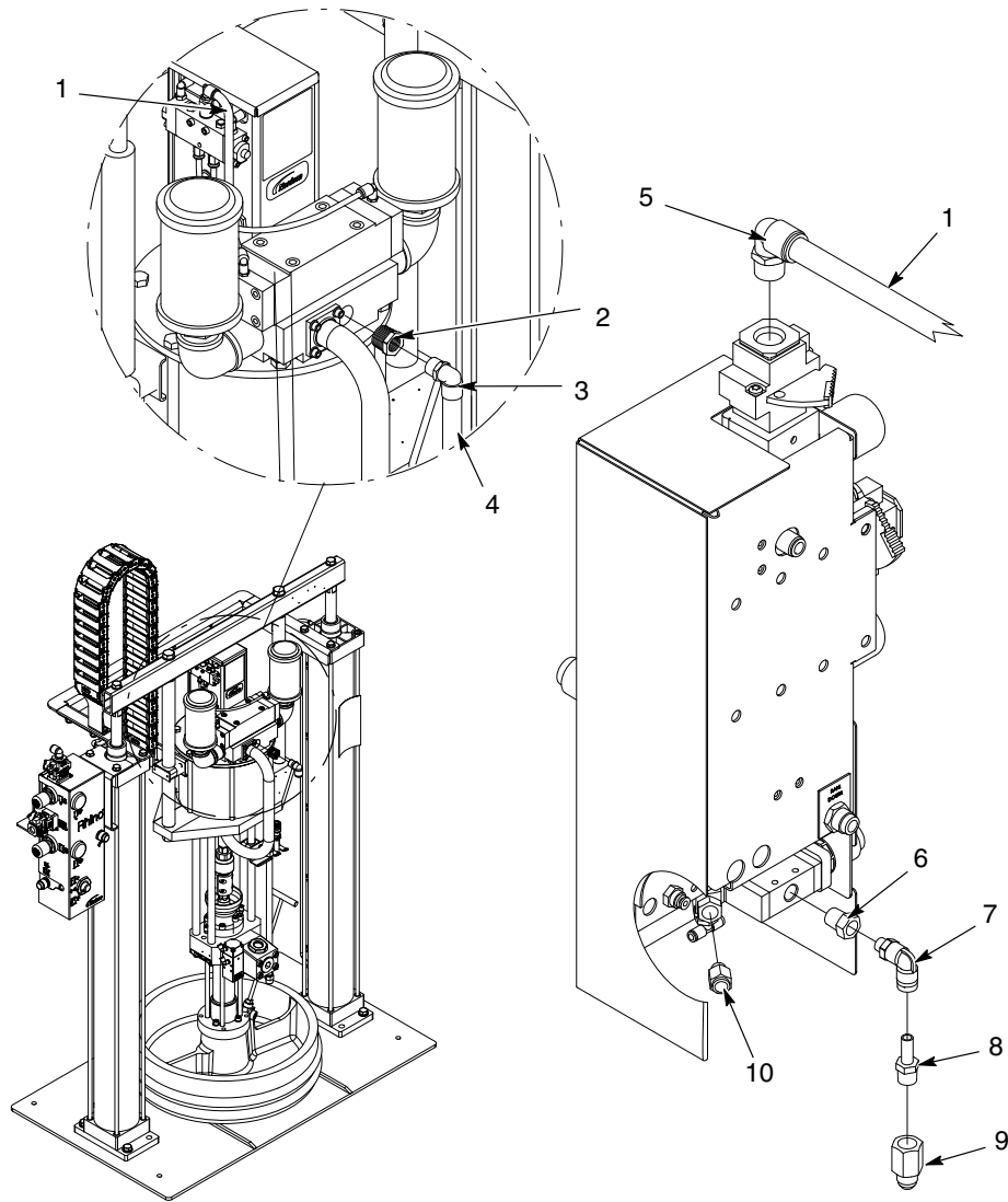
Obr. 25 Modul hadice s malým/veľkým rámom so vzduchovým motorom SD2, 5-gal. A 55-gal., pneumatický (2 z 2)
