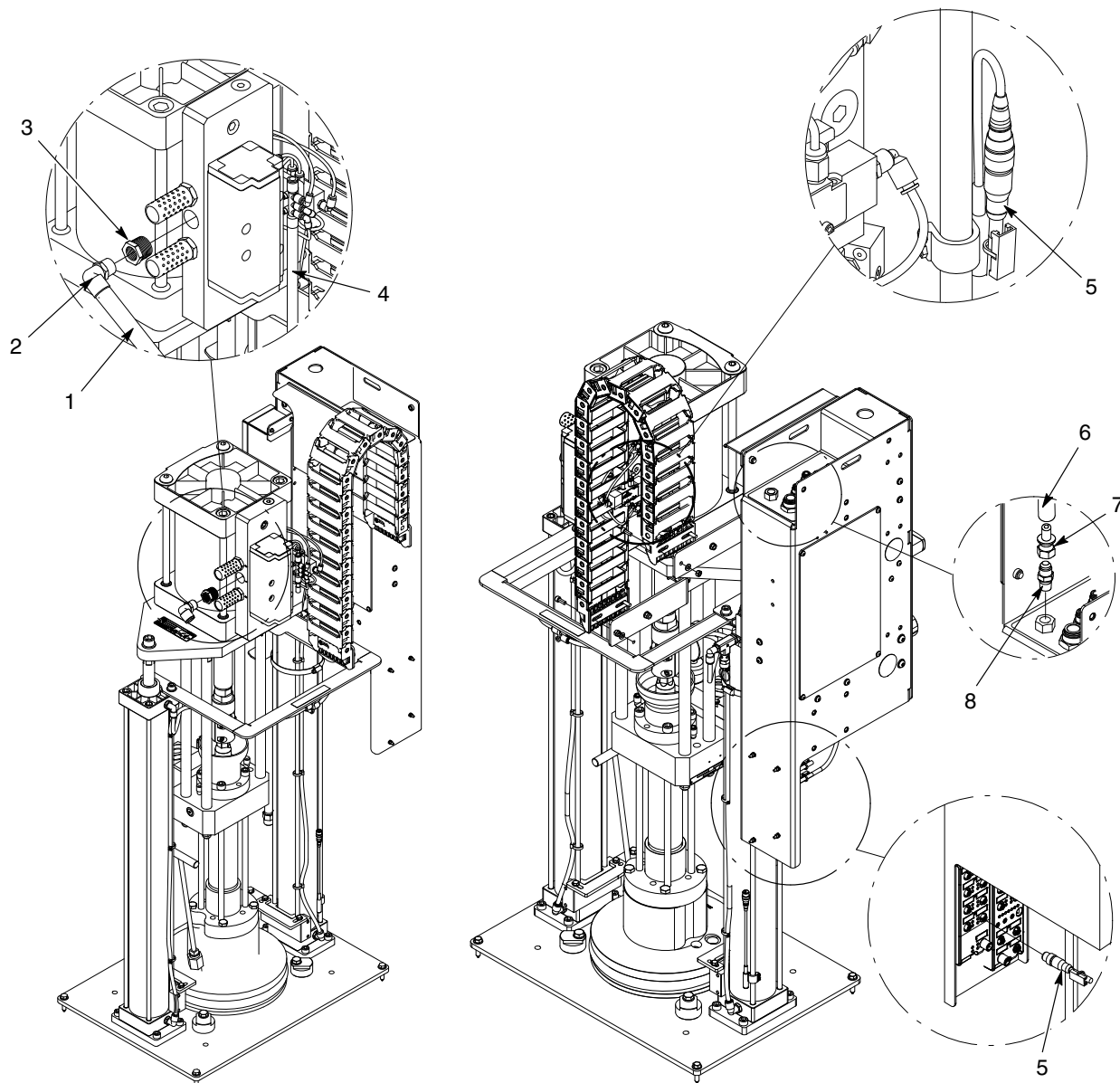
Obr. 4 Modul hadice s rámom DP so vzduchovým motorom SD3, 24 V DC (1 z 2)
