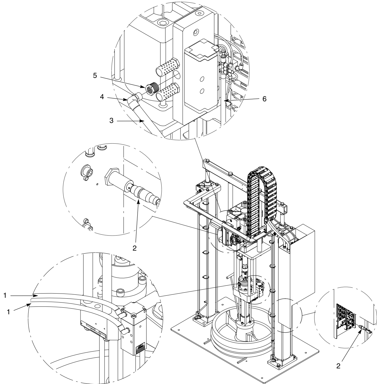
Obr. 17 Modul hadice s malým/veľkým rámom so vzduchovým motorom SD2, MT, 24 V DC (2 z 2)
