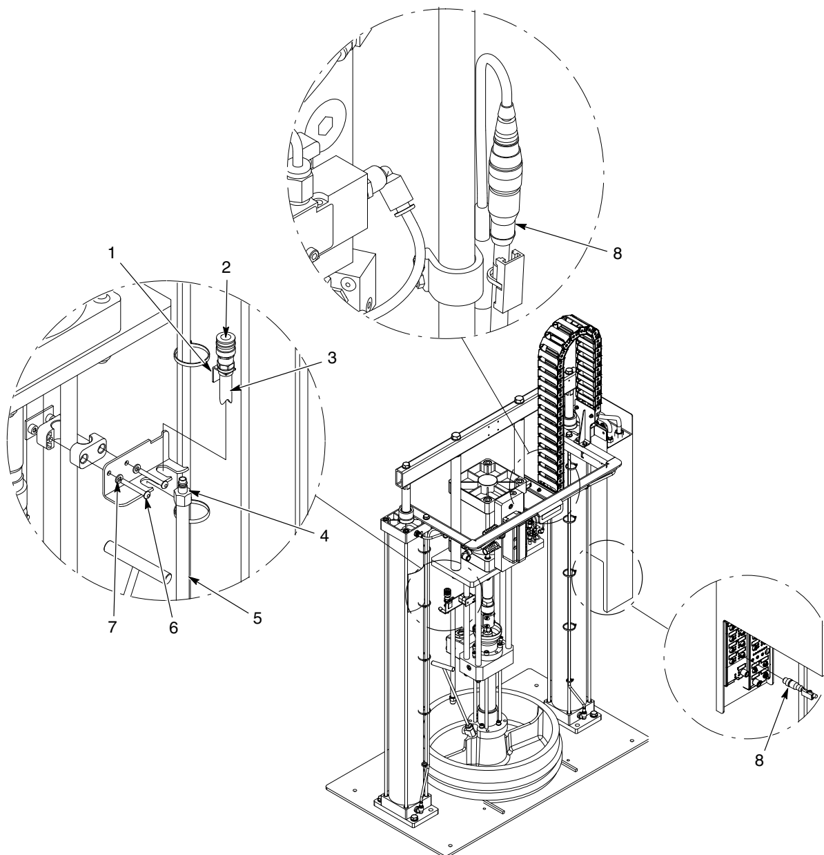
Obr. 10 Modul hadice s malým/veľkým rámom so vzduchovým motorom SD3, 24 V DC (3 z 3)
