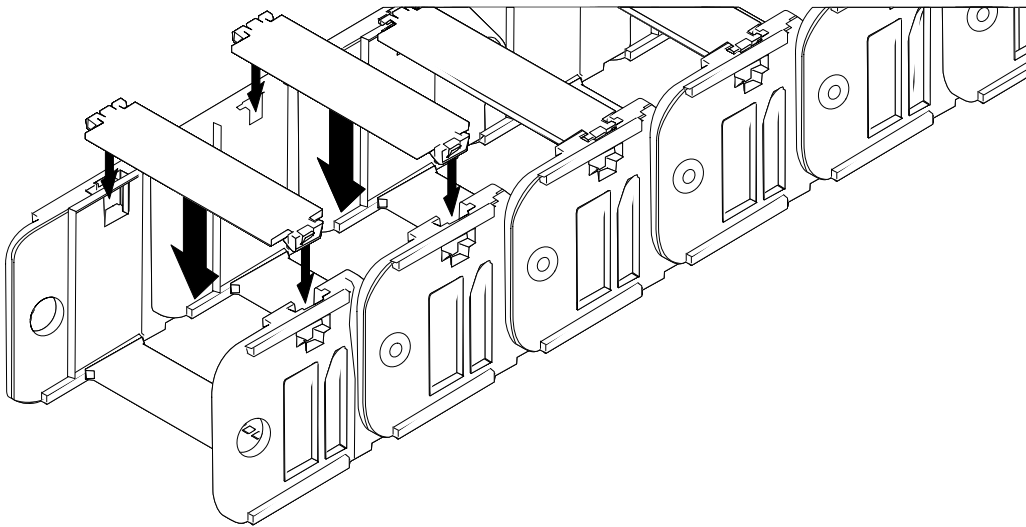
Obr. 3 Refazová trasa
