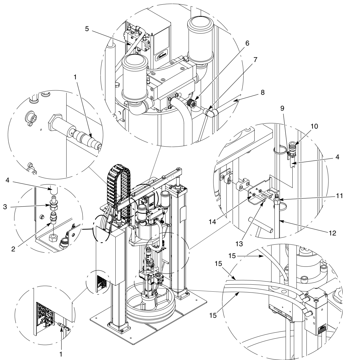
Obr. 13 Modul hadice s malým/veľkým rámom so vzduchovým motorom SD2, 24 V DC (3 z 3)
