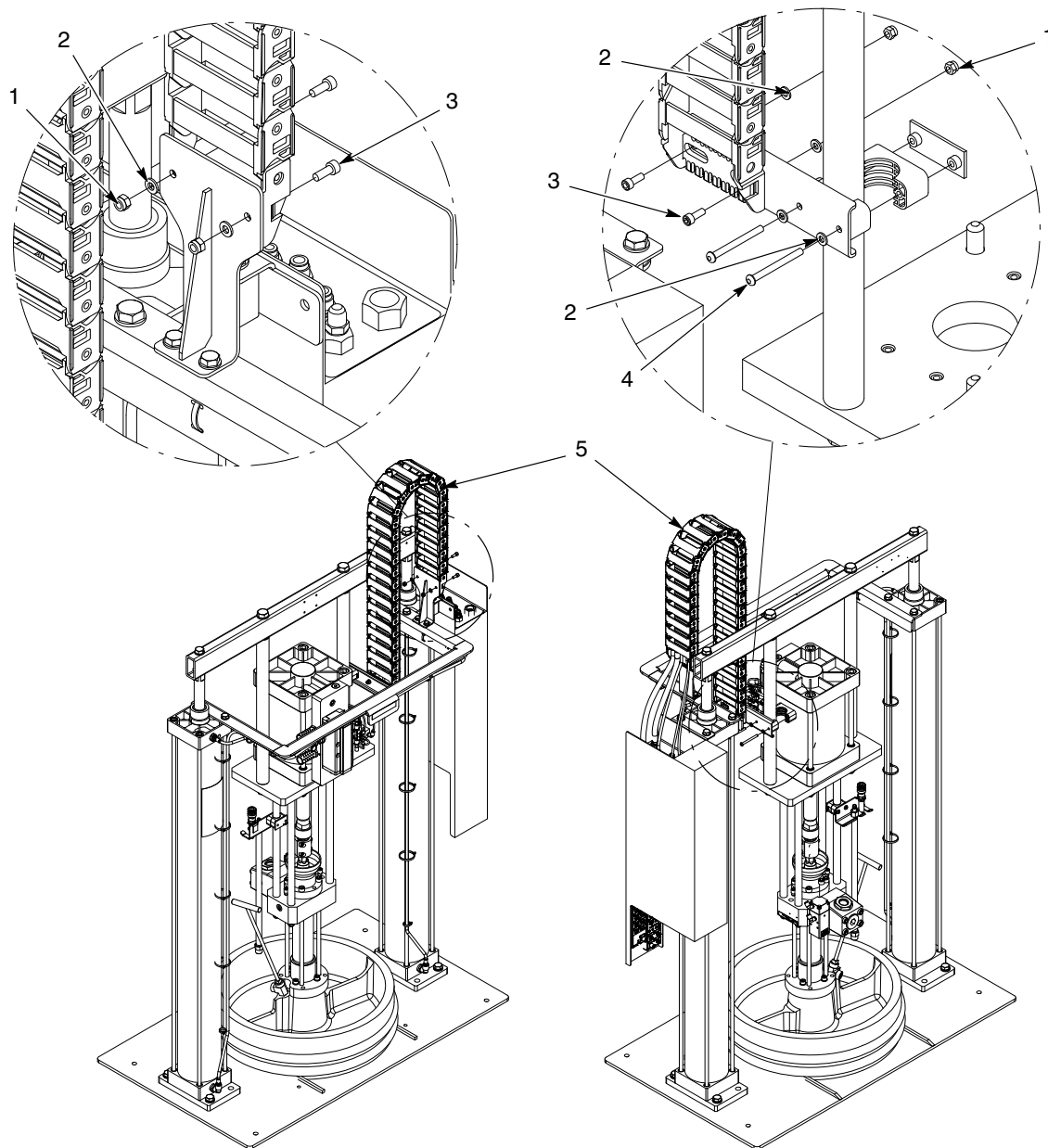
Obr. 14 Modul hadice s malým/velkým rámom so vzduchovým motorom SD3, MT, 24 V DC (1 z 2)
