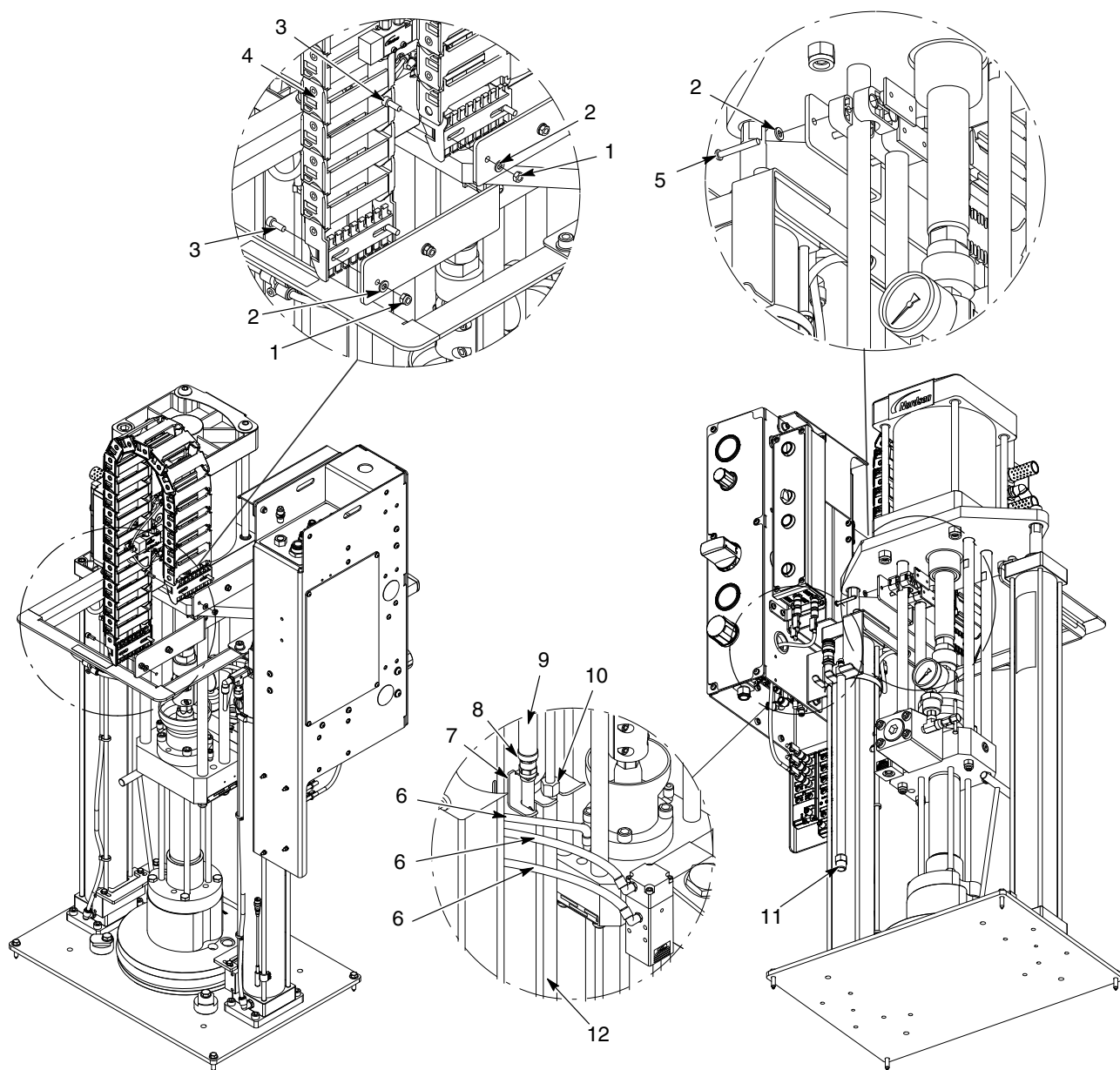
Obr. 5 Modul hadice s rámom DP so vzduchovým motorom SD3, 24 V DC (2 z 2)
