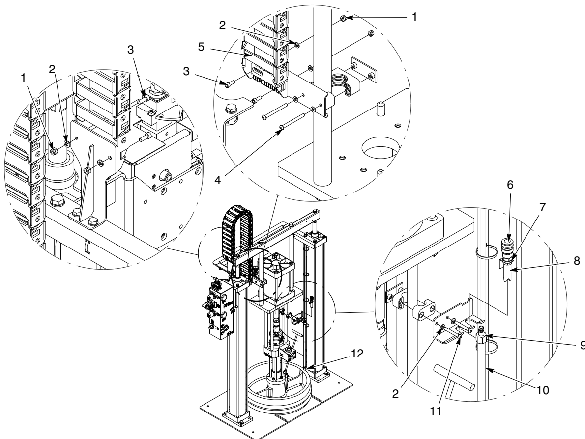
Obr. 22 Modul hadice s malým/velkým rámom so vzduchovým motorom SD3, 55-gal., pneumatický (1 z 2)
