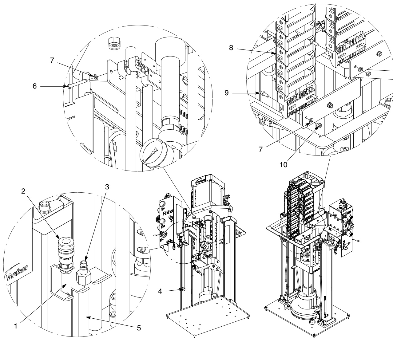
Obr. 18 Modul hadice s rámom DP so vzduchovým motorom SD3, pneumatický (1 z 2)
