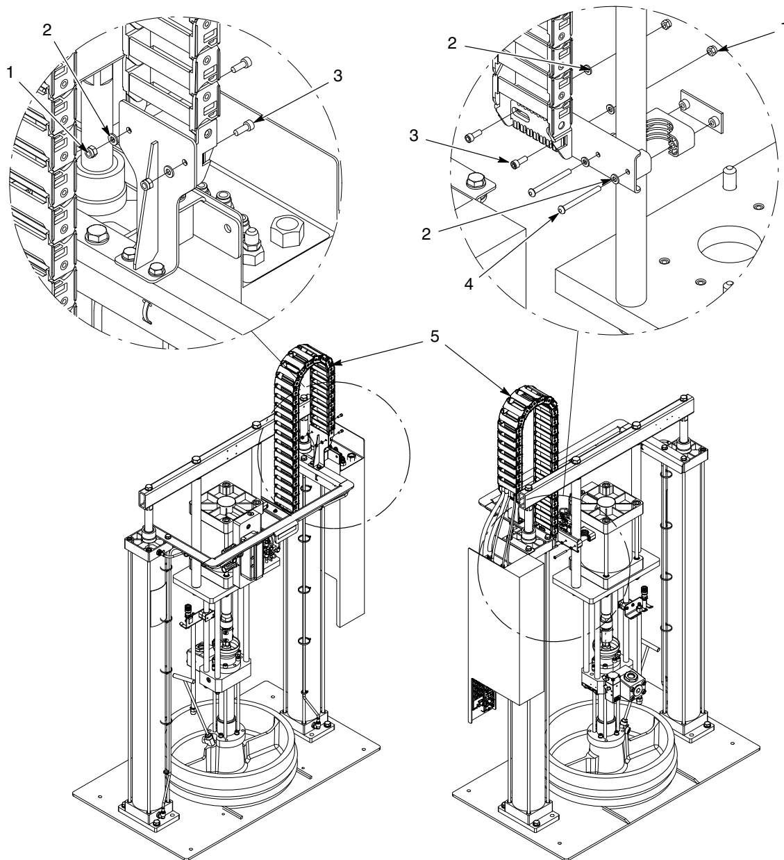
Obr. 8 Modul hadice s malým/velkým rámom so vzduchovým motorom SD3, 24 V DC (1 z 3)
