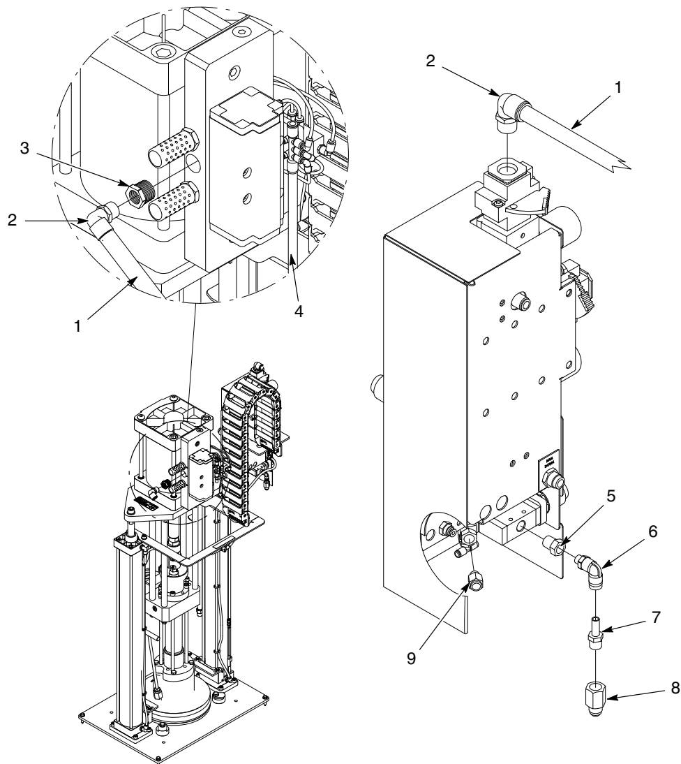
Obr. 19 Modul hadice s rámom DP so vzduchovým motorom SD3, pneumatický (2 z 2)
