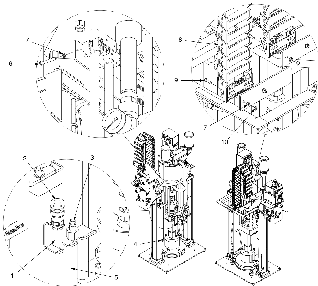
Obr. 20 Modul hadice s rámom DP so vzduchovým motorom SD2, pneumatický (1 z 2)
