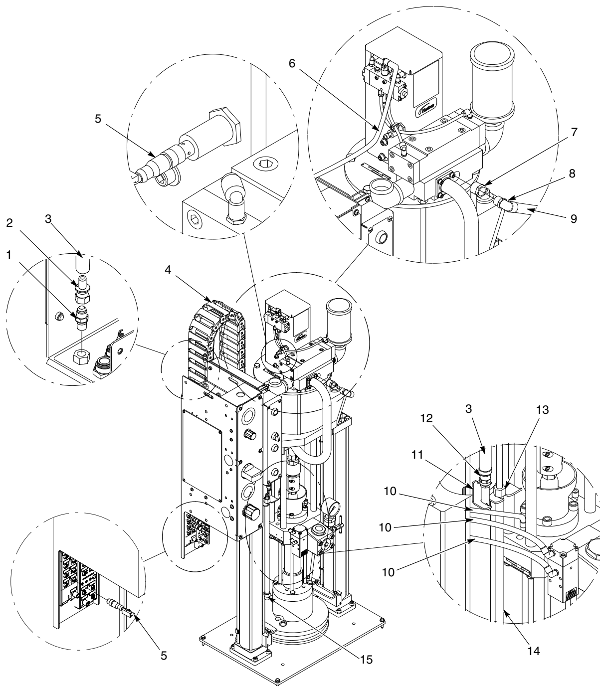
Obr. 6 Modul hadice s rámom DP so vzduchovým motorom SD2, 24 V DC (1 z 2)
