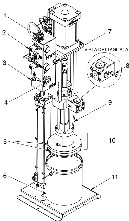
Figura 1 Scaricatore a montante singolo Rhino
