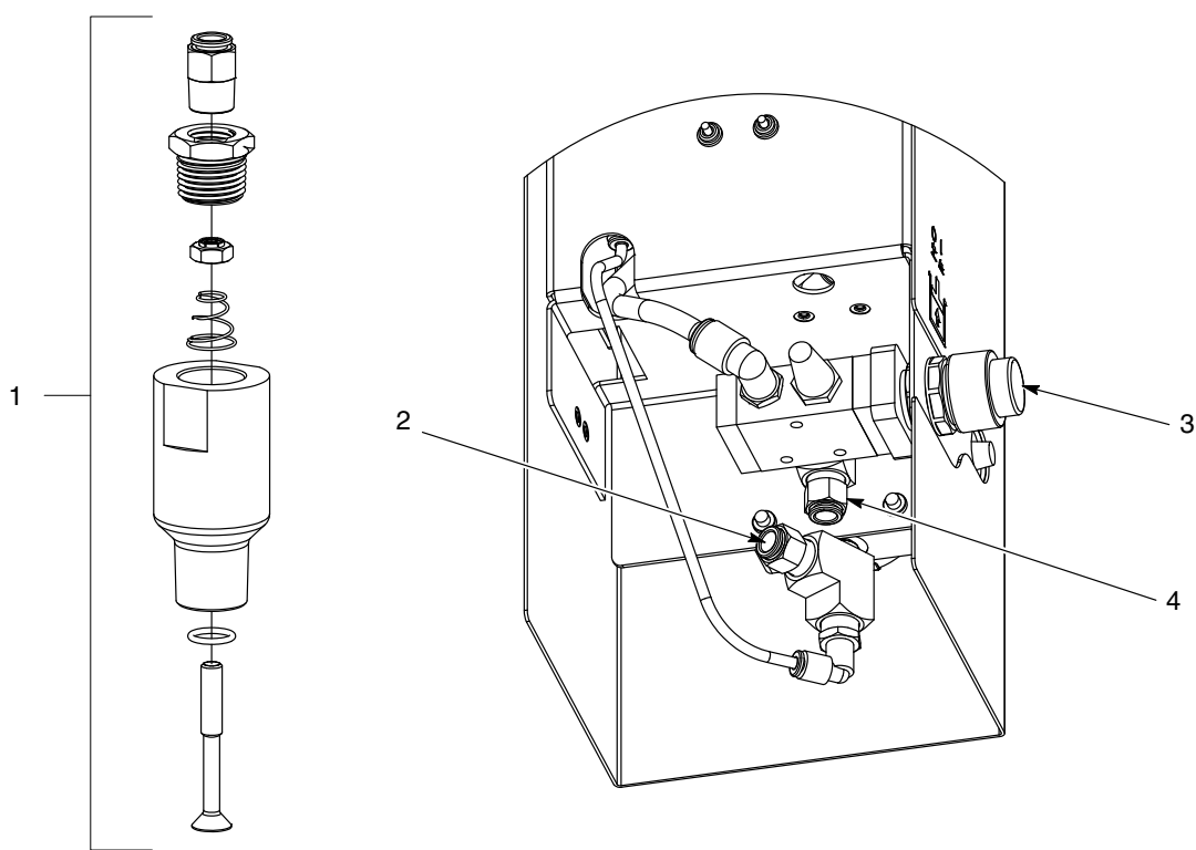
Obrázek 2 Montáž a armatury pojistného ventilu
