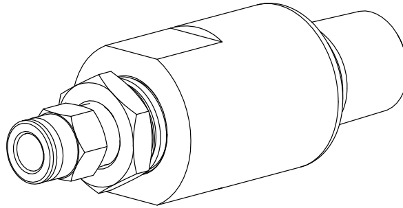
Obrázek 3 Sestava pojistného ventilu ofukovače kontejneru na materiál
