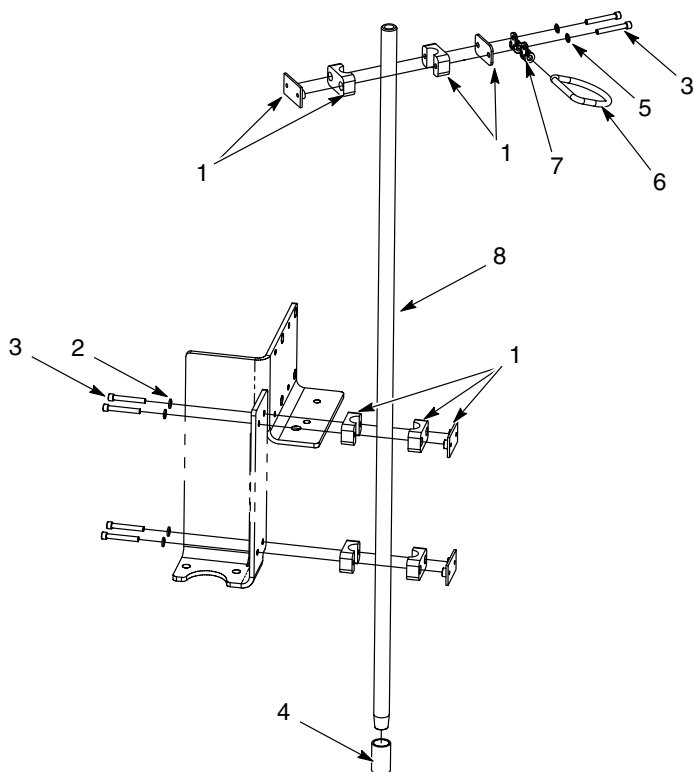
Obrázek 2 Modul držáku hadic pro 5galonový přečerpávač
