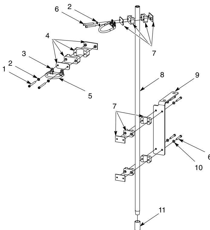
Obrázek 3 Modul držáku hadic pro 55galonový přečerpávač
