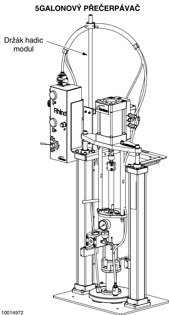
Obrázek 1 Modul držáku hadic
