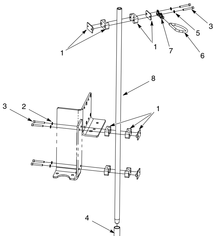
図 2 5ガロン アンローダー用のホースサポート モジュール
