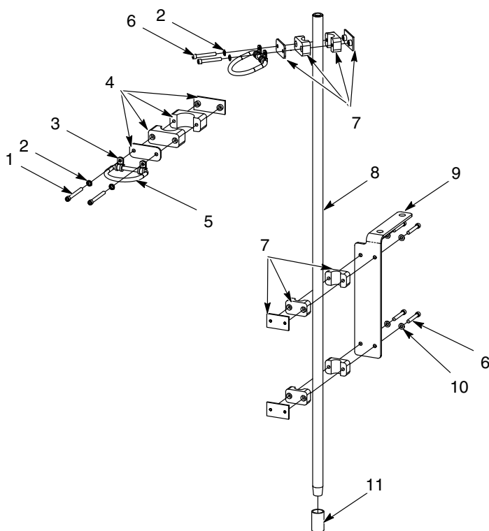
図 3 55ガロン アンローダー用のホースサポート モジュール
