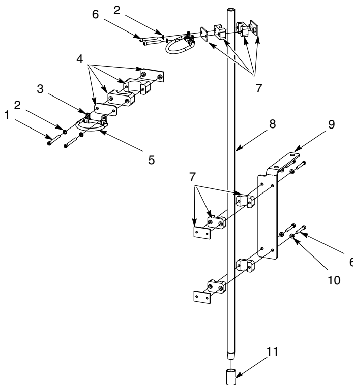
Figure 3 Module porte-tuyau pour vide-fûts de 55 Gal (200 l)
