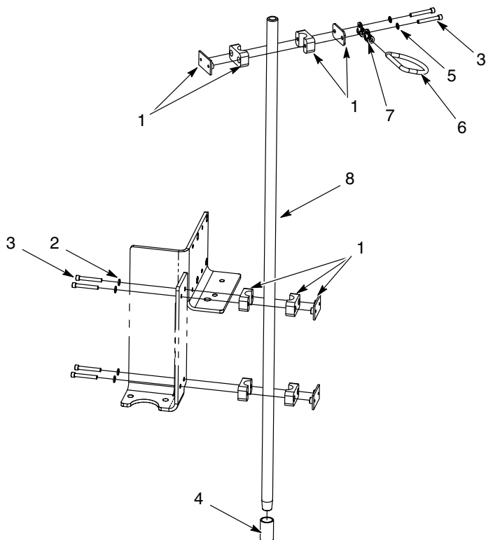
Figure 2 Module porte-tuyau pour vide-fûts de 5 Gal (20 l)
