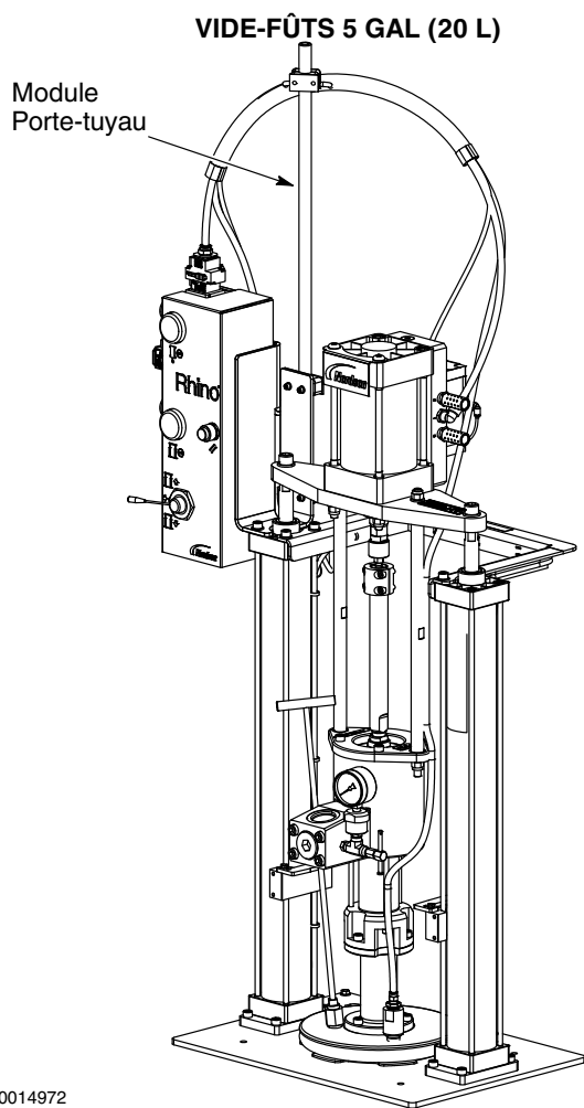
Figure 1 Module porte-tuyau
