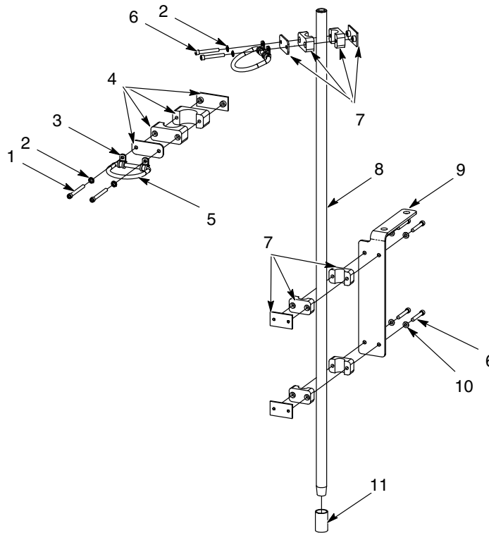
Figura 3 Módulo de soporte de manguera para descargador de 55 galones
