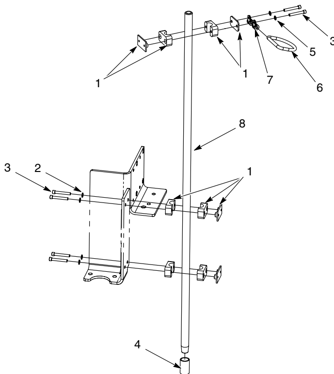
Figura 2 Módulo de soporte de manguera para descargador de 5 galones
