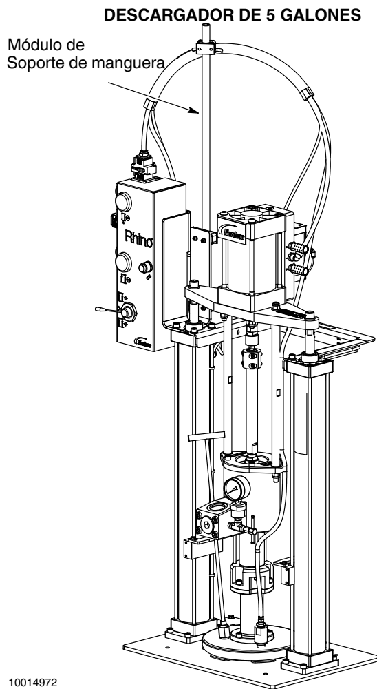
Figura 1 Módulo de soporte de manguera
