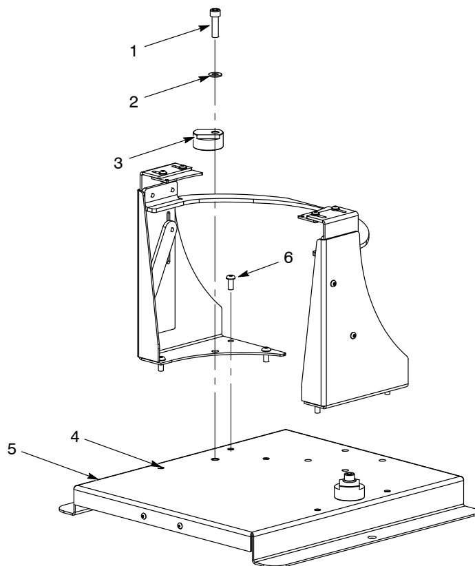
図 2 容器ホールドダウンの取付け
