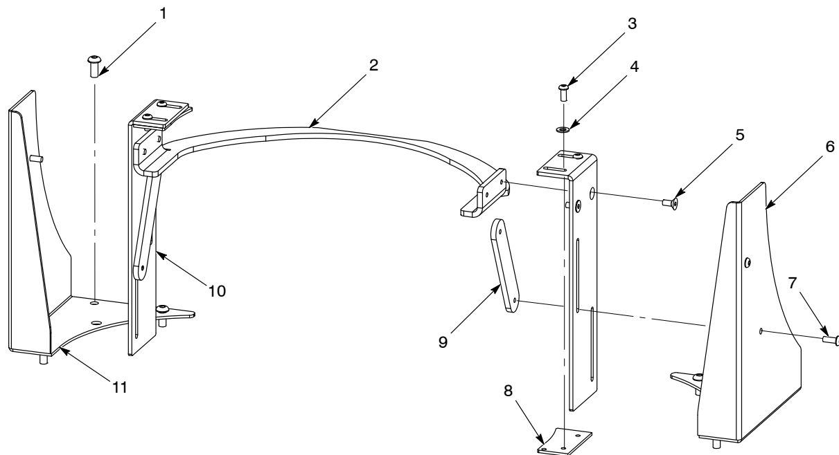
図 4 容器ホールドダウン
