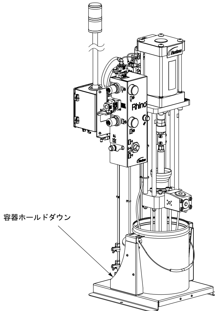
図 1 容器ホールドダウン
