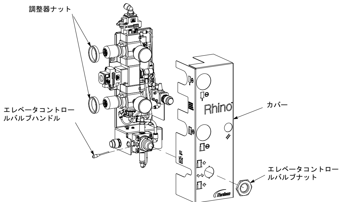
図 1 エア圧コントロールモジュール カバーの取外し
