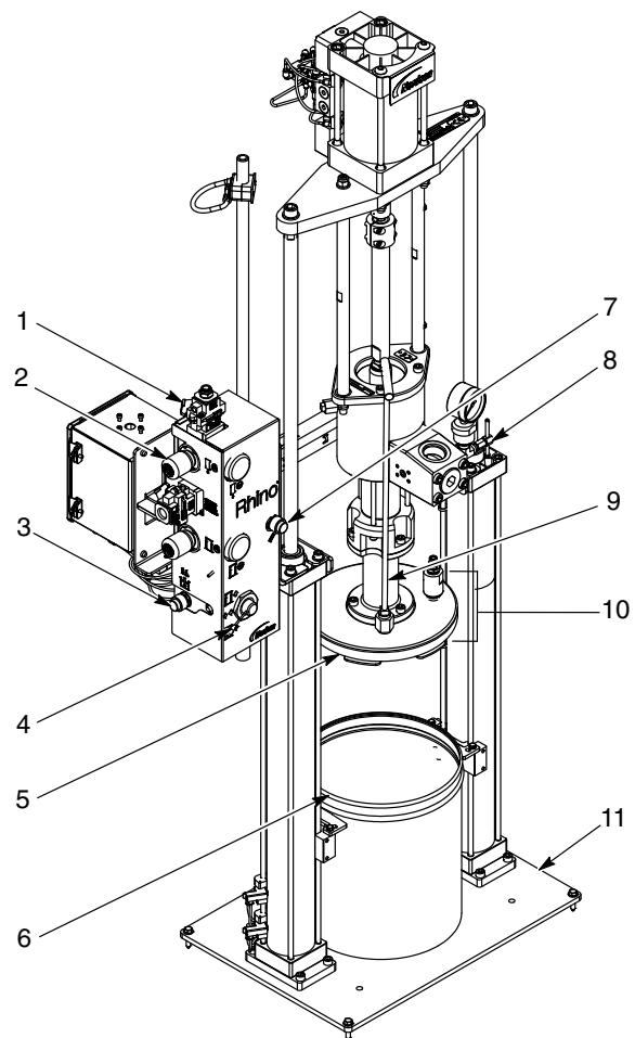
Abbildung 1 Rhino AB 5-Gallonen-Entleerer
