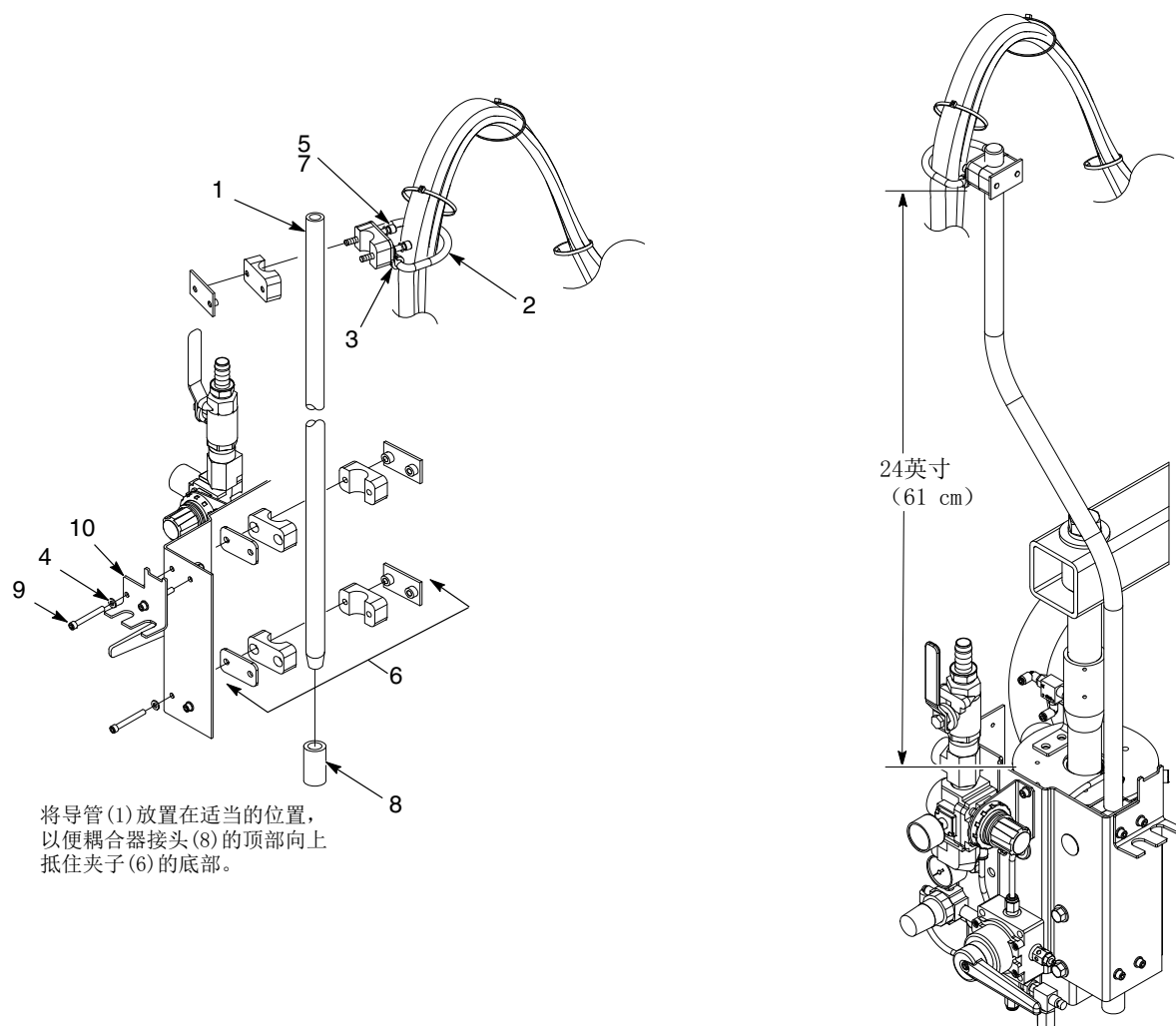
图 2 典型Rhino VE胶管支撑安装
