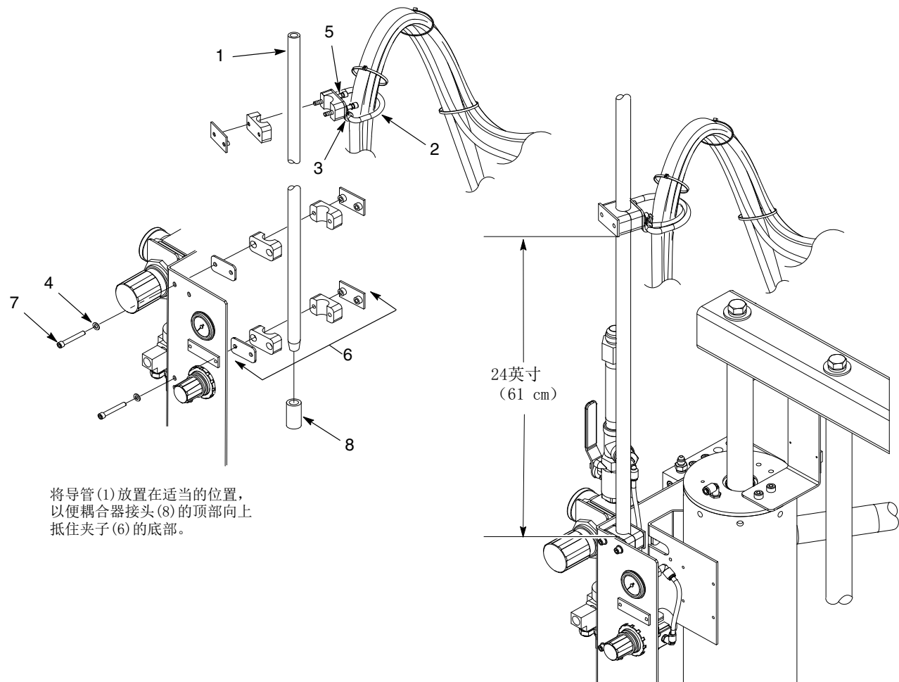
图 1 典型Rhino SD2/XD2安装
