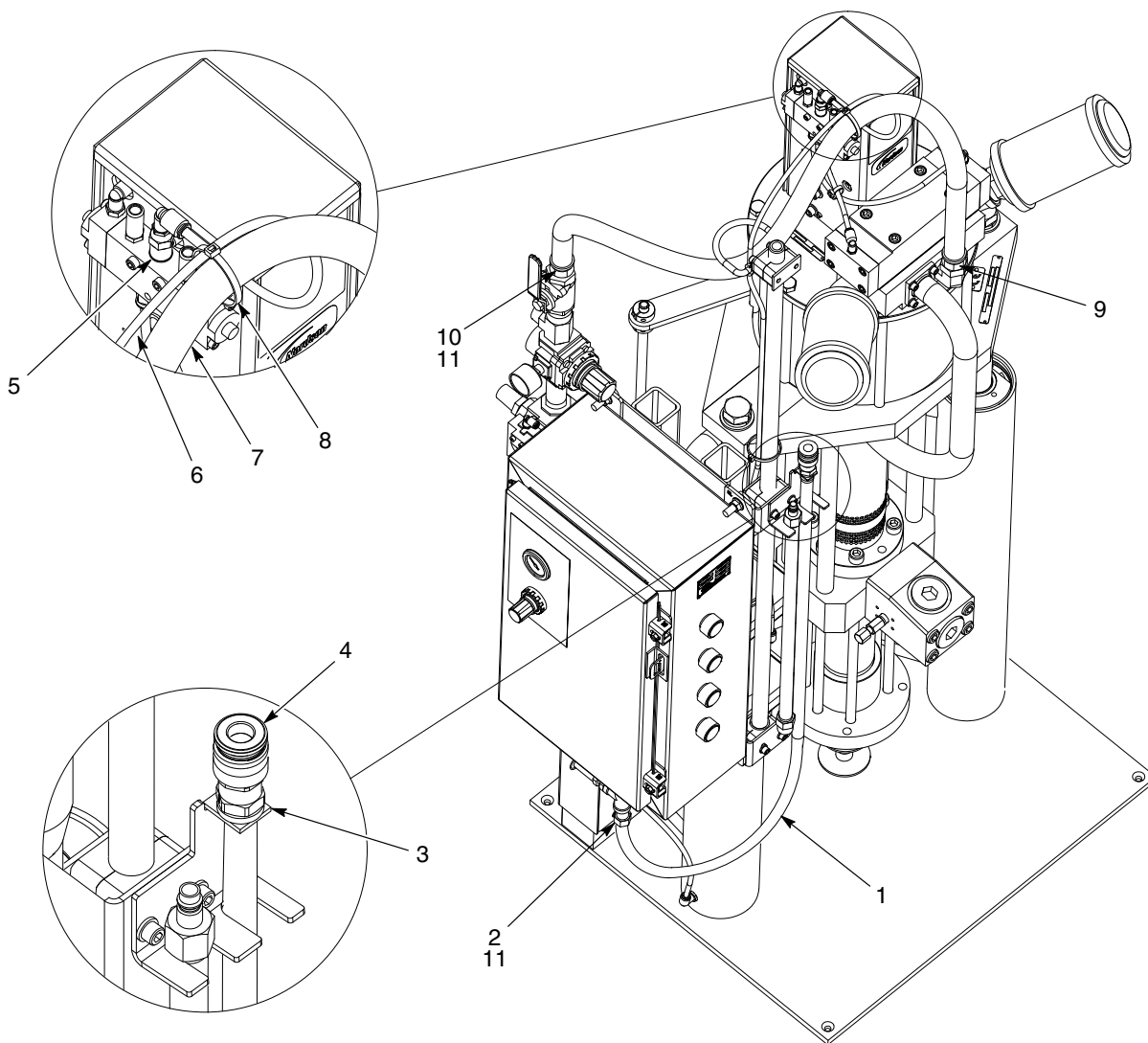
图 18 Rhino VE小型泵座CE胶管
