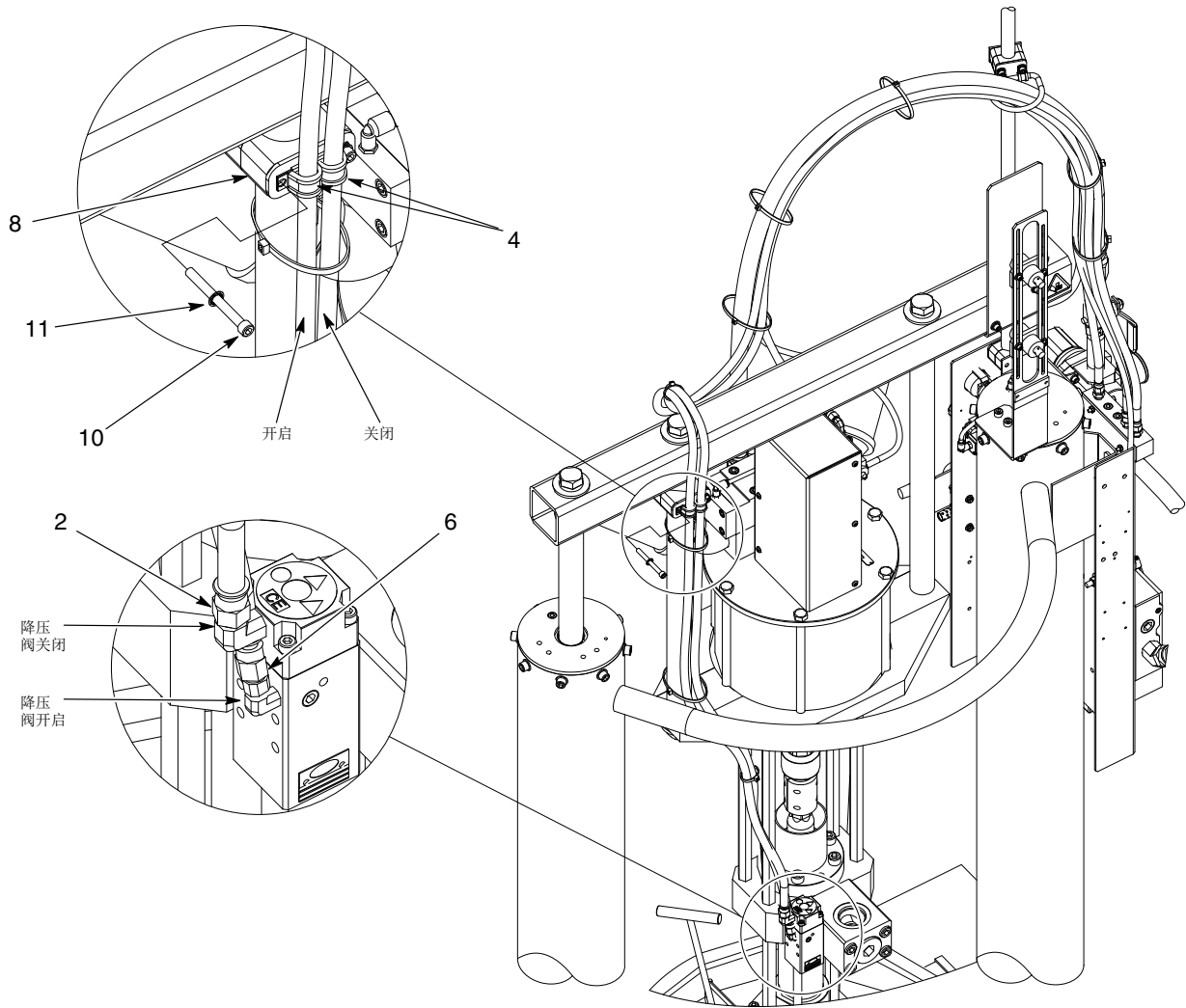
图 7 配有降压选项的5/30加仑大型泵座耐火胶管 (续)
