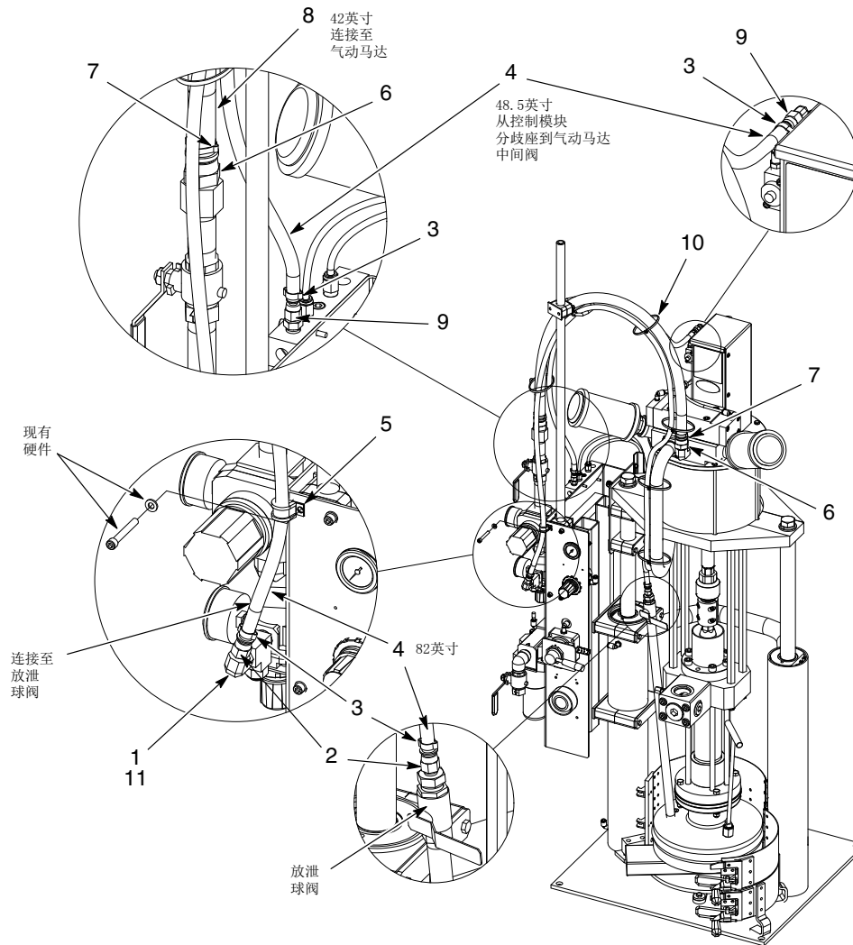
图 3 小型泵座黑色胶管
