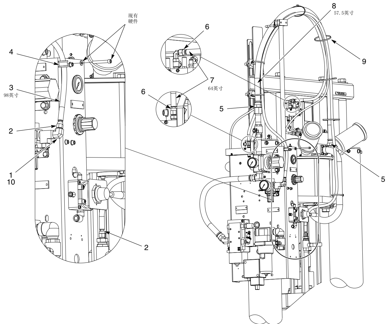
图 10 55加仑大型泵座耐火胶管
