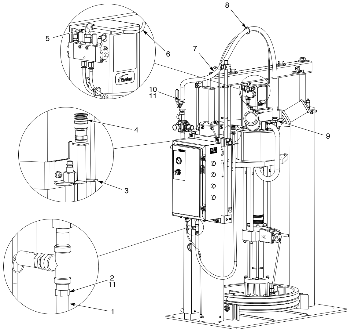
图 20 Rhino VE大型泵座CE胶管
