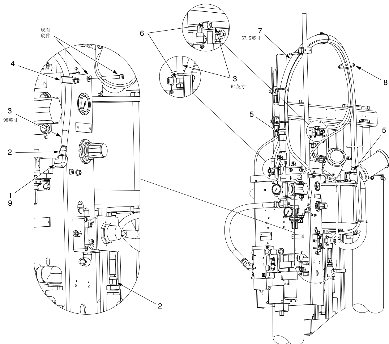
图 4 5/30加仑大型泵座耐火胶管
