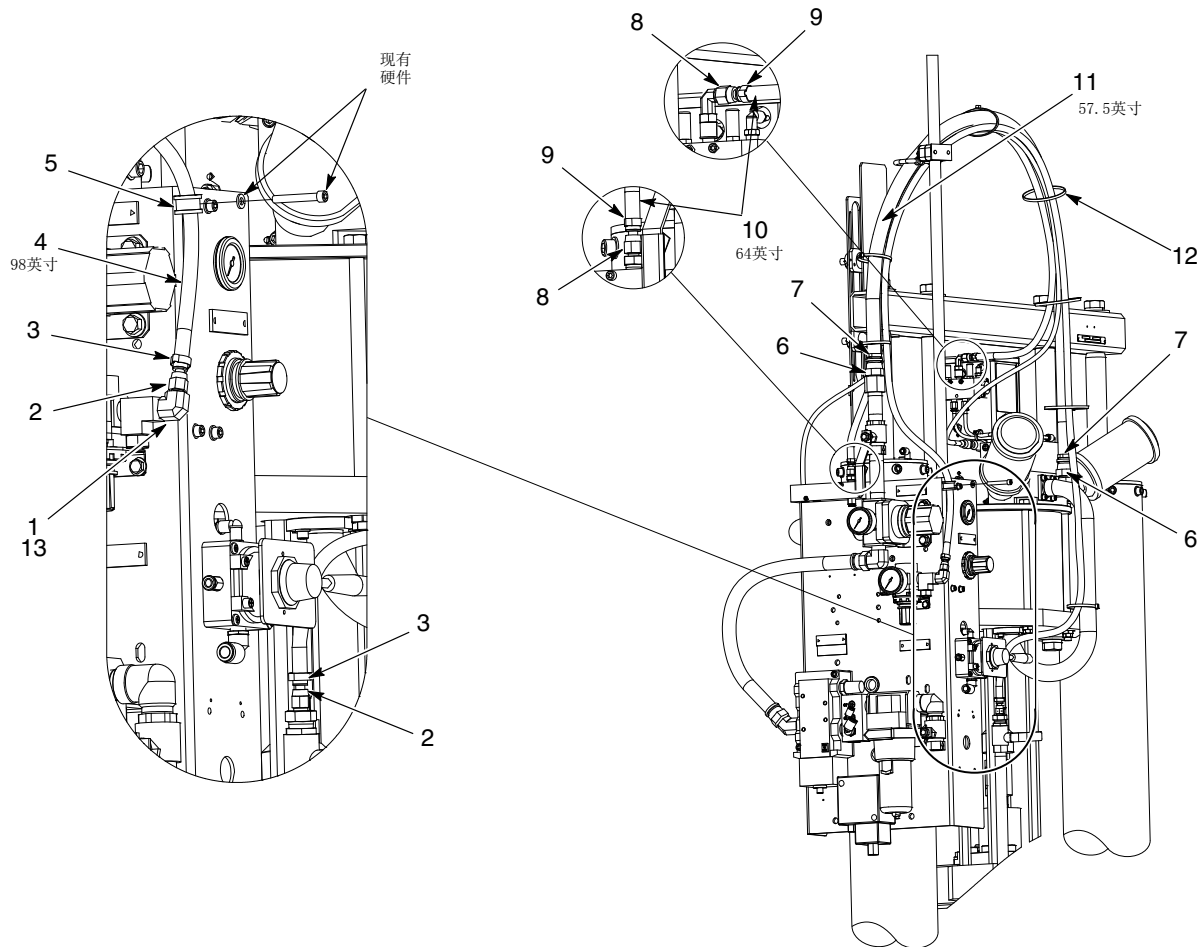
图 12 55加仑大型泵座黑色胶管
