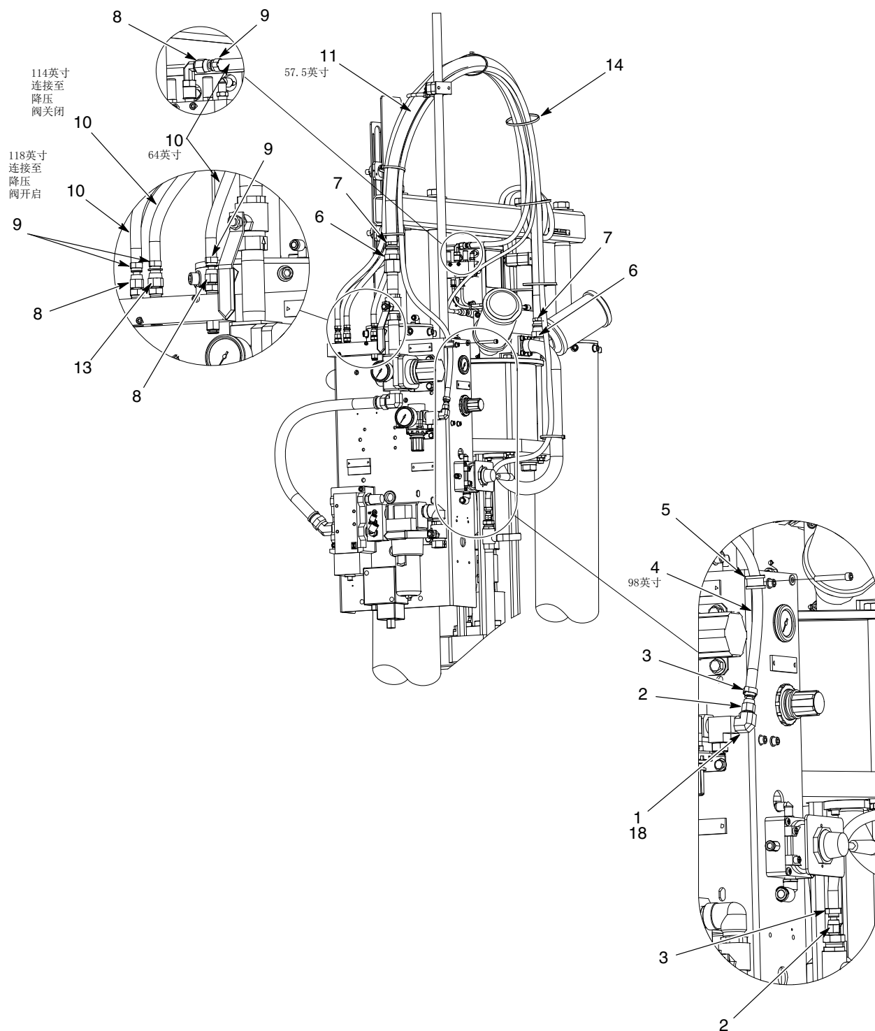
图 15 配有降压选项的55加仑大型泵座黑色胶管
