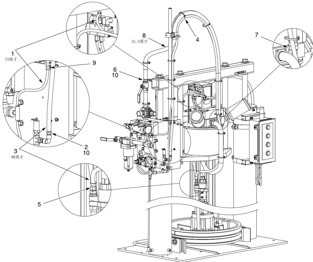
图 11 55加仑大型泵座绿色耐火胶管
