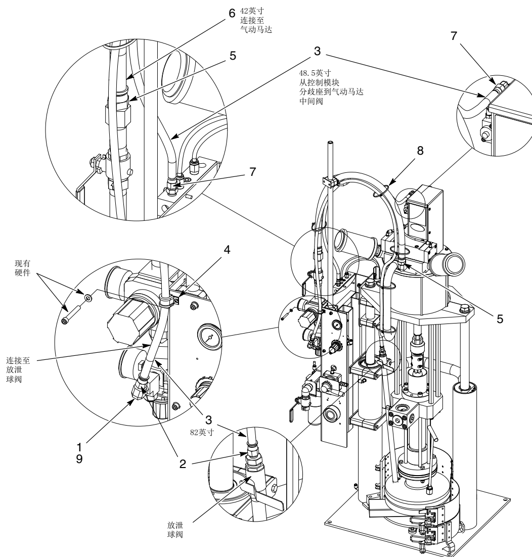
图 2 小型泵座耐火互连胶管模块
