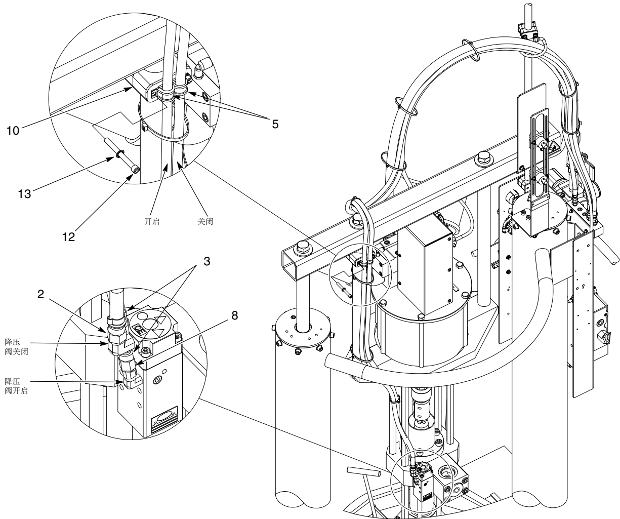
图 9 配有降压选项的5/30加仑大型泵座黑色胶管（续）
