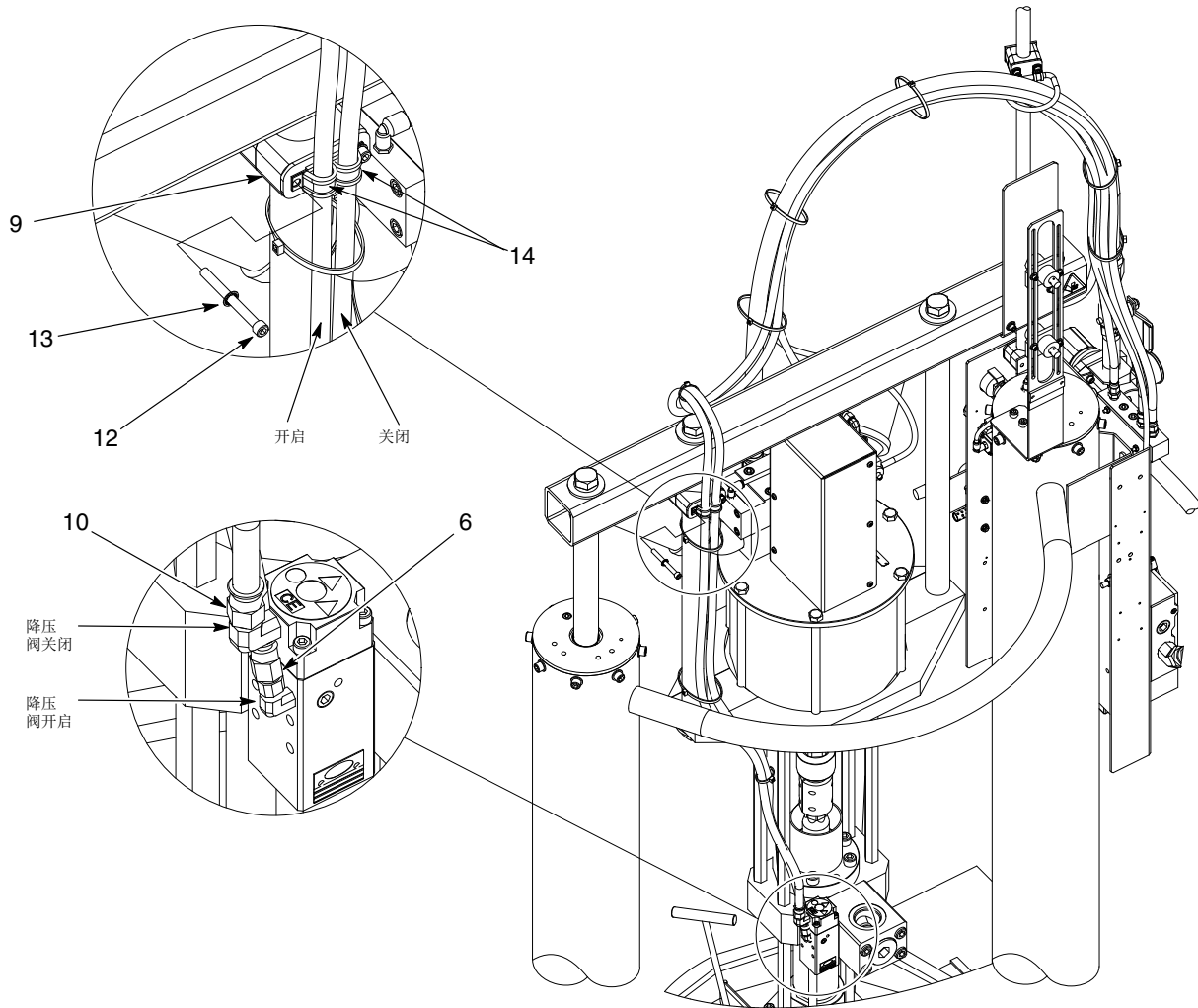
图 14 55加仑大型泵座黑色胶管 (续)
