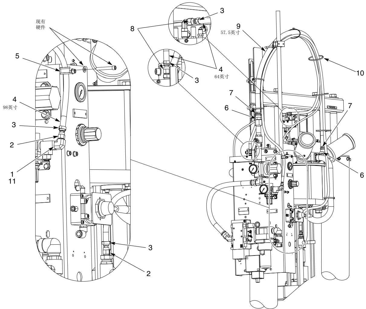
图 5 5/30加仑大型泵座黑色胶管
