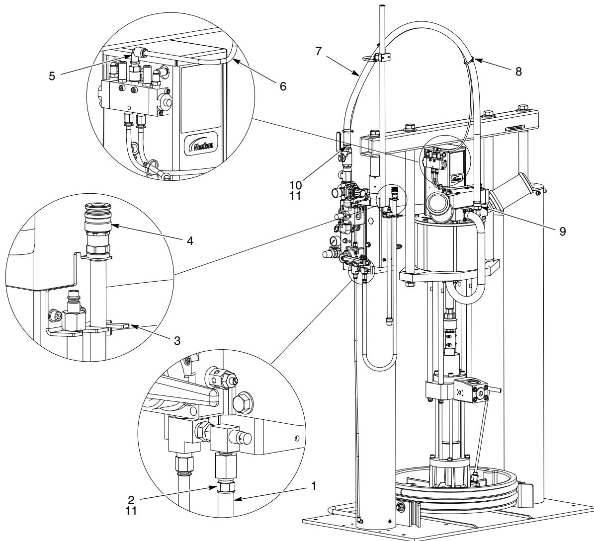
图 19 Rhino VE大型泵座CE胶管
