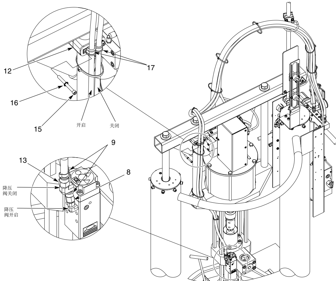
图 16 配有降压选项的55加仑大型泵座黑色胶管 (续)
