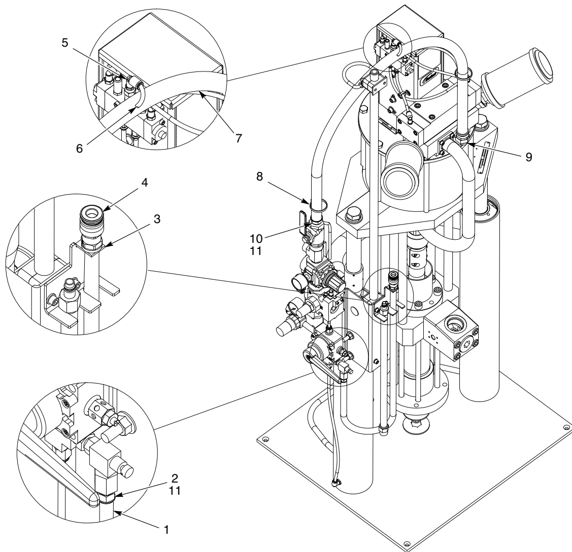
图 17 Rhino VE小型泵座胶管
