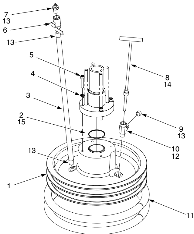
图 5 30加仑从动模块（适用于5.8和8.1立方英寸泵）
