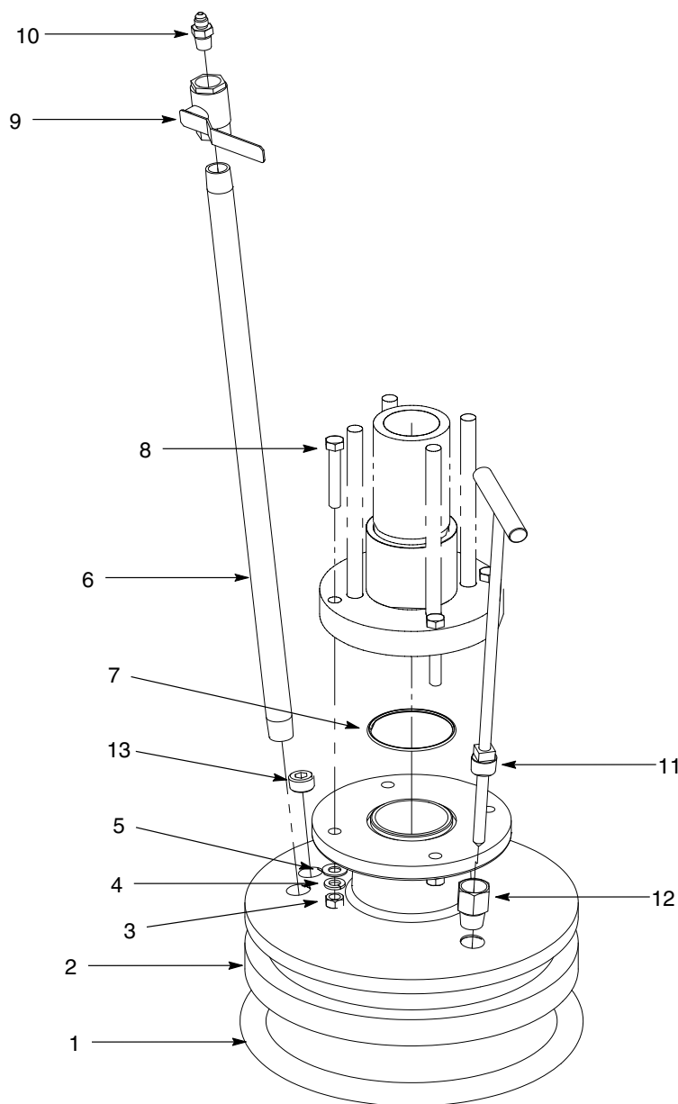
图 3 5加仑从动模块（适用于5.8立方英寸泵）
