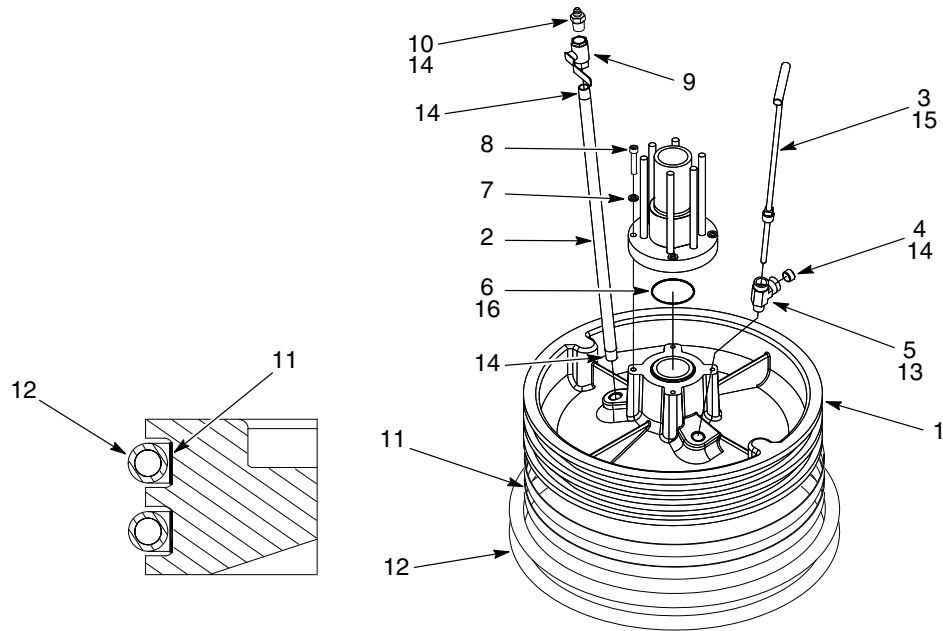
图 6 55加仑从动模块（适用于5.8立方英寸泵）
