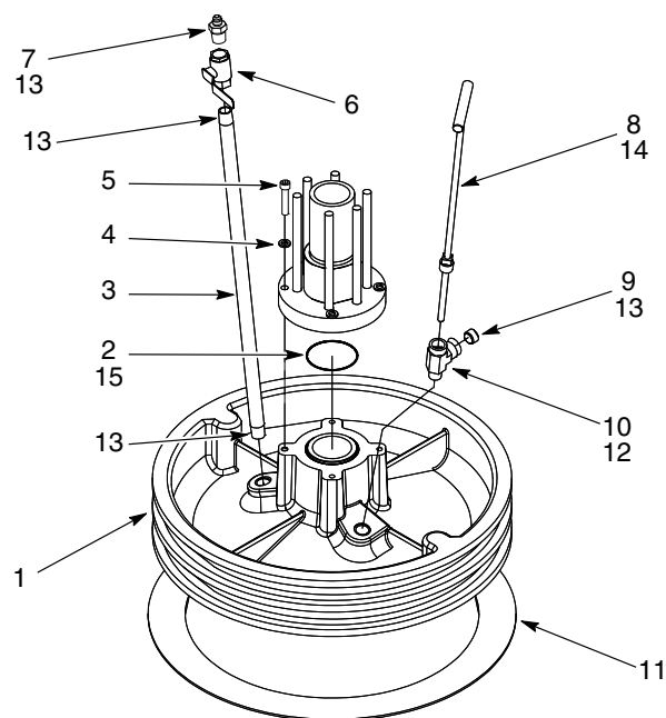
图 9 带有钢环的55加仑从动模块 (适用于5.8和8.1立方英寸泵)
