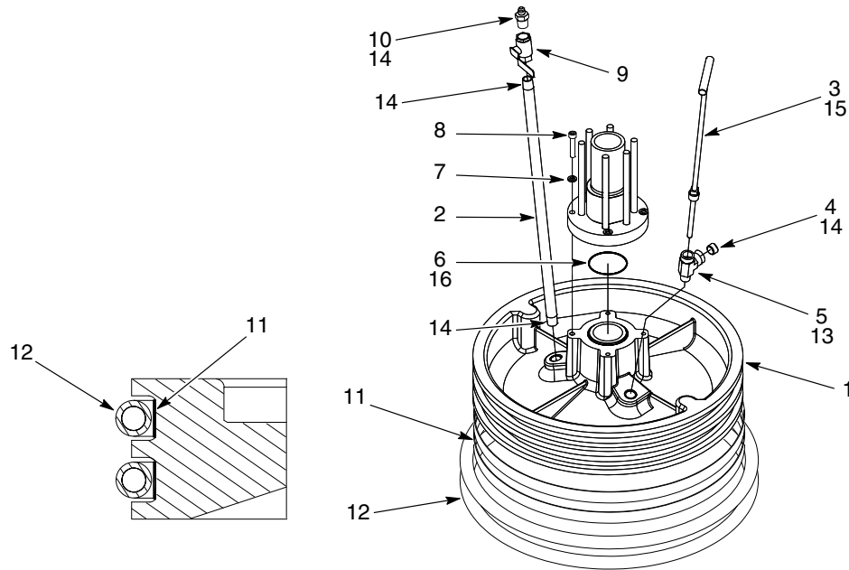
图 8 55加仑从动模块（适用于8.1立方英寸泵）
