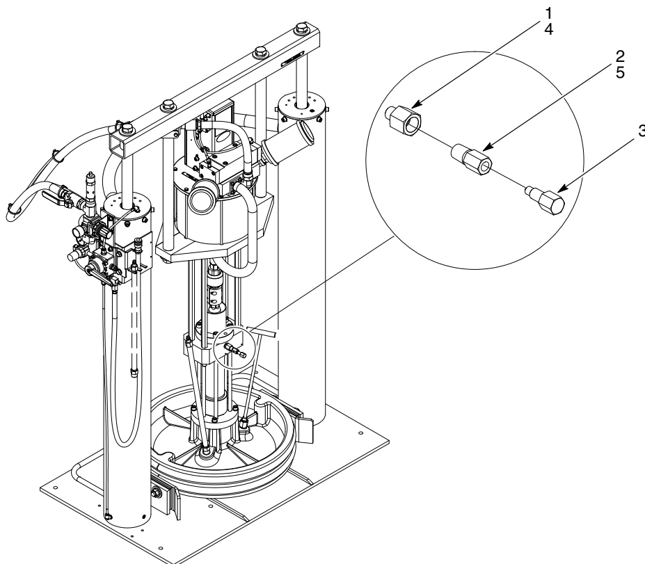
Рис. 1 Спускной клапан Rhino VE
