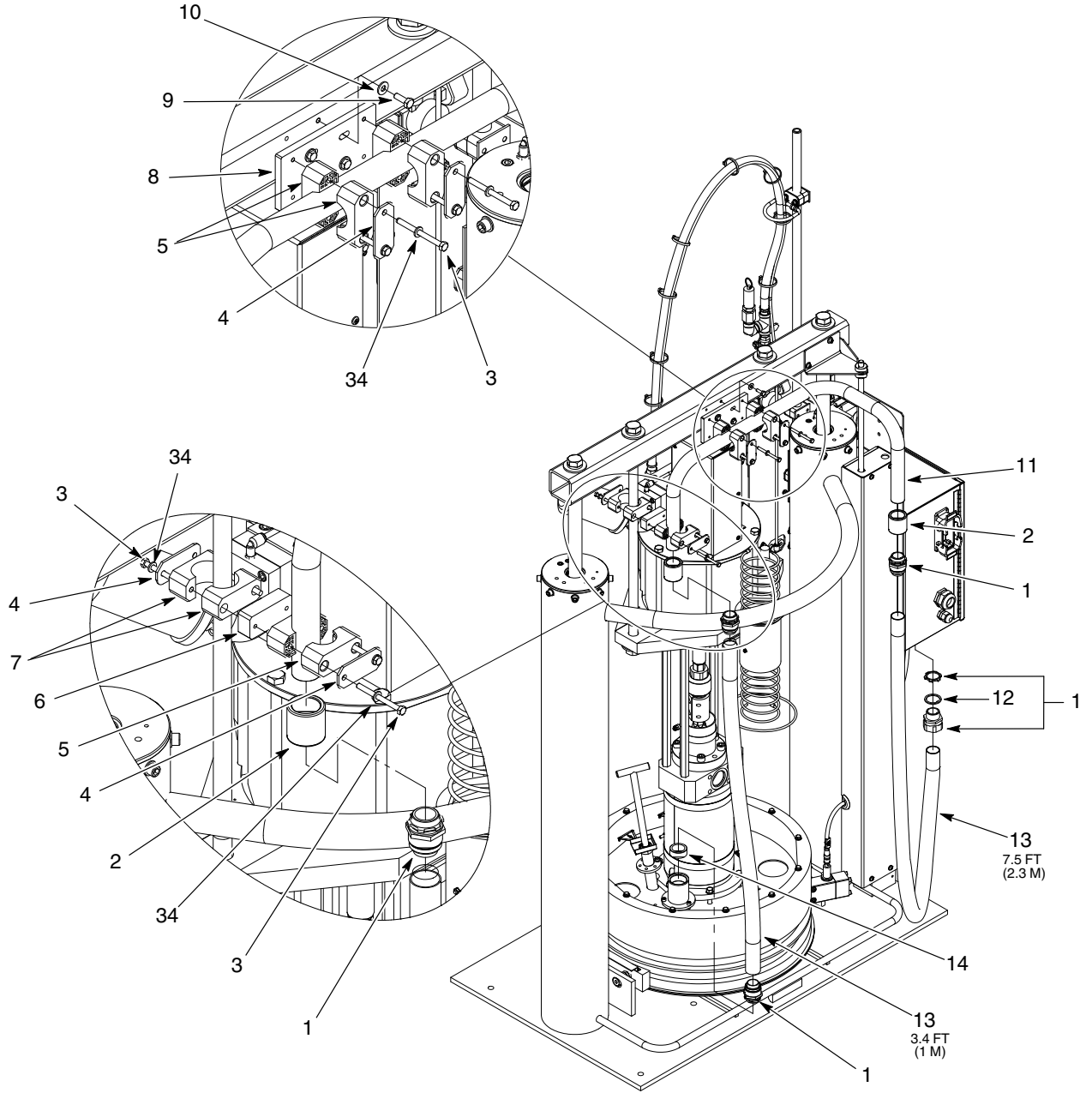
Şekil 2 Tesisat Ünitesi Parçaları
