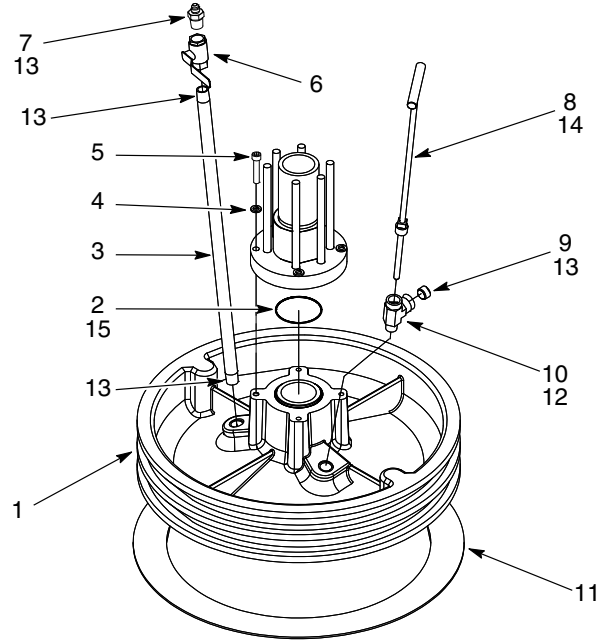
Şekil 9 5.8 ve 8.1 İnç küp Pompalar için Çelik Halkalı 55 - Galon Takipçi Modülleri
