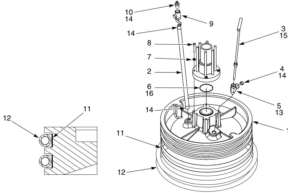
Şekil 6 5.8 İnç küp pompalar için 55-Galon Takipçi Modülleri
