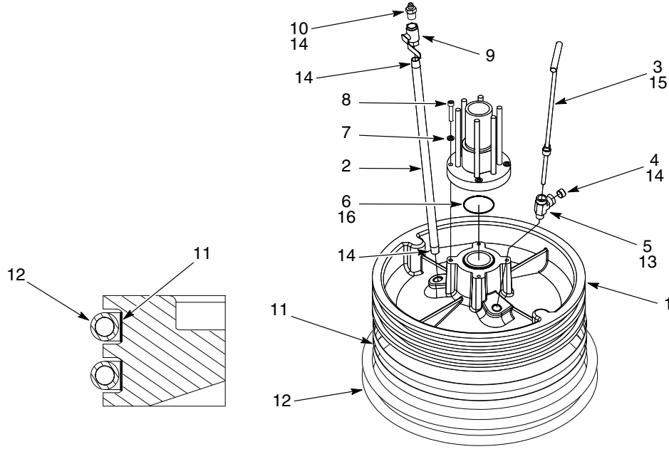
Şekil 8 8.1 İnç küp pompalar için 55-Galon Takipçi Modülleri
