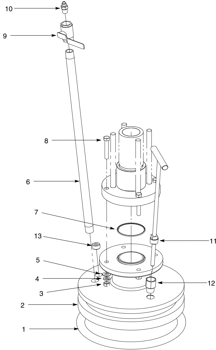
Şekil 3 5.8 İnç küp pompalar için 5-Galon Takipçi Modülleri
