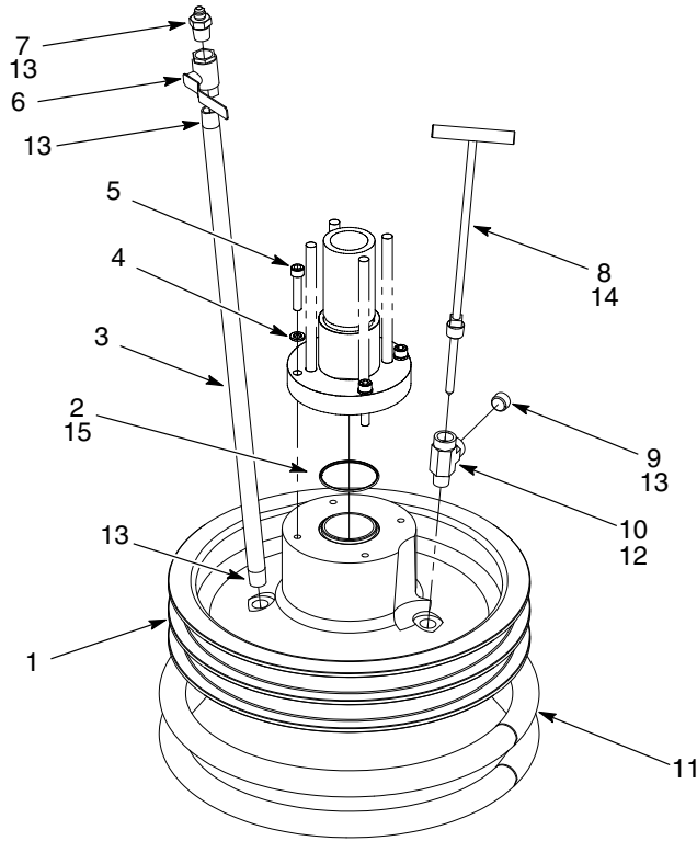
Şekil 5 5.8 ve 8.1 İnç küp pompalar için 30-Galon Takipçi Modülleri
