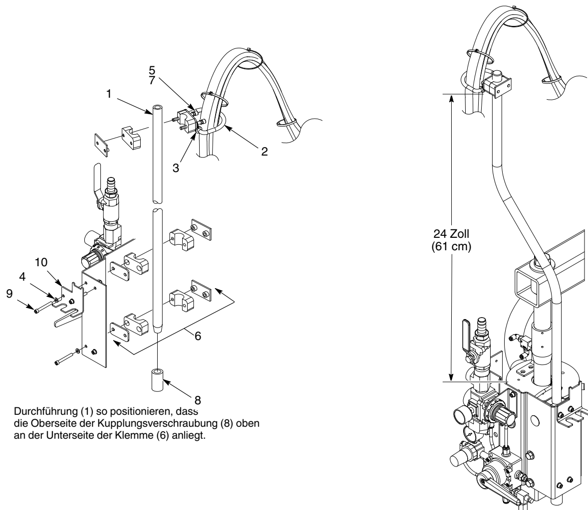
Abb. 2 Typische Rhino VE Installation Schlauchhaltemodul
