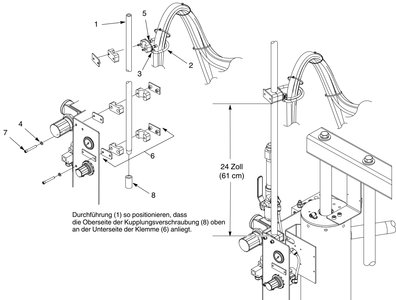
Abb. 1 Typische Rhino SD2/XD2 Installation
