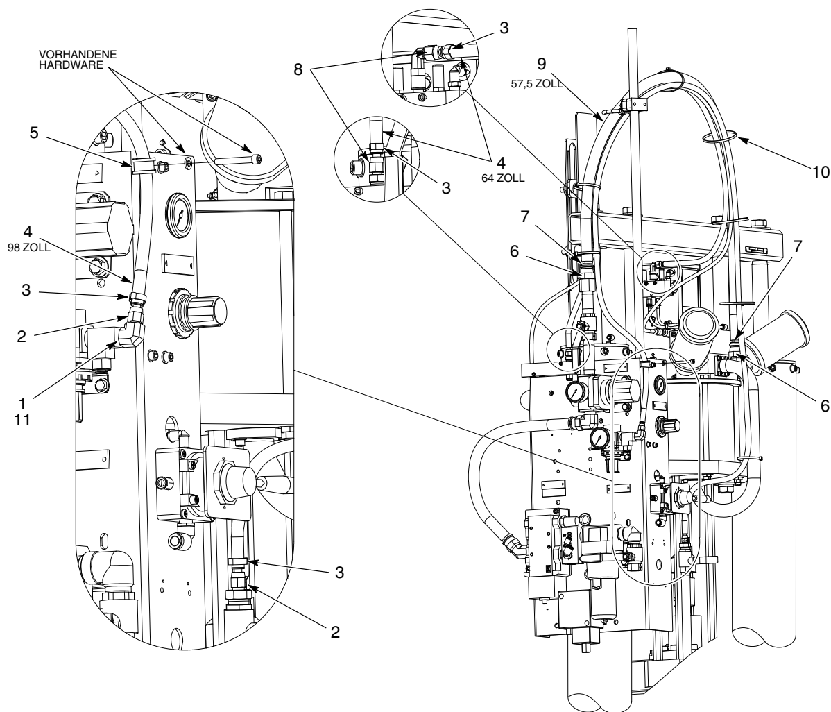
Abb. 5 Schwarzer Schlauch für großen Rahmen mit 5/30 Gallonen
