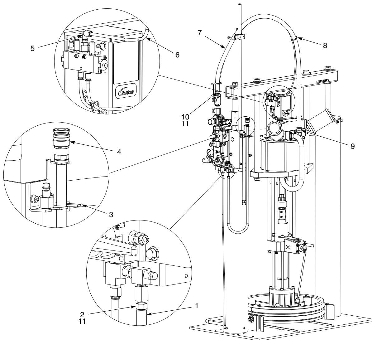
Abb. 19 CE-Schlauch für Rhino VE mit großem Rahmen
