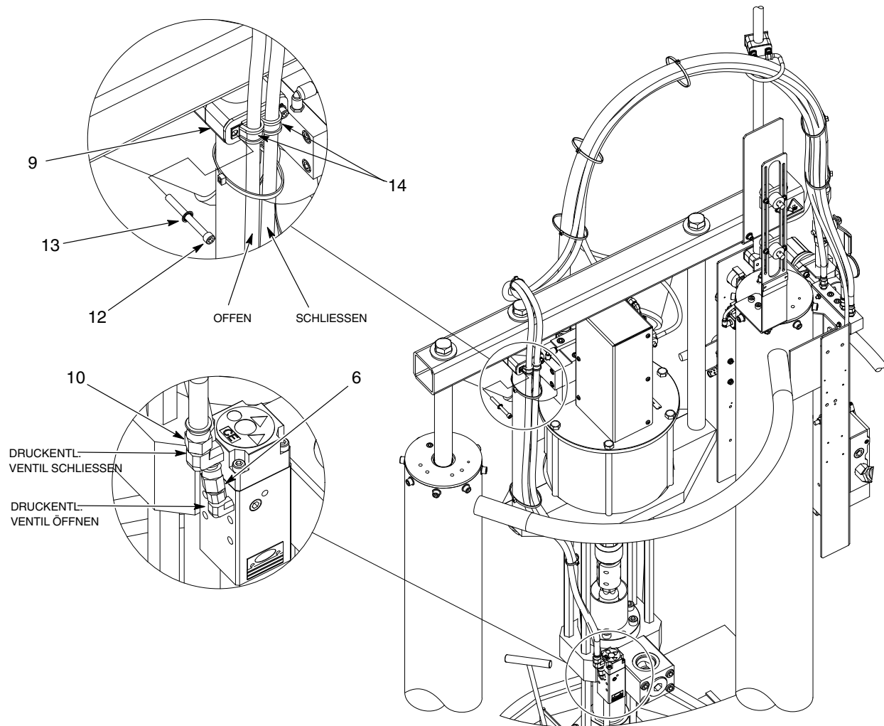
Abb. 14 Schwarzer Schlauch für großen Rahmen mit 55 Gallonen (Forts.)
