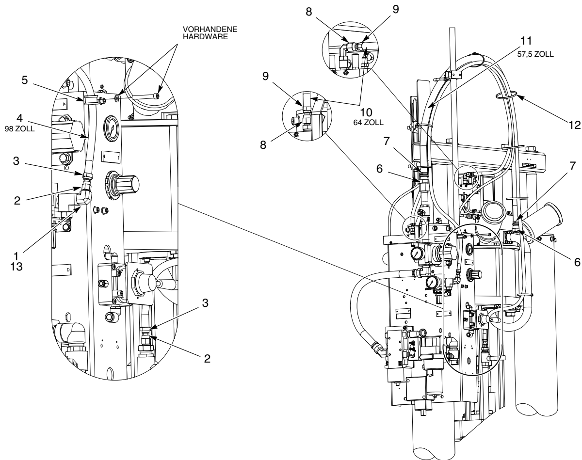
Abb. 12 Schwarzer Schlauch für großen Rahmen mit 55 Gallonen
