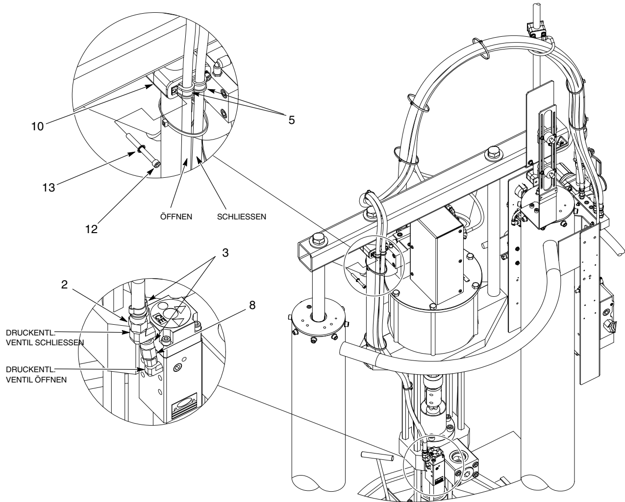
Abb. 9 Schwarzer Schlauch für großen Rahmen mit 5/30 Gallonen mit Druckentlastung (Forts.)
