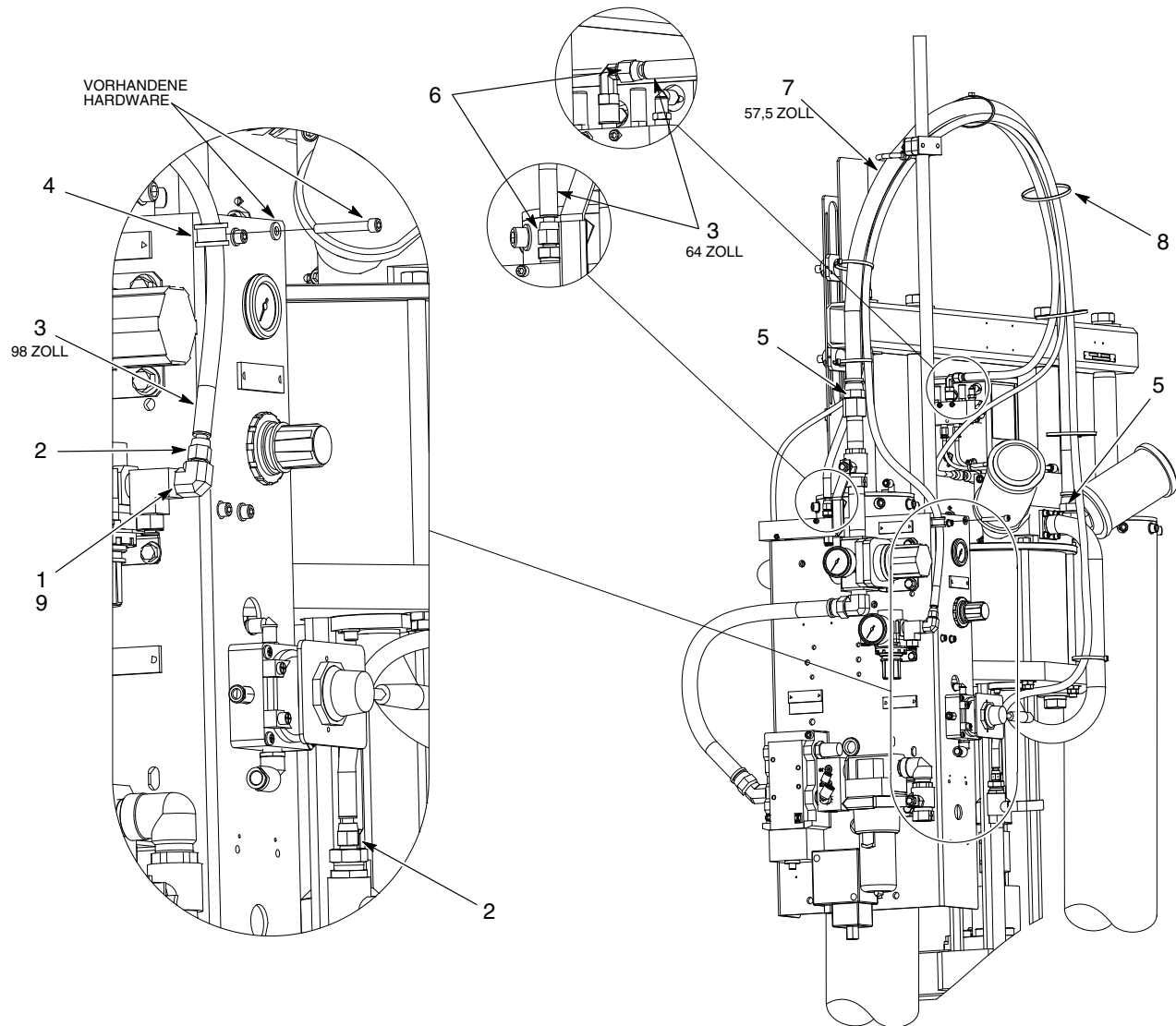
Abb. 4 Feuerbeständiger Schlauch für großen Rahmen mit 5/30 Gallonen
