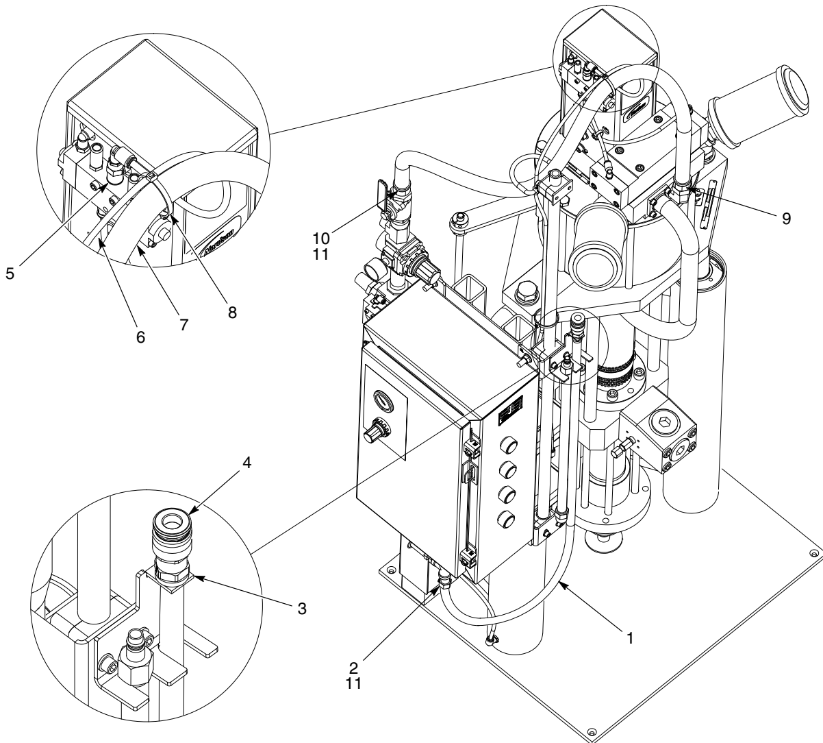
Abb. 18 CE-Schlauch für Rhino VE mit kleinem Rahmen
