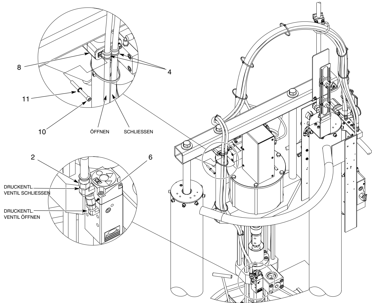
Abb. 7 Feuerbeständiger Schlauch für großen Rahmen mit 5/30 Gallonen mit Druckentlastung (Forts.)
