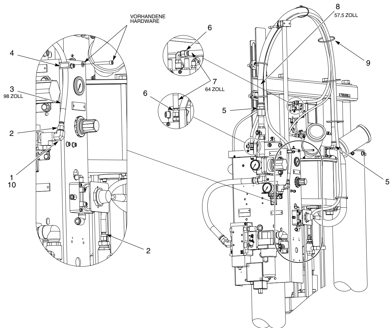
Abb. 10 Feuerbeständiger Schlauch für großen Rahmen mit 55 Gallonen
