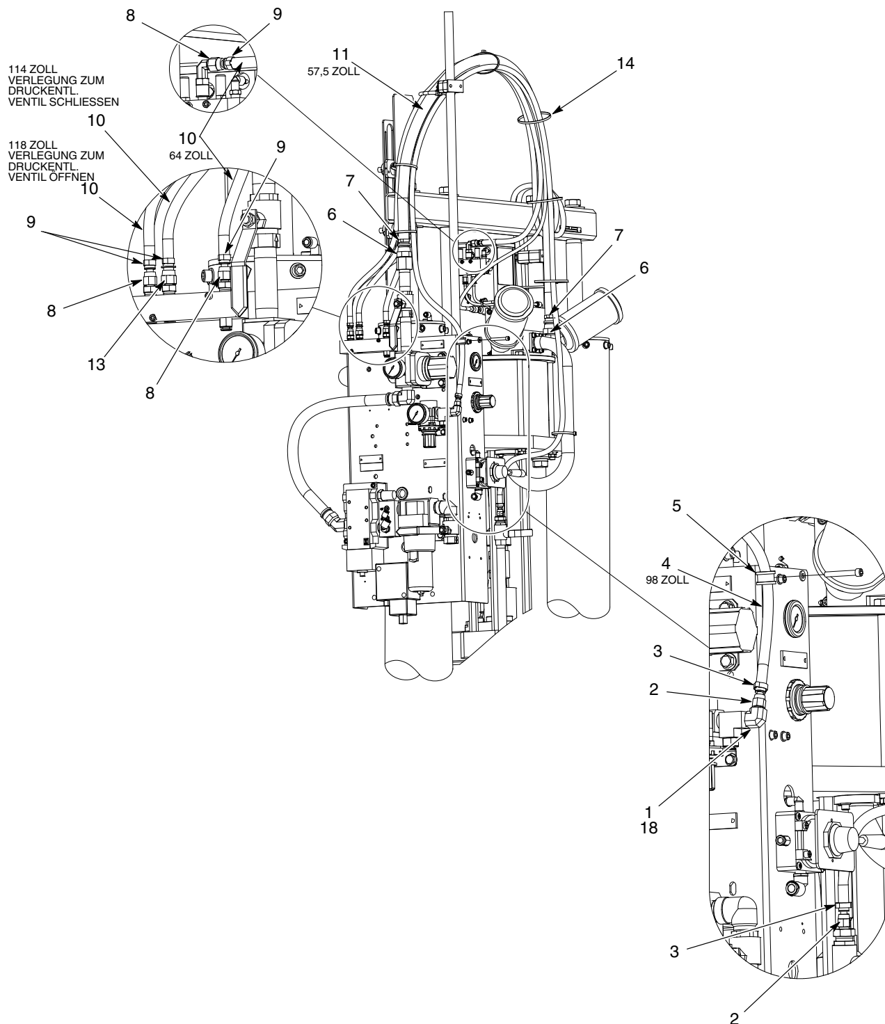
Abb. 15 Schwarzer Schlauch für großen Rahmen mit 55 Gallonen mit Druckentlastung
