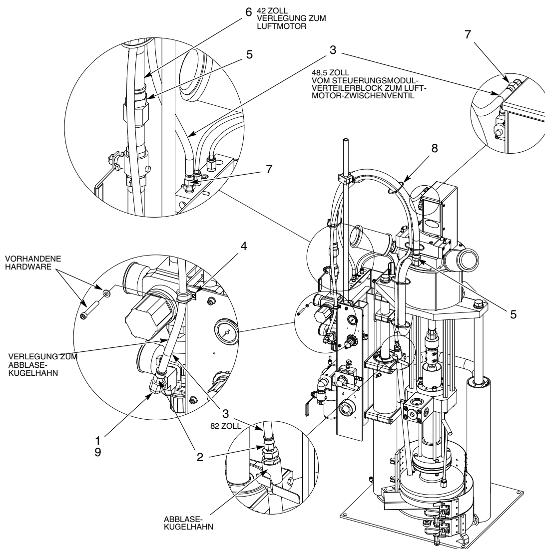
Abb. 2 Feuerbeständiges Verbindungsschlauchmodul für kleinen Rahmen
