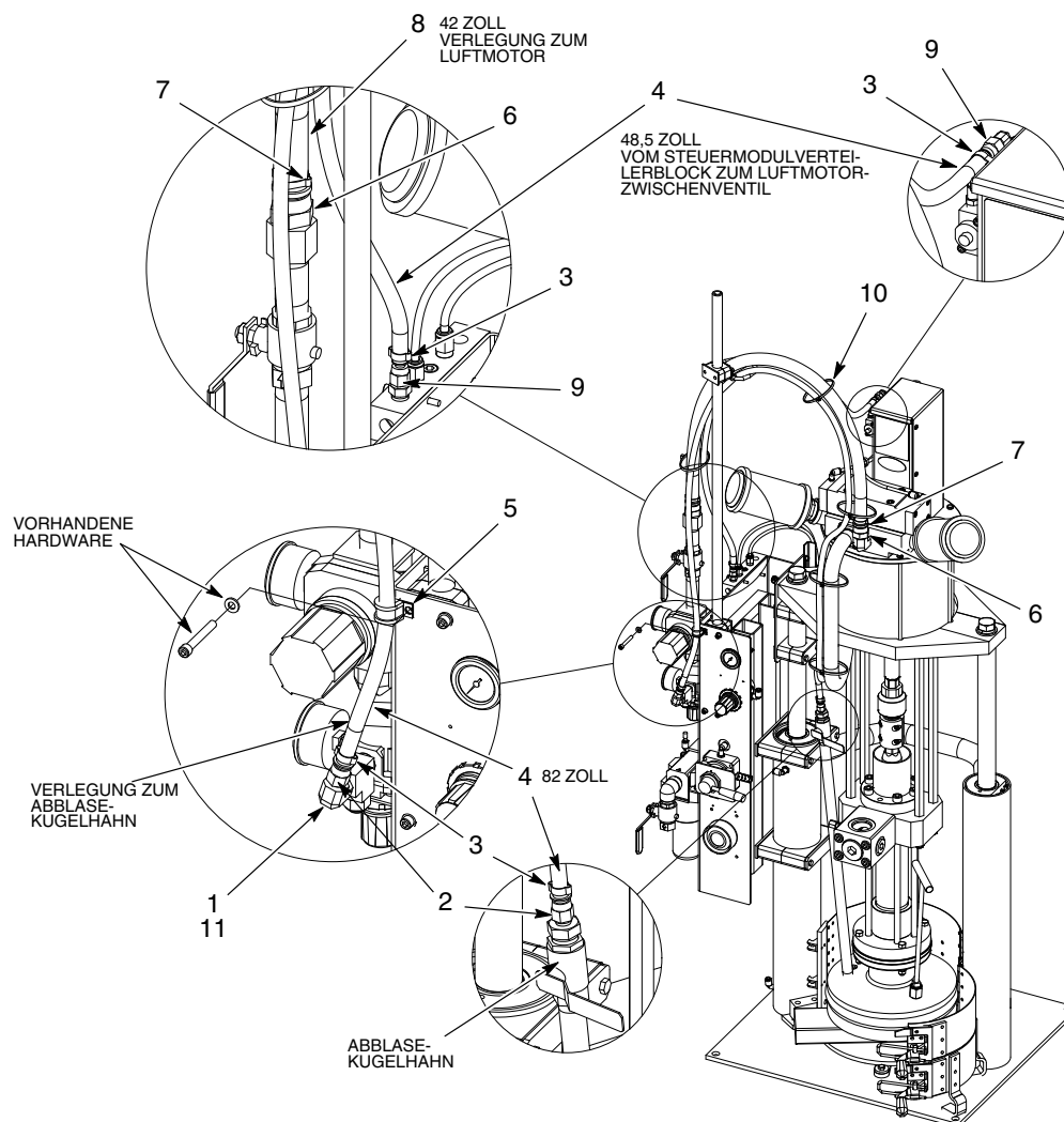
Abb. 3 Schwarzer Schlauch für kleinen Rahmen
