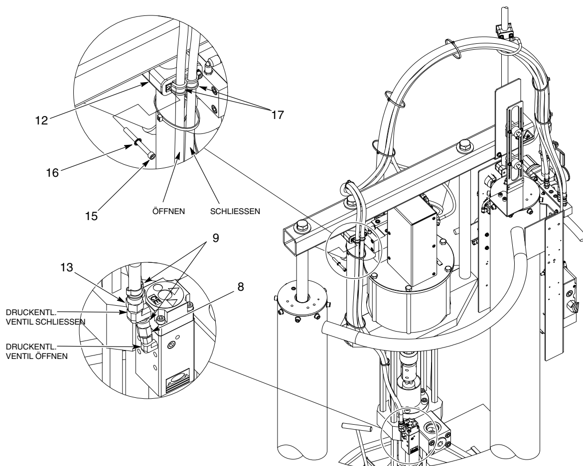
Abb. 16 Schwarzer Schlauch für großen Rahmen mit 55 Gallonen mit Druckentlastung (Forts.)
