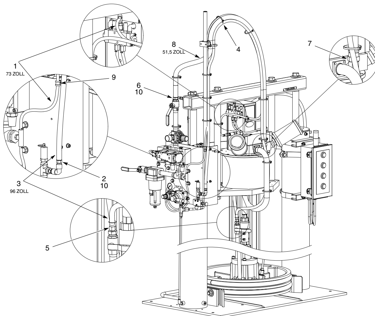
Abb. 11 Grüner feuerbeständiger Schlauch für großen Rahmen mit 55 Gallonen
