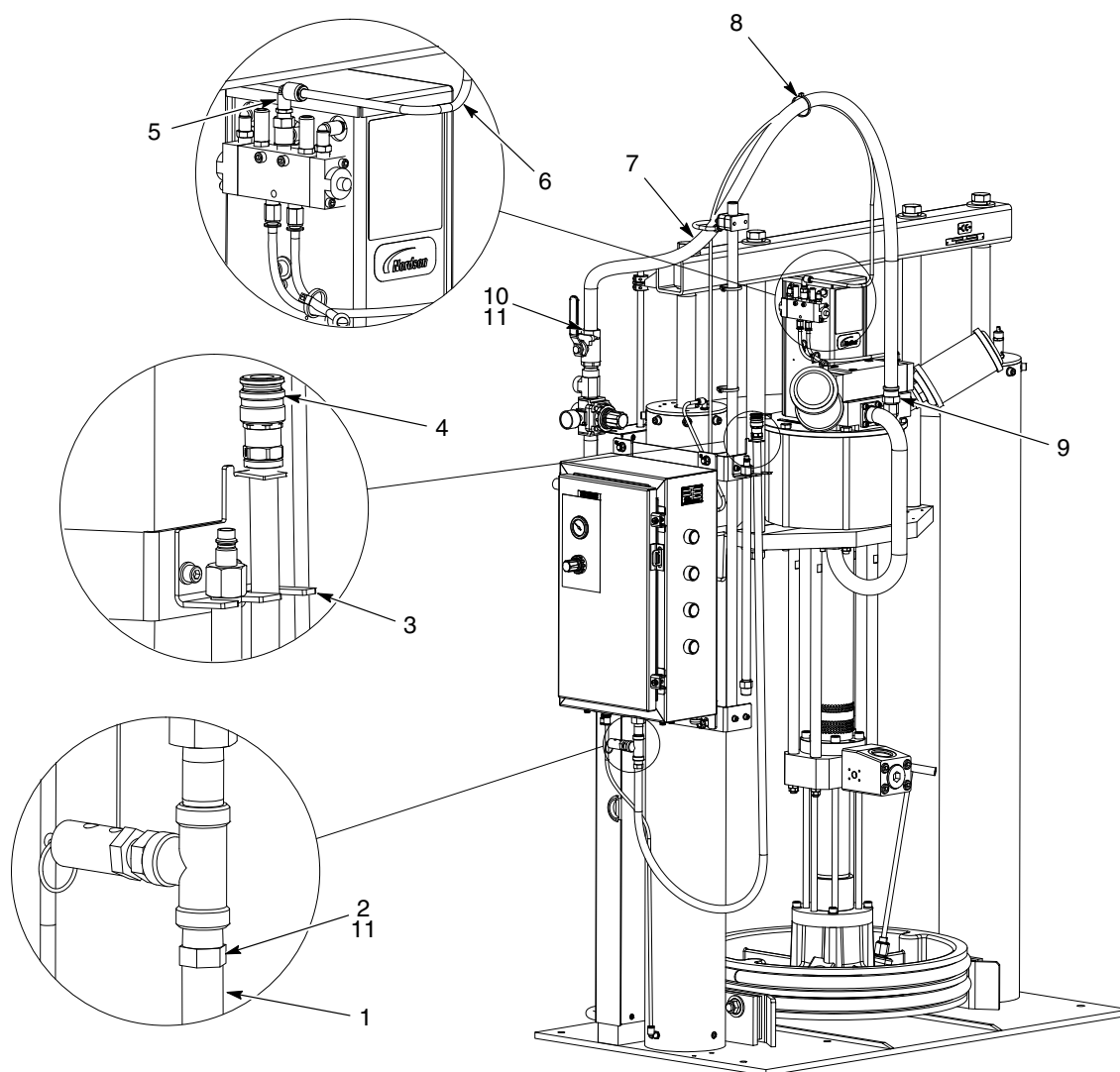
Abb. 20 CE-Schlauch für Rhino VE mit großem Rahmen
