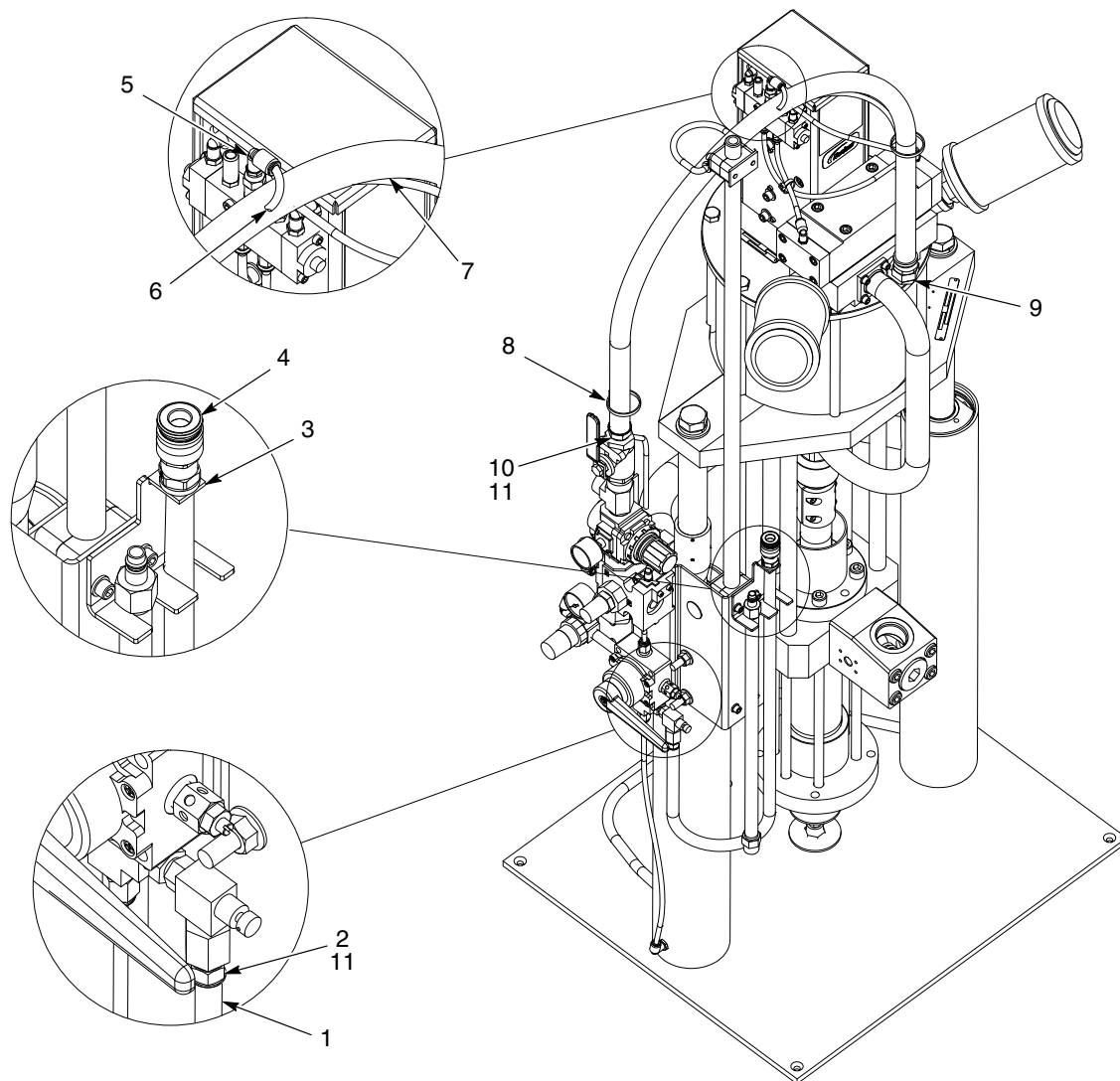
Abb. 17 Schlauch für Rhino VE mit kleinem Rahmen
