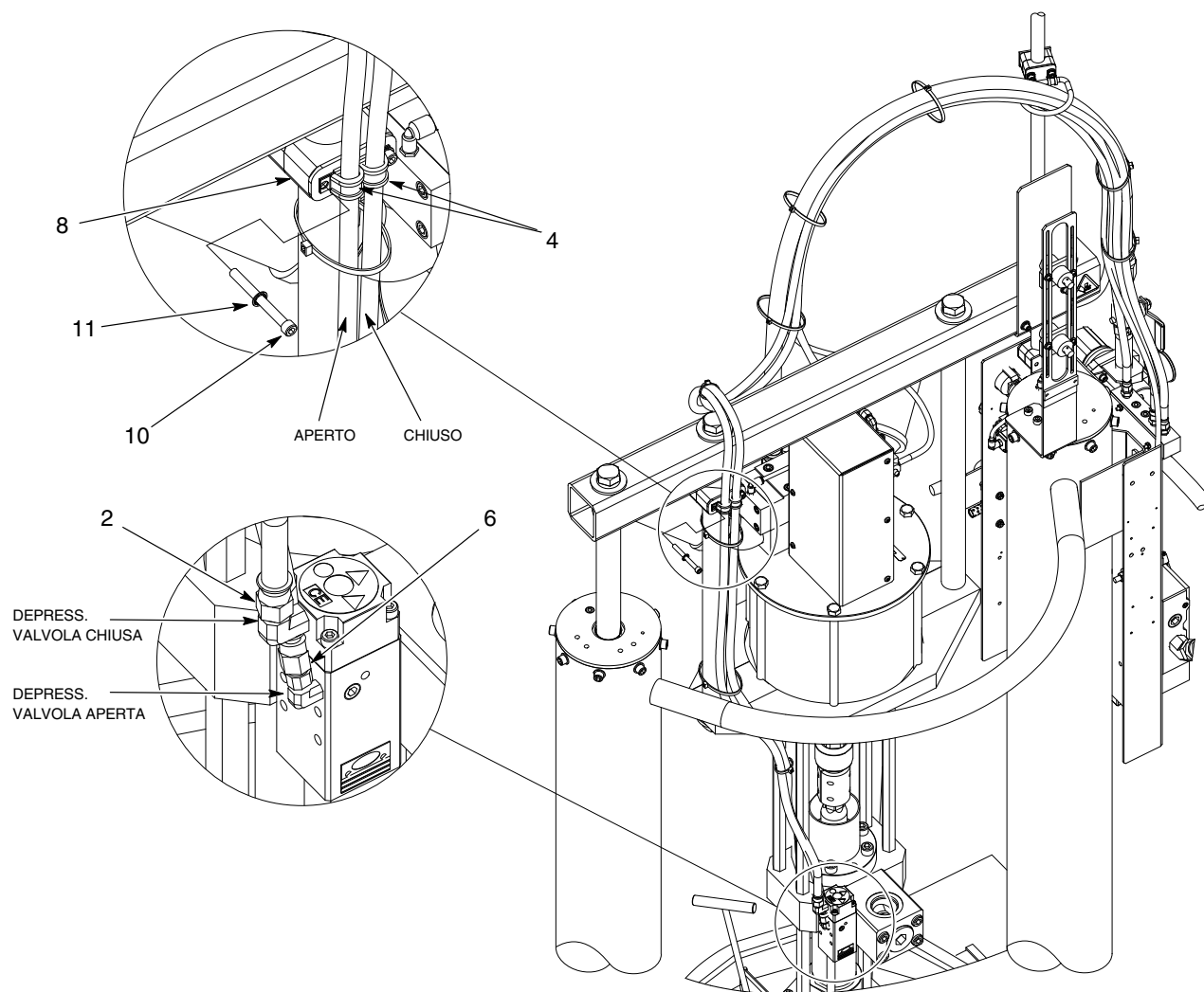
Figura 7 Tubo resistente al fuoco con telaio grande da 5/30 galloni con depressurizzazione (segue)
