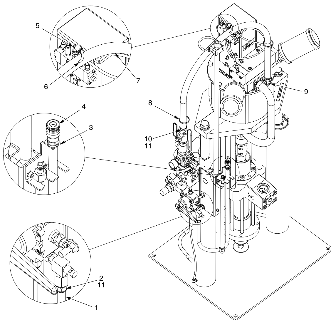
Figura 17 Tubo con telaio piccolo VE Rhino
