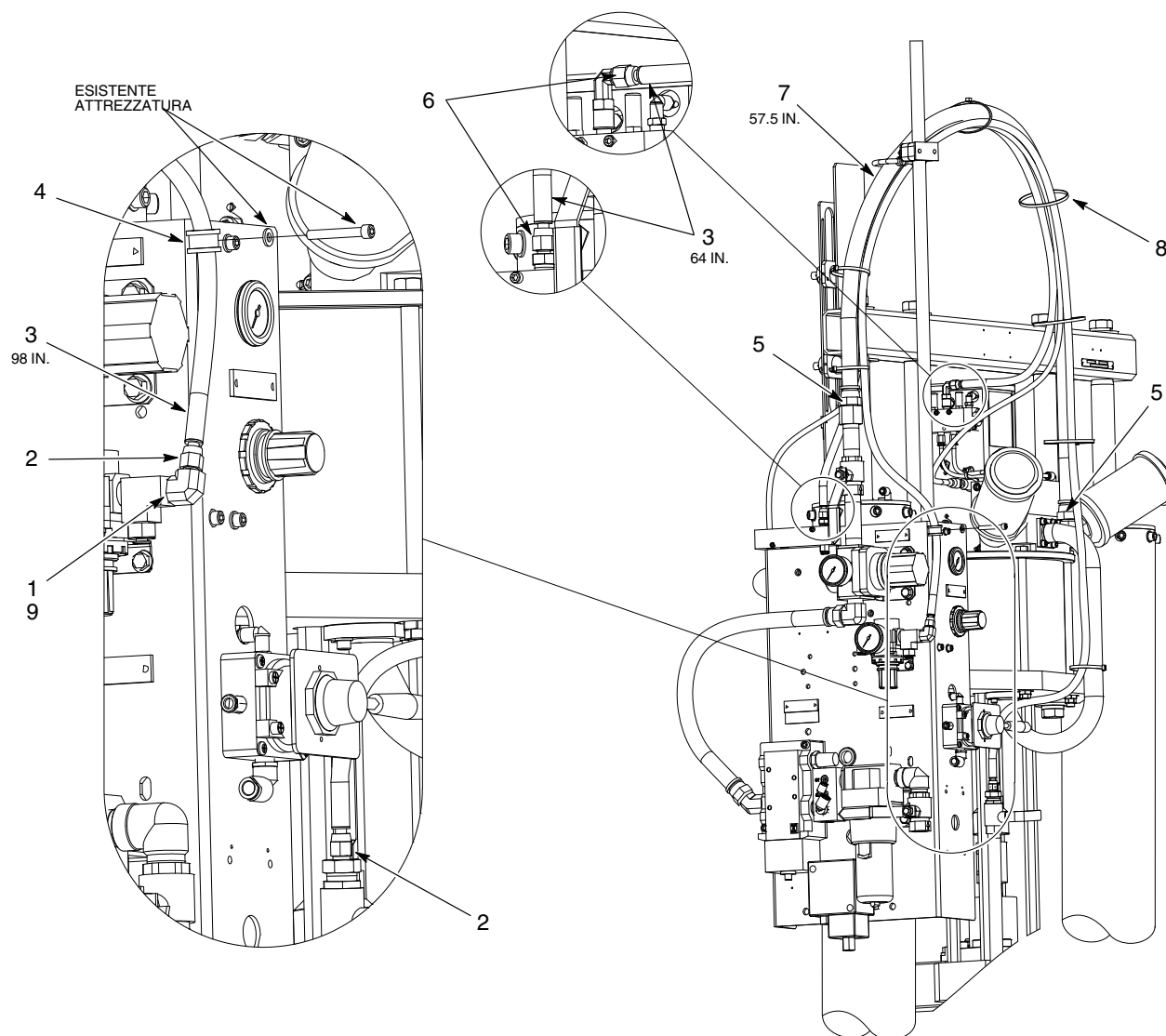
Figura 4 Tubo resistente al fuoco con telaio grande da 5/30 galloni
