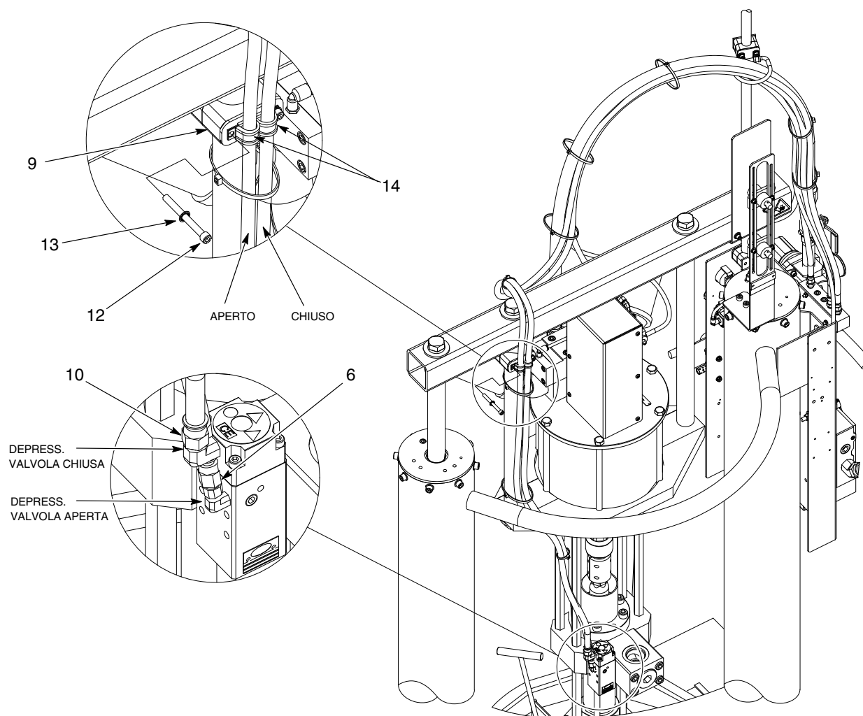
Figura 14 Tubo nero con telaio grande da 55 galloni (segue)
