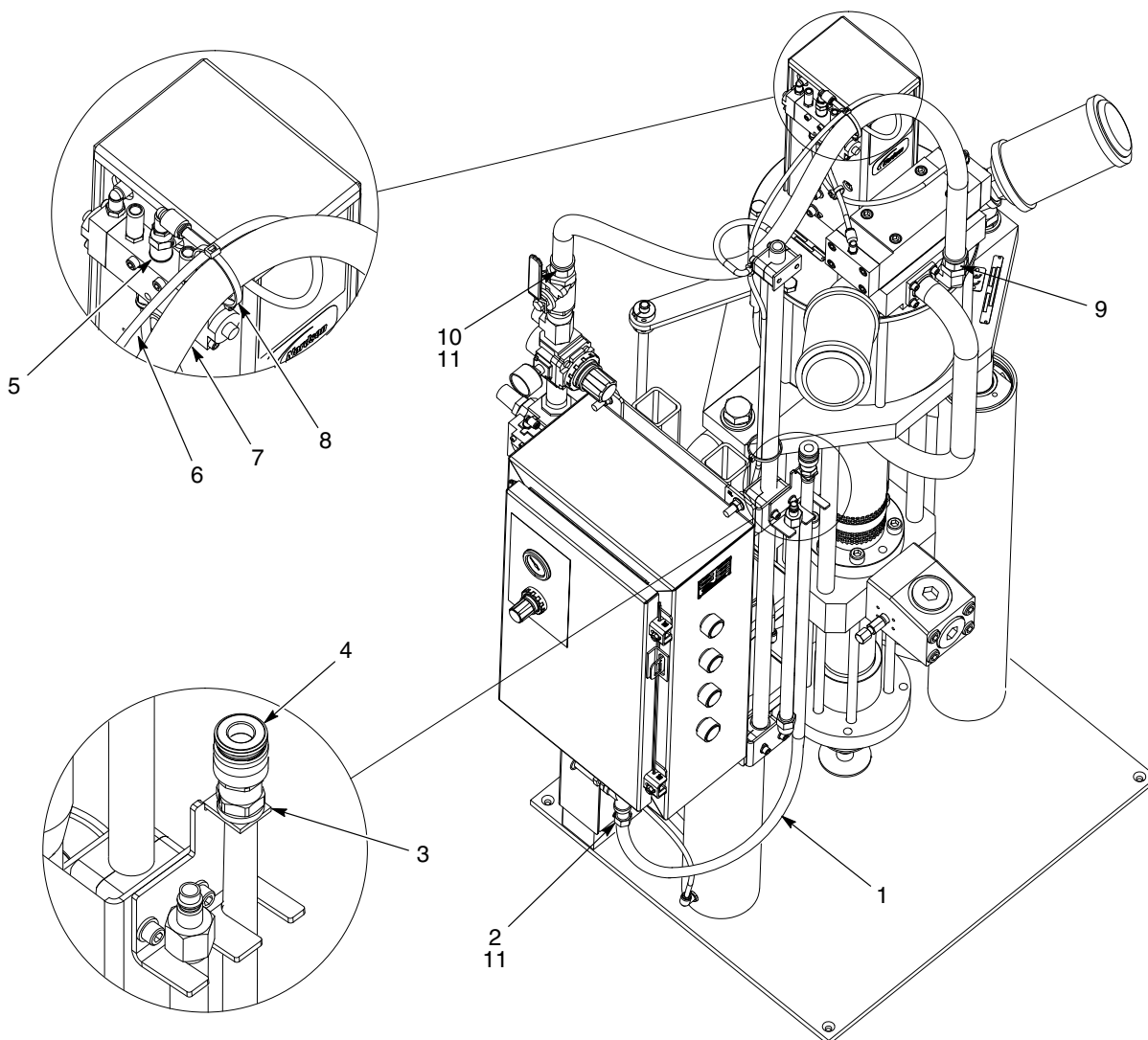
Figura 18 Tubo CE con telaio piccolo VE Rhino
