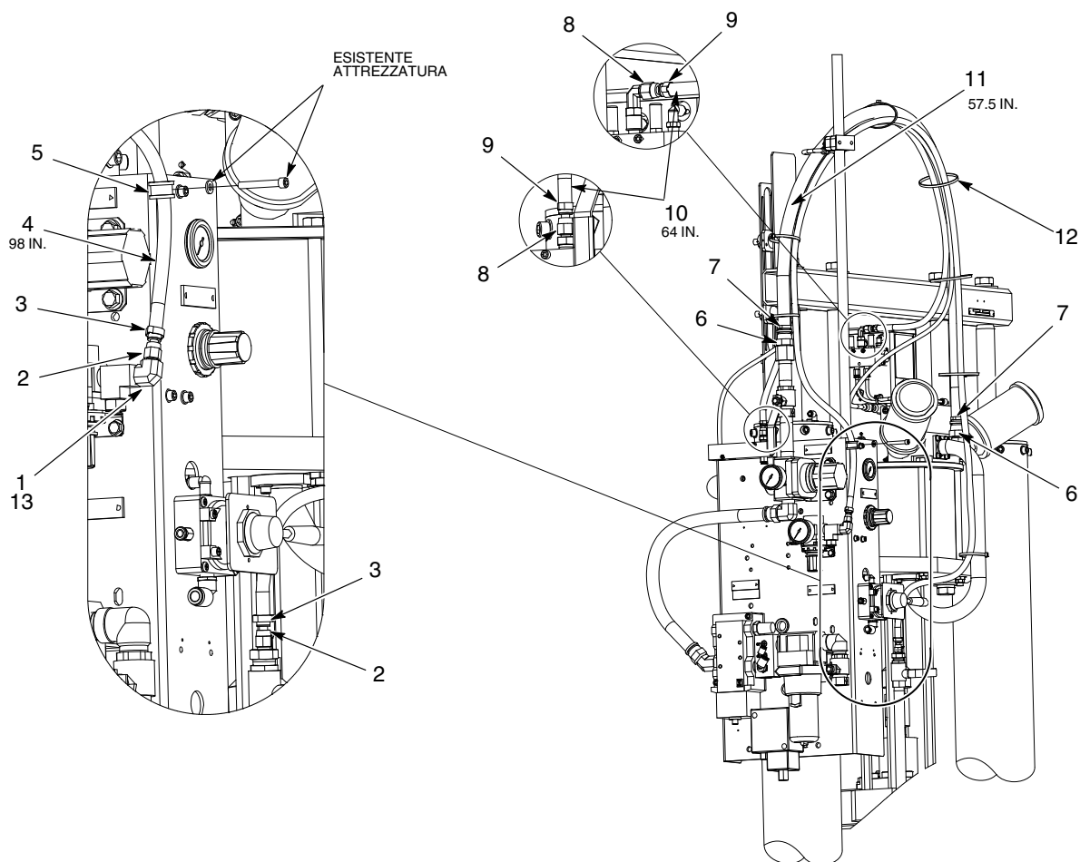
Figura 12 Tubo nero con telaio grande da 55 galloni
