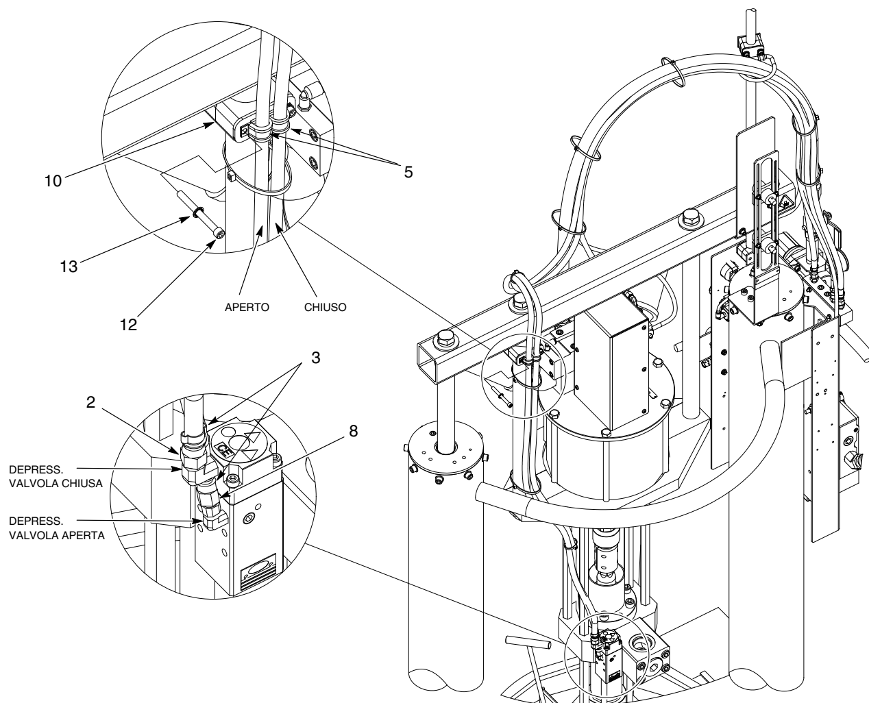
Figura 9 Tubo nero con telaio grande da 5/30 galloni con depressurizzazione (segue)
