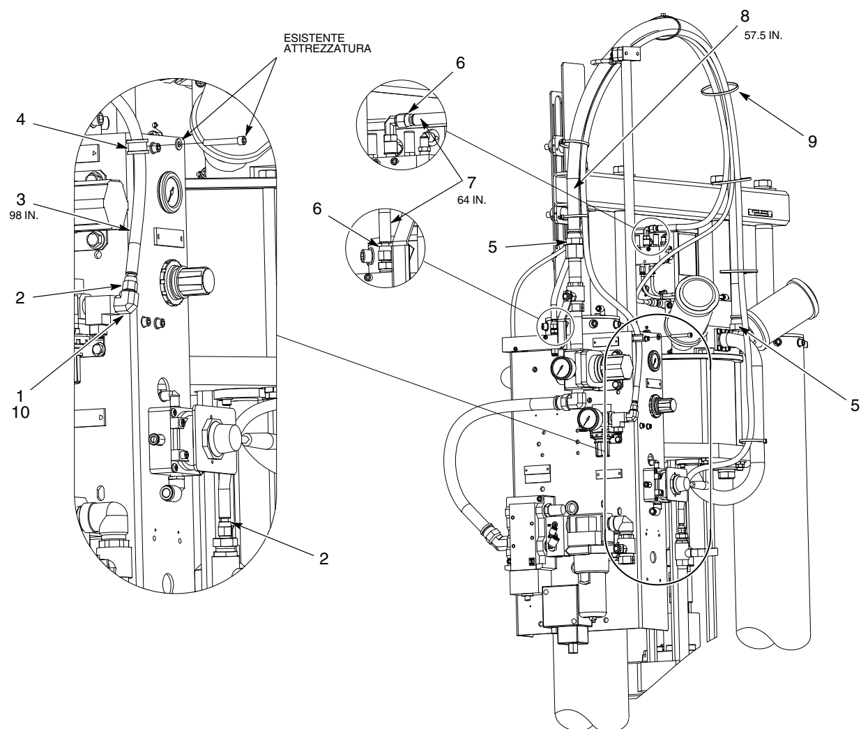
Figura 10 Tubo resistente al fuoco con telaio grande da 55 galloni
