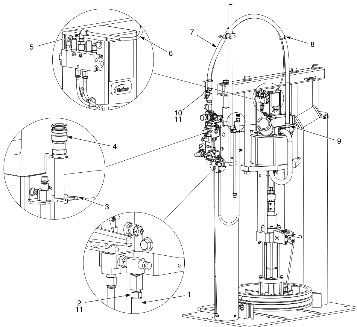
Figura 19 Tubo CE con telaio grande VE Rhino
