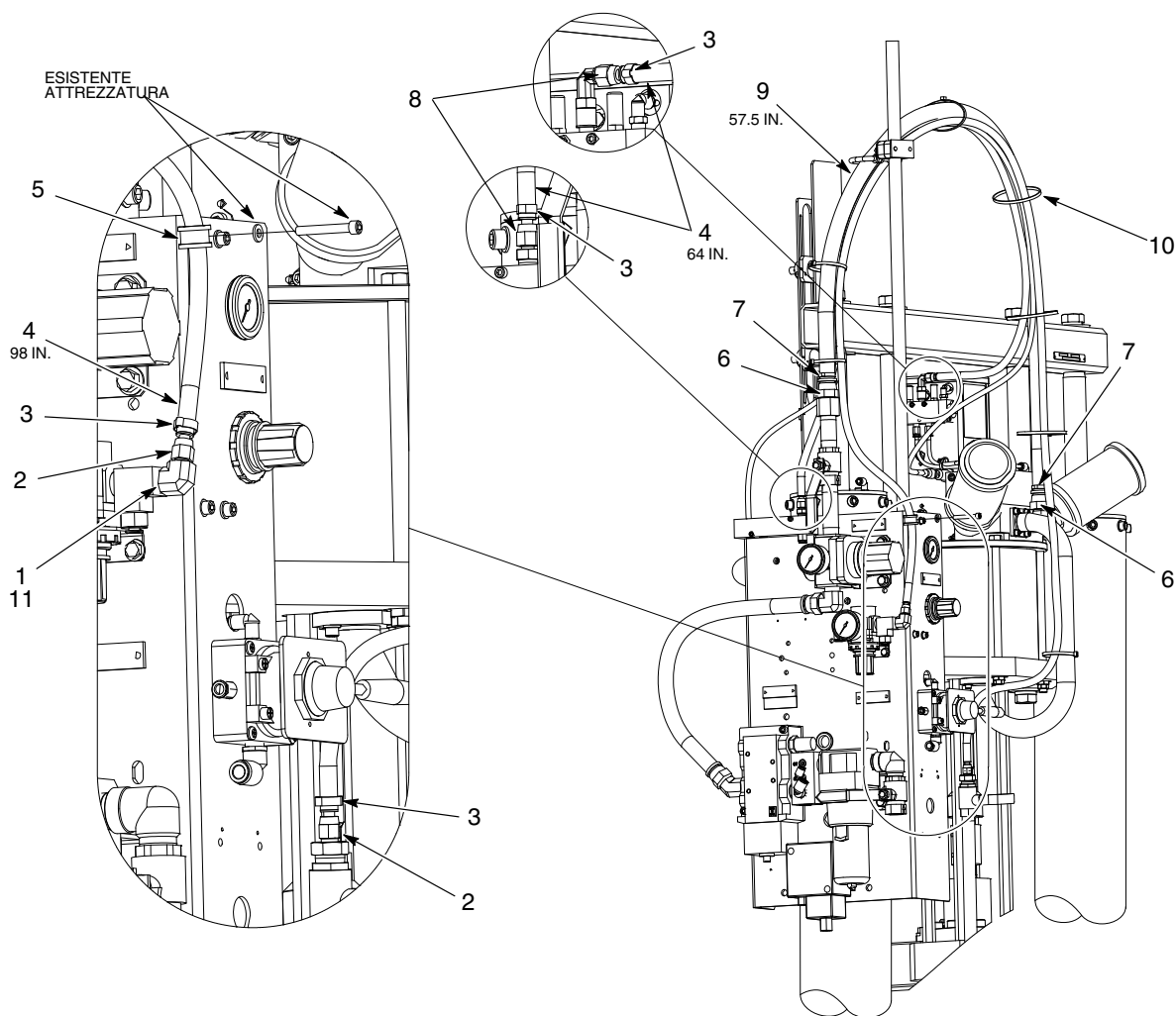
Figura 5 Tubo nero con telaio grande da 5/30 galloni
