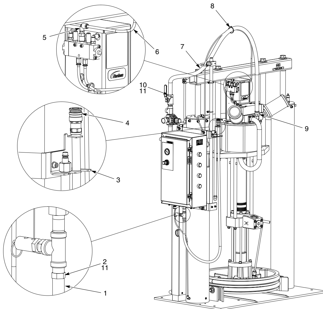
Figura 20 Tubo CE con telaio grande VE Rhino
