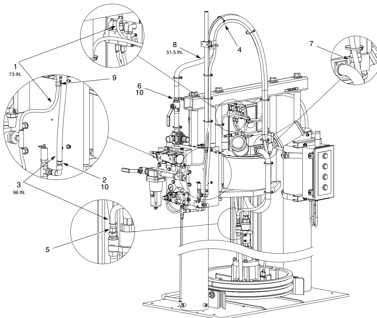
Figura 11 Tubo resistente al fuoco verde con telaio grande da 55 galloni
