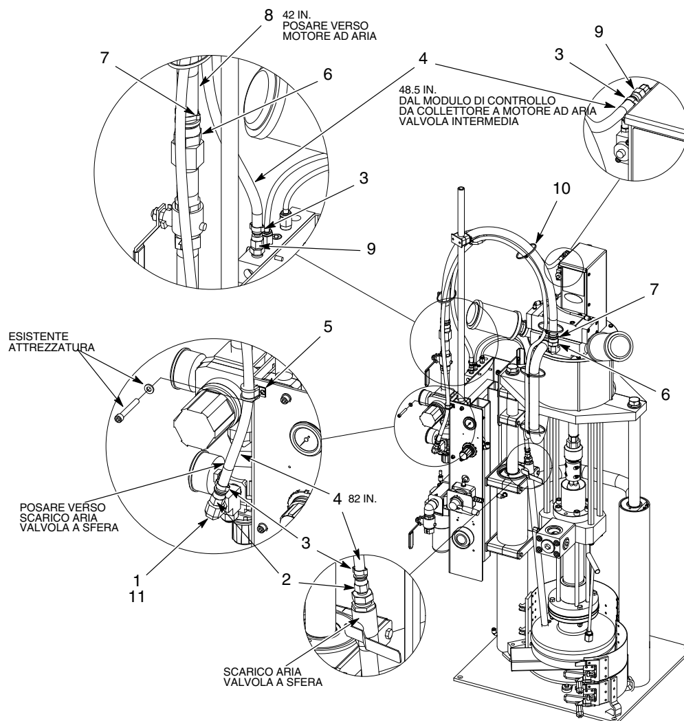
Figura 3 Tubo nero con telaio piccolo
