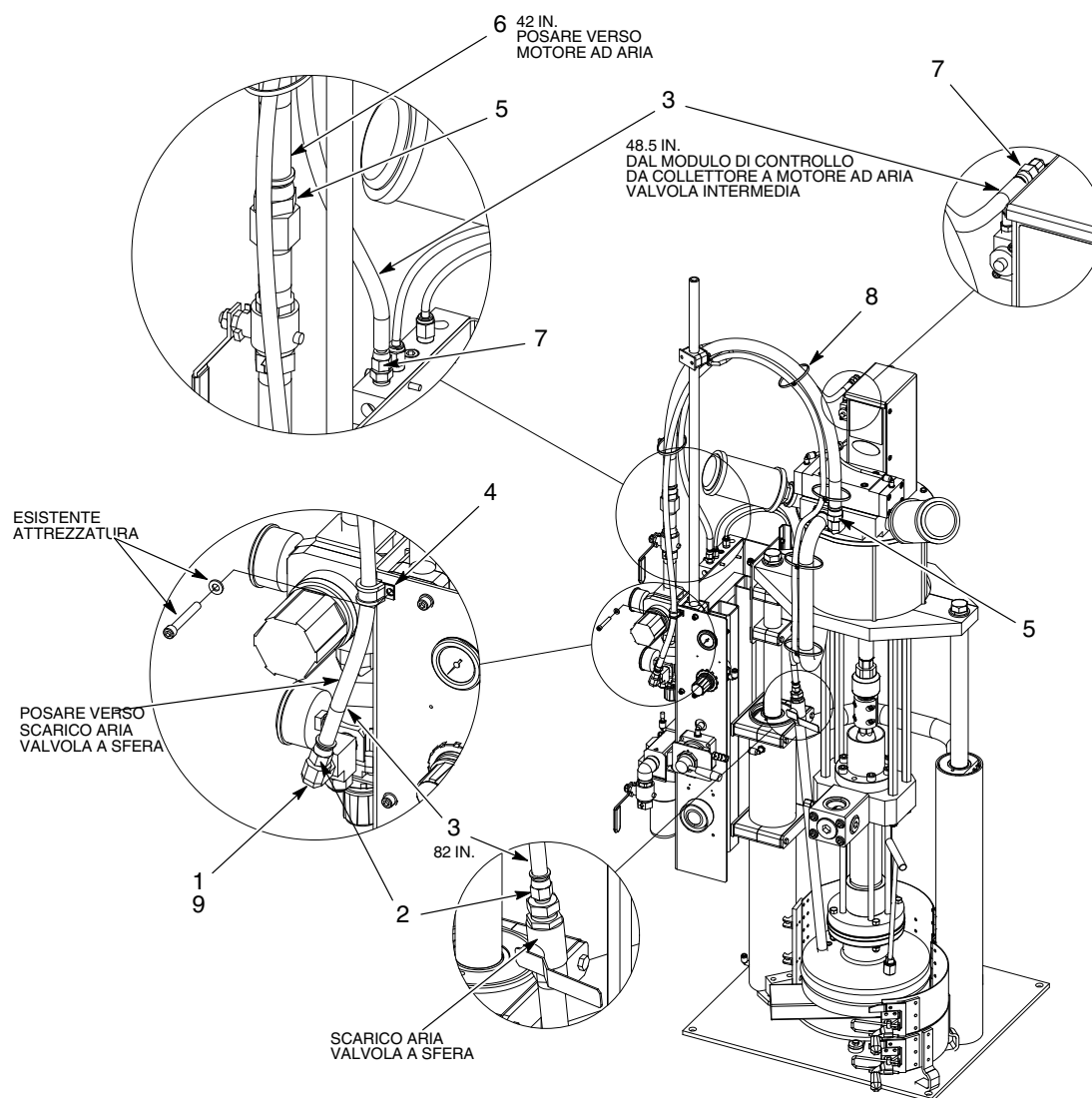
Figura 2 Modulo del tubo di intercollegamento resistente al fuoco con telaio piccolo
