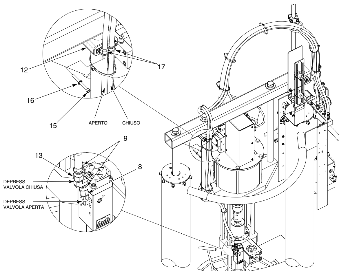
Figura 16 Tubo nero con telaio grande da 55 galloni con depressurizzazione (segue)
