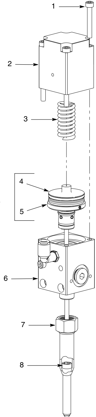
Yayı Kapalı Bağımsız Dağıtım Valfi
