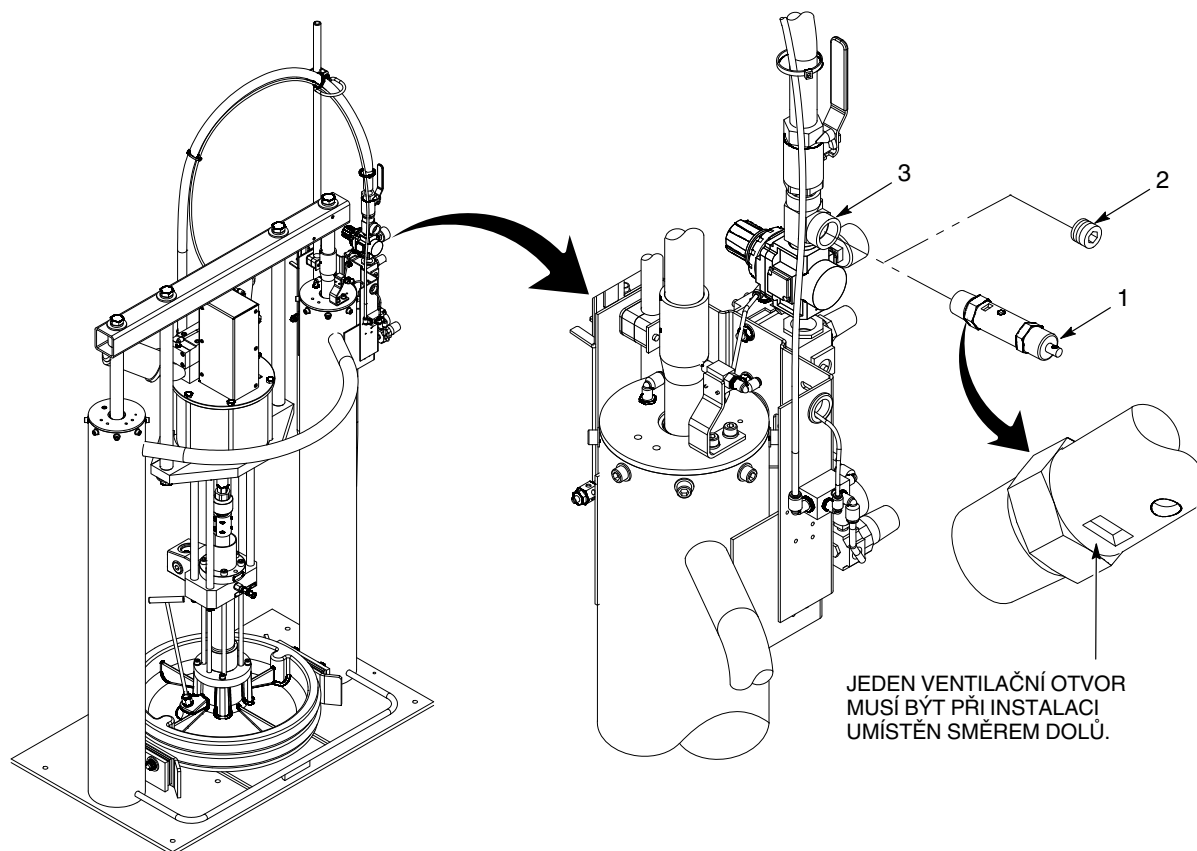
Obr. 1 Typické instalace
